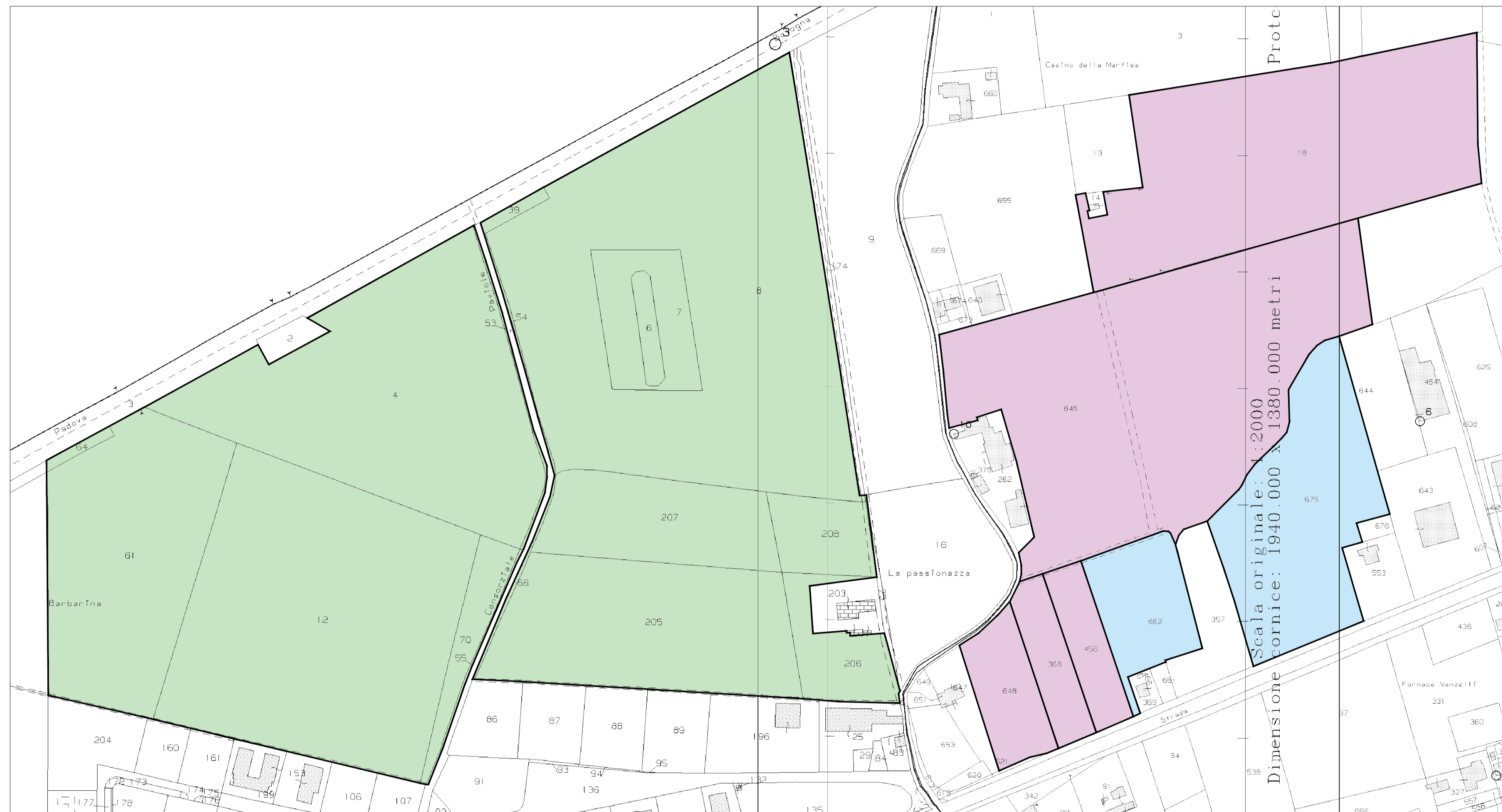
PARTICELLE CATASTALI OCCUPATE DA IMPIANTO FOTOVOLTAICO - Scala 1:2500
