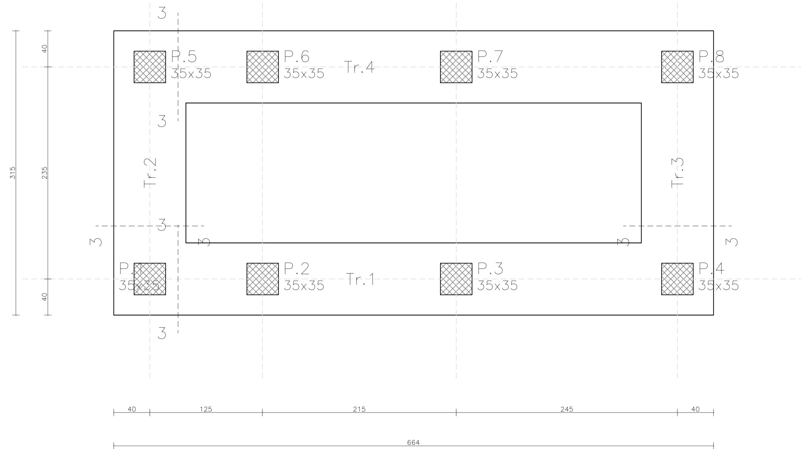
Pianta a quota -40,0
