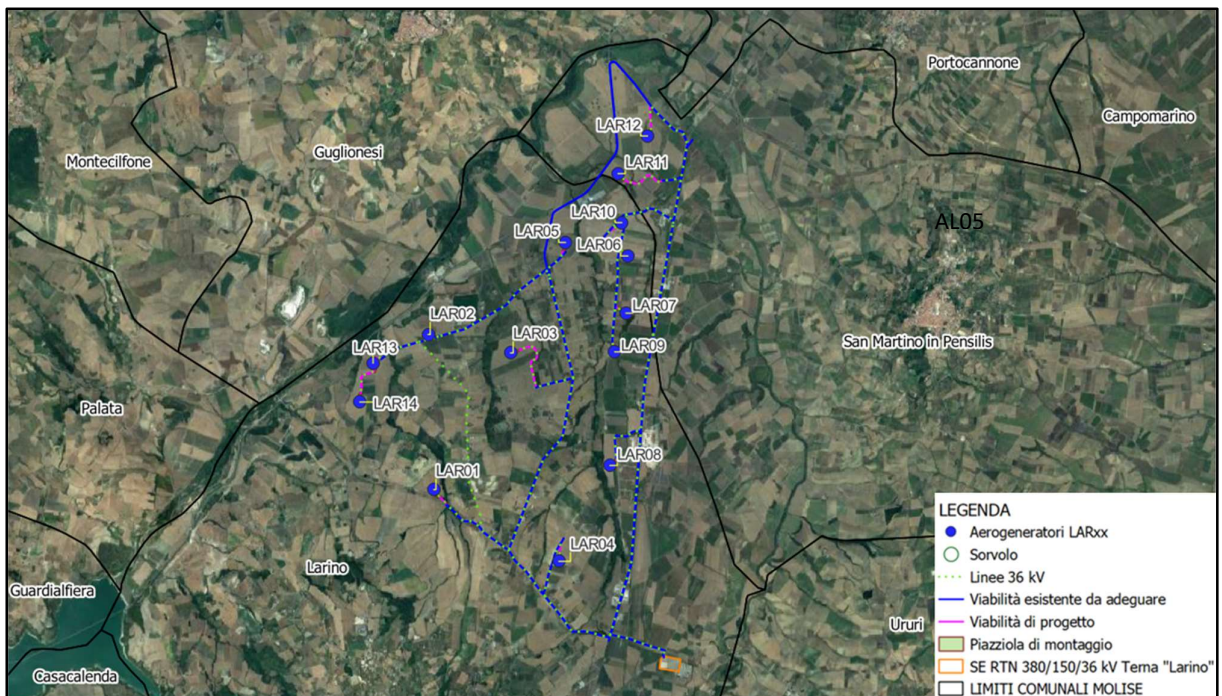
Figura 6.2: Layout d'impianto su immagine satellitare
