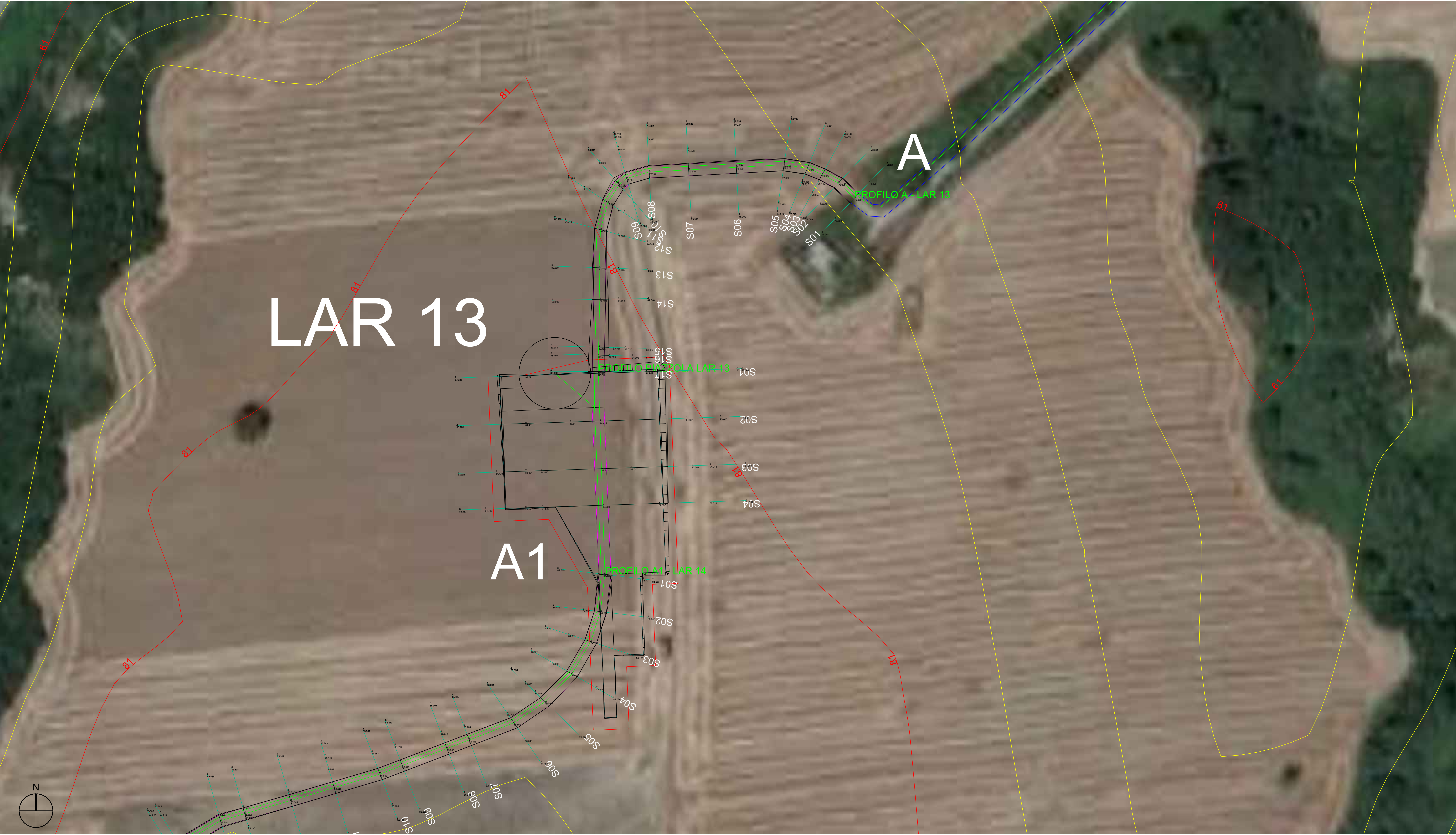
PLANIMETRIA LAR13 SU CURVE DI LIVELLO_ SCALA 1:1.000
