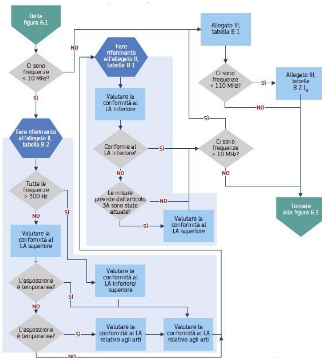
Figura 3. Rappresentazione schematica che illustra la relazione tra i valori limite di esposizione e i livelli di azione.
