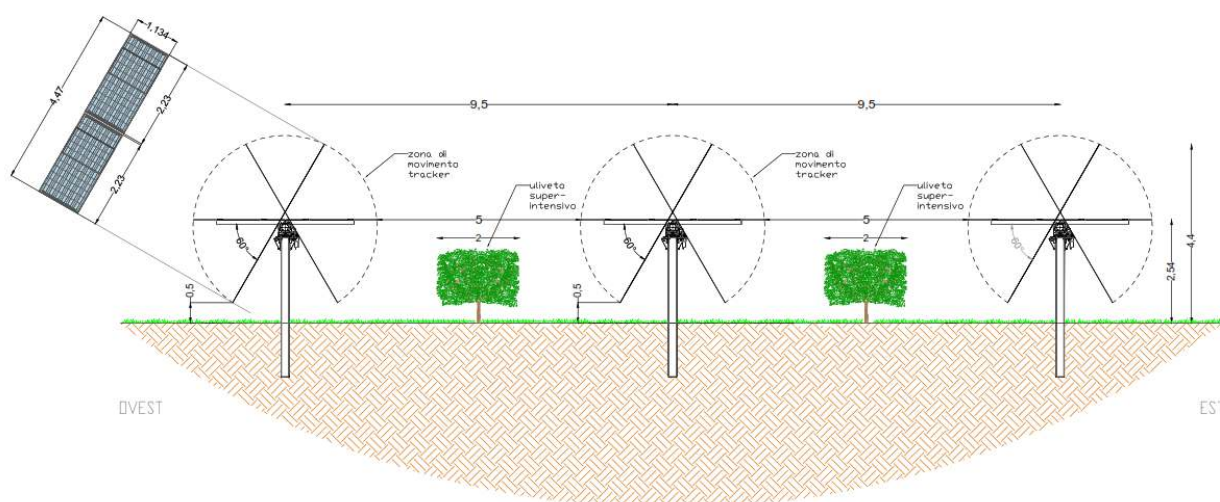
Fig. 17 Pitch dei tracker
