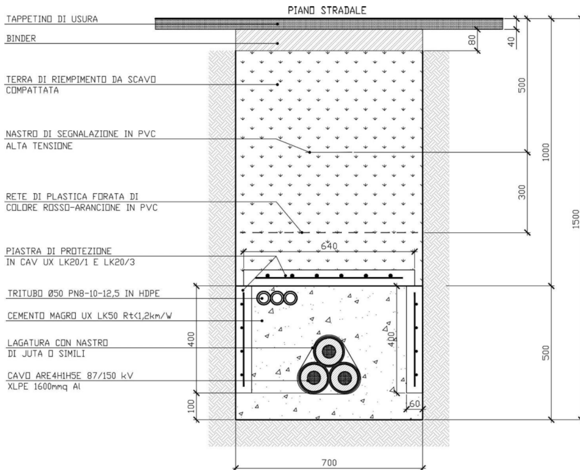
Fig. 19 – Sezione di posa a trifoglio sotto strada
