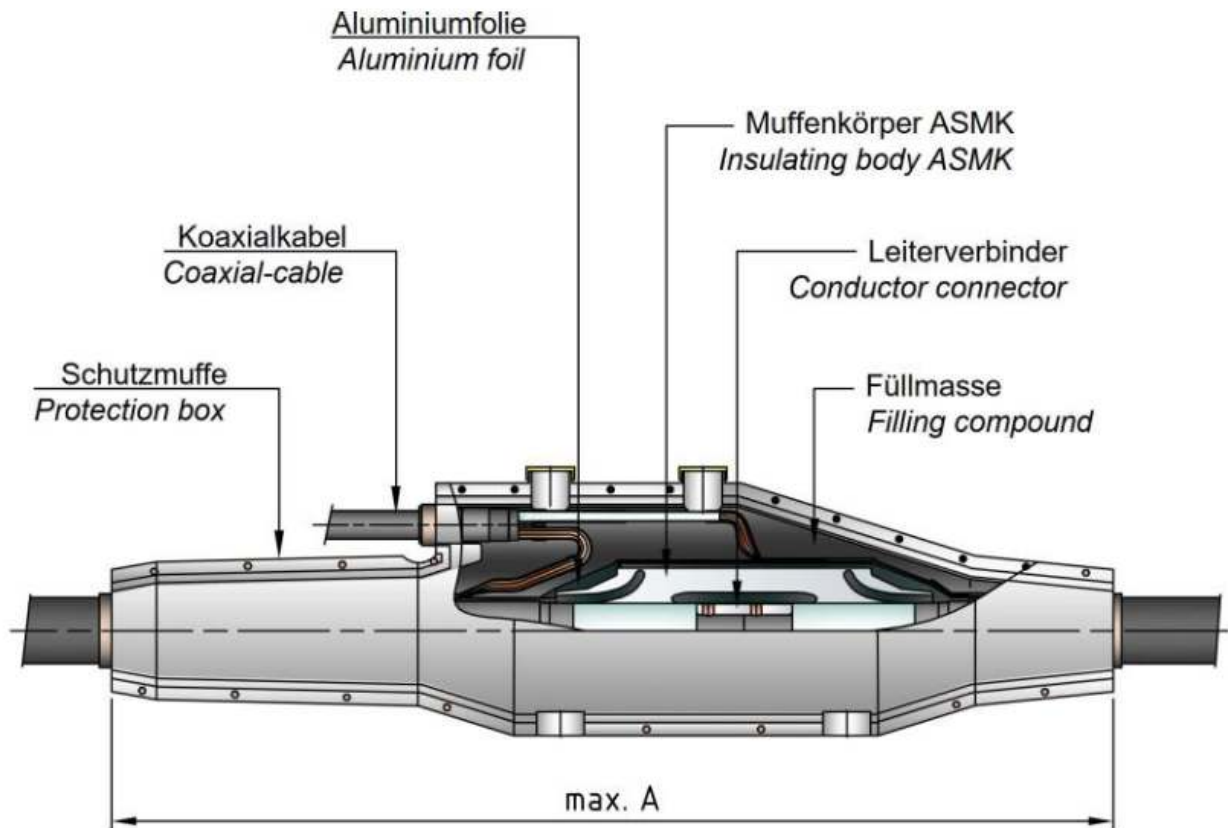
Fig. 20 – Tipico giunto per cavo AT
