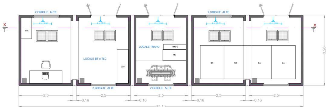
Fig. 17 Cabina di servizio
