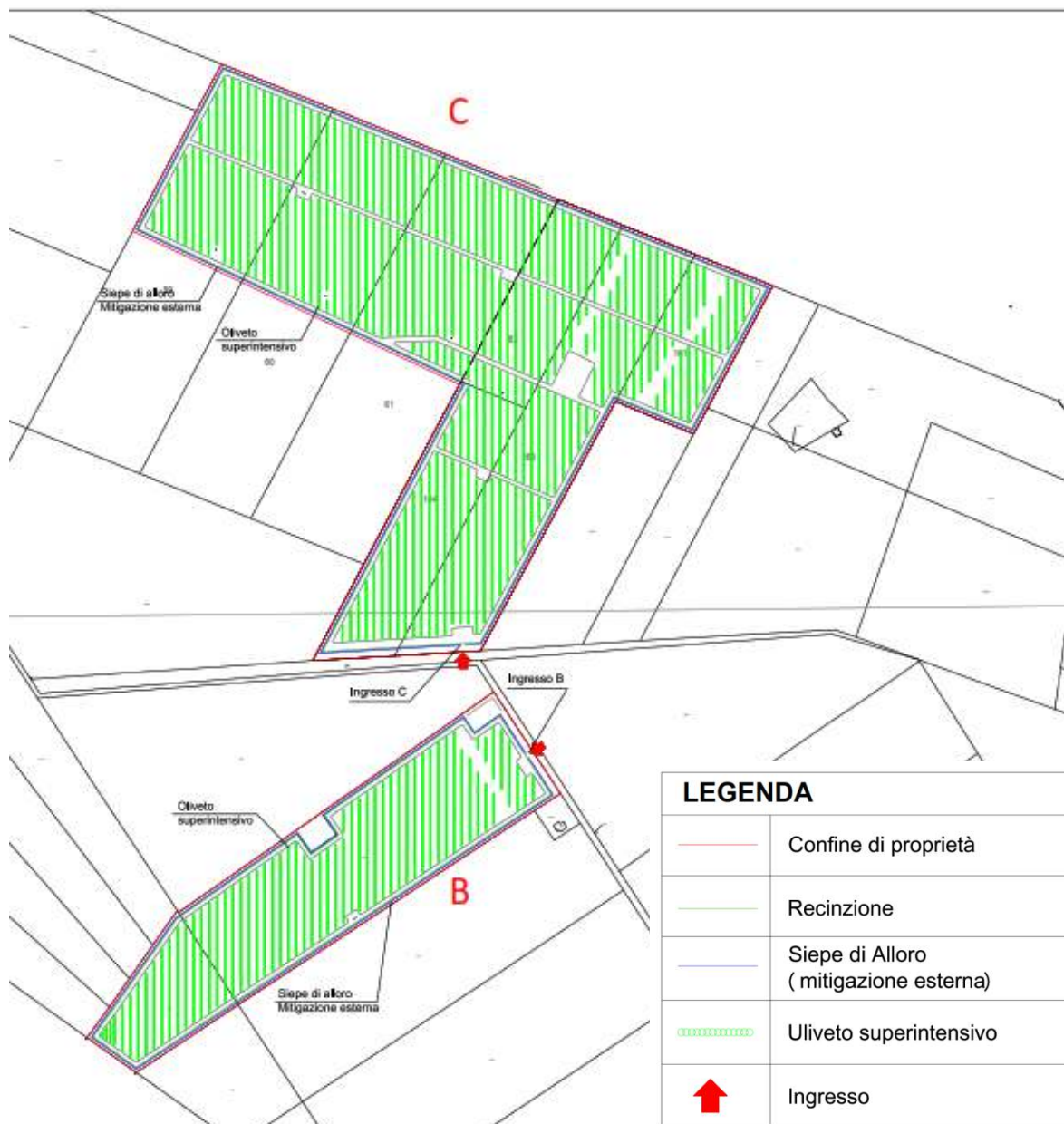
Fig. 8 Blocchi "B" e "C" su stralcio catastale
