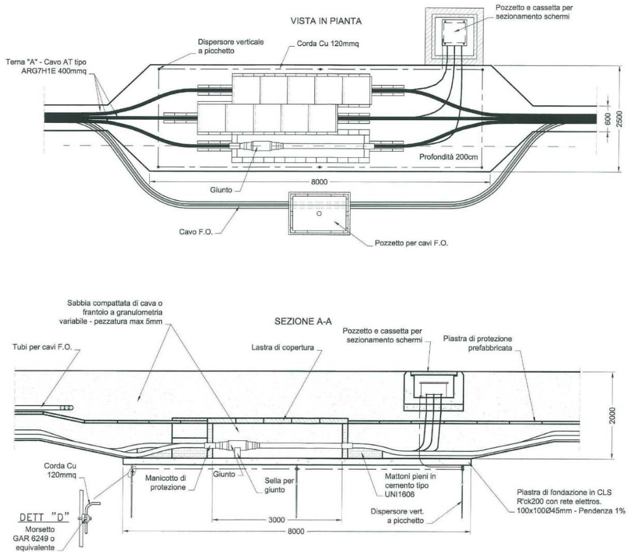
Fig.21 – Tipica buca giunti
