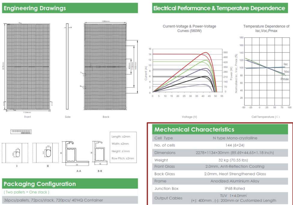
Fig. 12 Data Sheet Modulo Fotovoltaico _1
