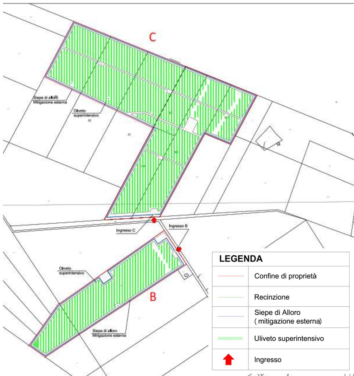
Fig. 3 Impianto agrivoltaico blocco "B" e "C" - aree destinate all'agricoltura e misure mitigative
