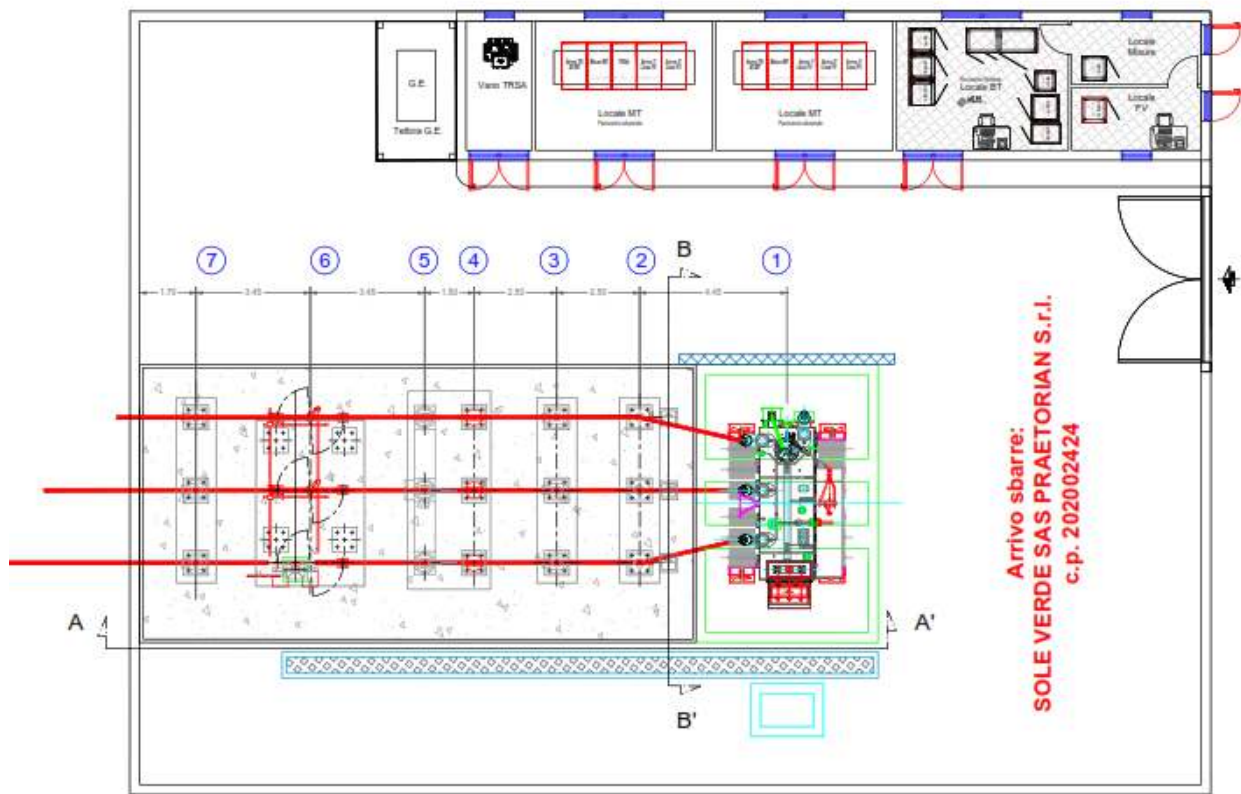
Fig. 11 Planimetria sottostazione utente
