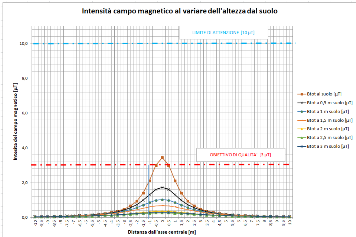
Fig. n°4 Intensità del campo magnetico al variare dell'altezza dal suolo del tratto L05-L06 di cavidotto
