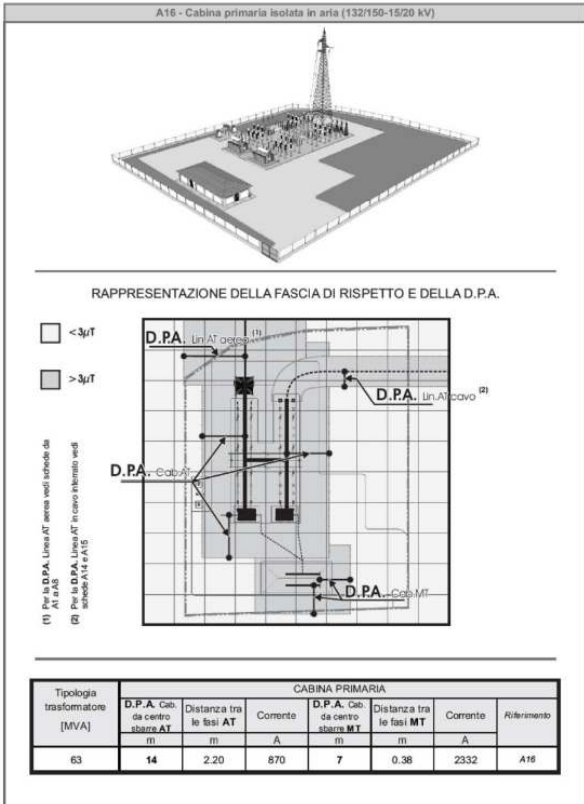
Fig. 9 Fasce di rispetto relative ad una cabina primaria di Enel
