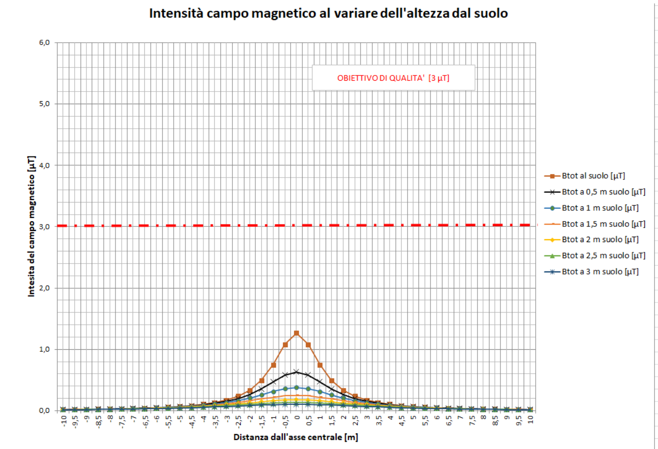
Fig. n°3 Intensità del campo magnetico al variare dell'altezza dal suolo del tratto L05 di cavidotto
