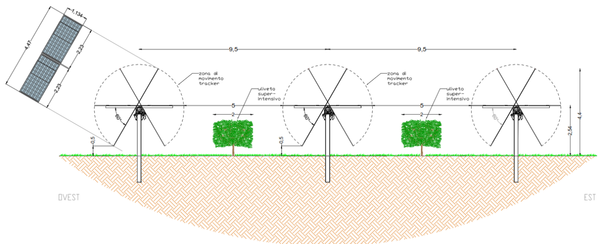
Figura 4-4: Schema d'impianto dell'ulivo super intensivo tra i pannelli fotovoltaico – vista in sezione
