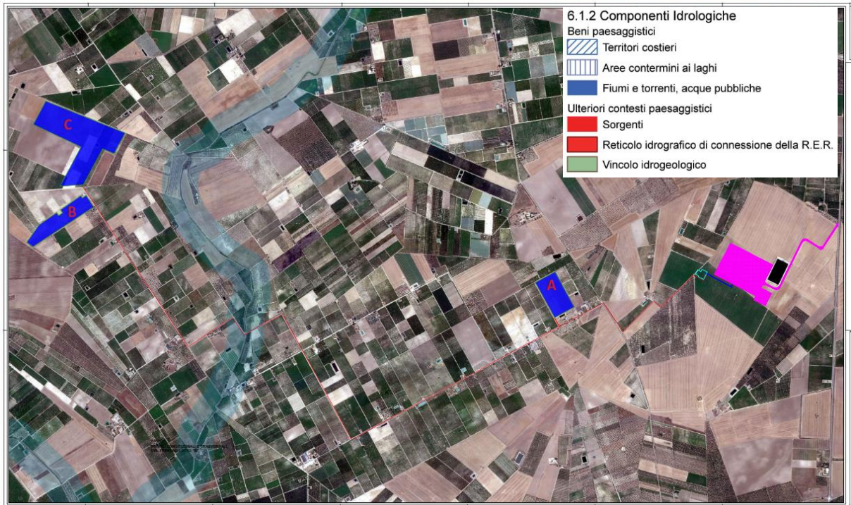
Figura 5-2: Struttura Idrogeomorfologica – fonte PPTR
