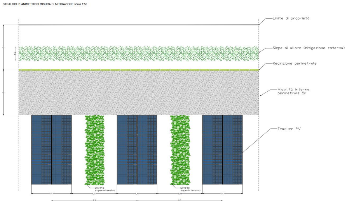
Figura 2-6: Esempio di sistemazione dell'oliveto super intensivo all'interno dell'impianto fotovoltaico
