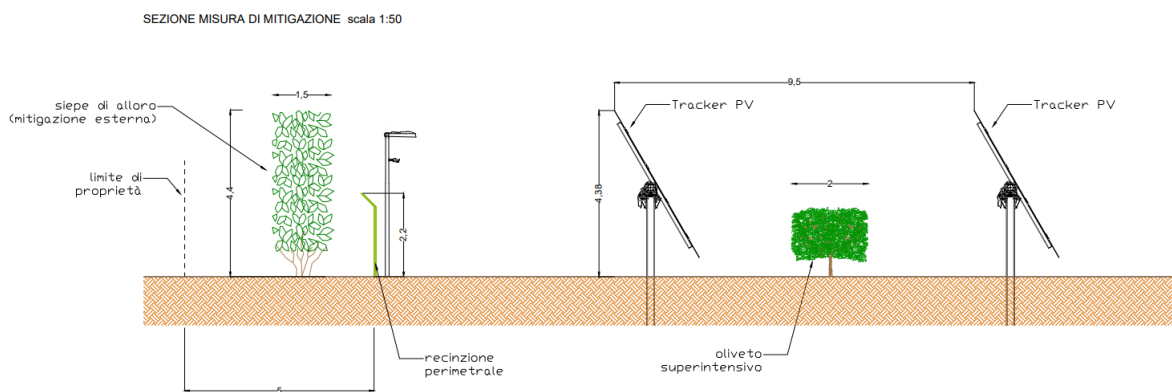
Figura 4-2: Layout misura mitigativa dell'impianto agro-fotovoltaico
