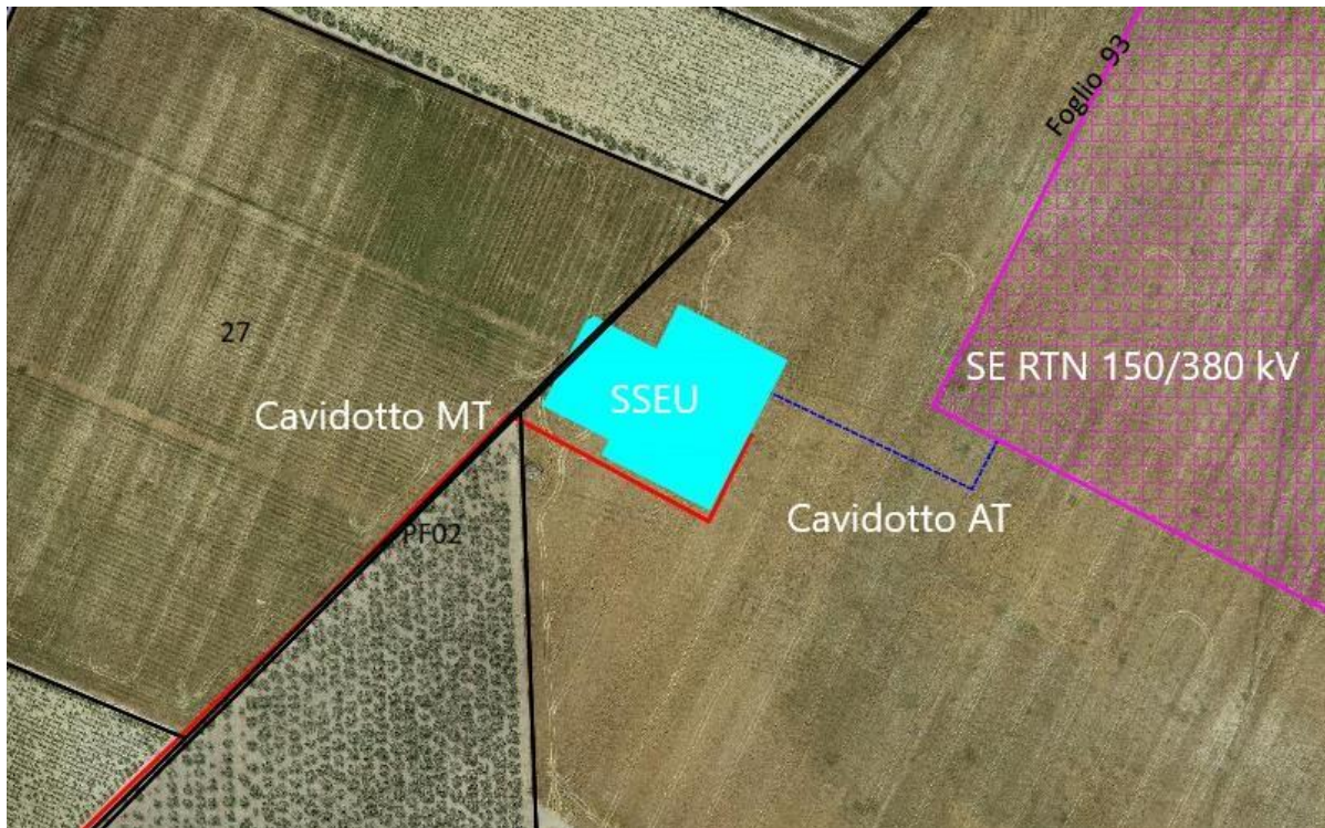
Figura 3-4: Ubicazione Sottostazione Utente su ortofoto
