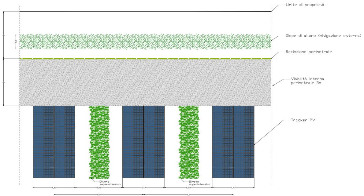
Figura 4-3: Schema esempio d'impianto uliveto super intensivo tra i pannelli fotovoltaici
