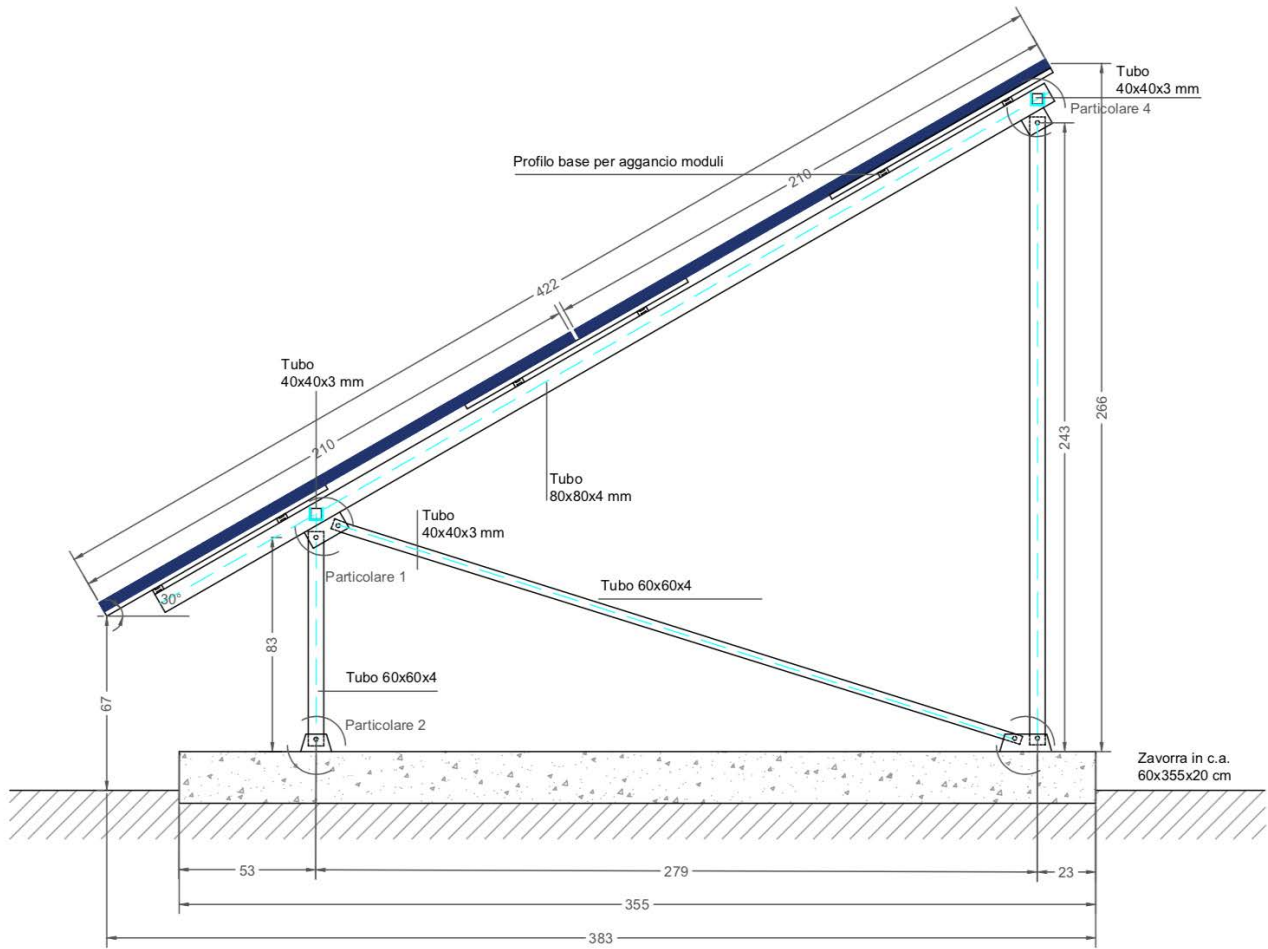
Prospetto laterale scala 1:20
