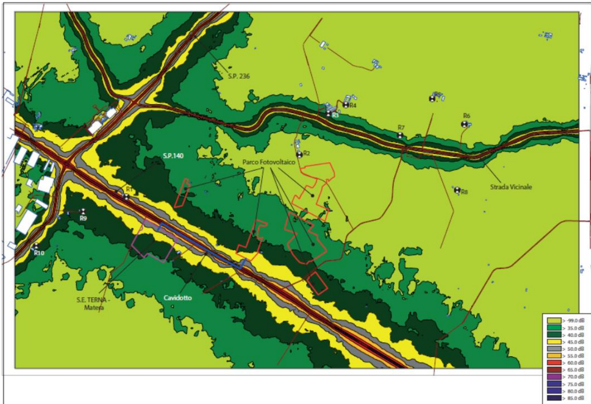
Figura 71: Mappa isolivello sonoro
