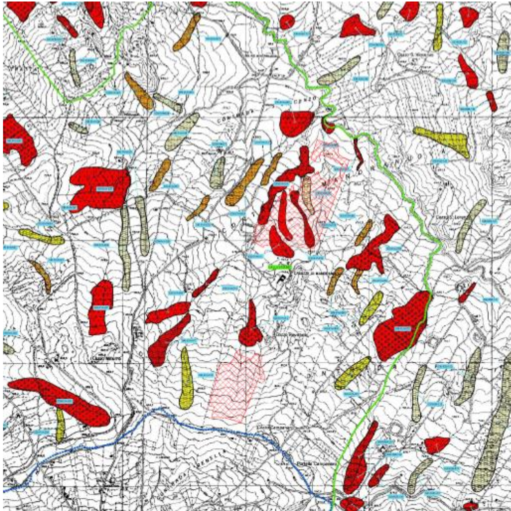
Figura 28 - Stralcio dalla Carta dei Dissesti (BAC030) [Fonte: Regione Sicilia. PAI].
