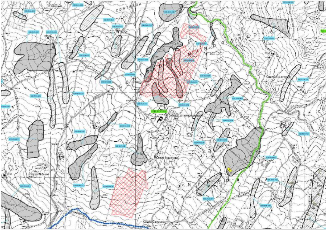
Figura 30 - Stralcio dalla Carta della Pericolosità Geomorfologica (BAC030) [Fonte: Regione Sicilia. PAI].
