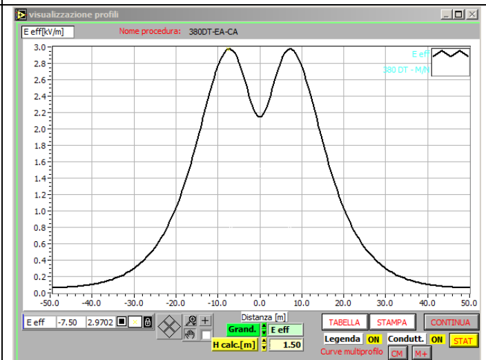
Campo elettrico inferiore a 3kV/m
