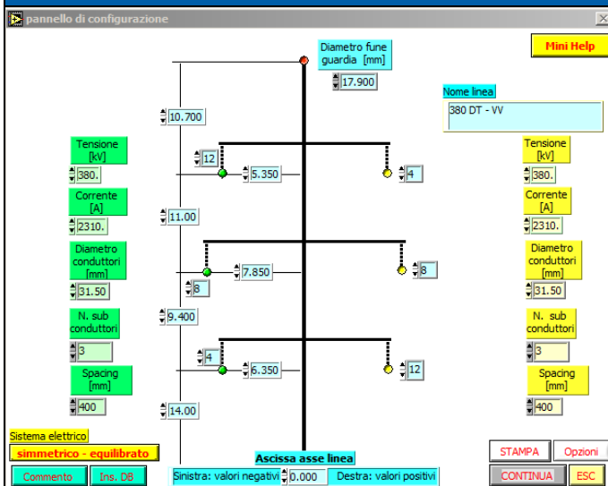
Configurazione 380 DT – Tipo VV
