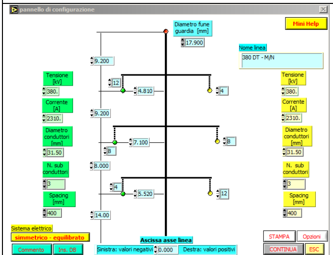
Configurazione 380 DT – Tipo M e Tipo N
