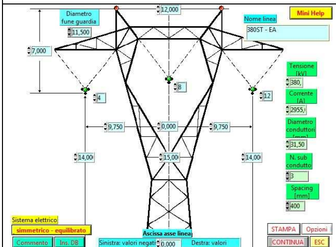
Configurazione 380 ST – Tipo EA
