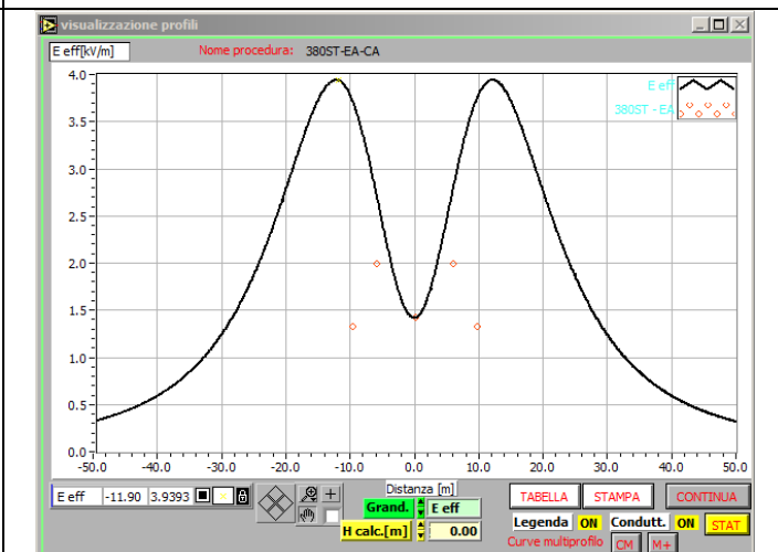
Campo elettrico inferiore a 3.9kV/m
