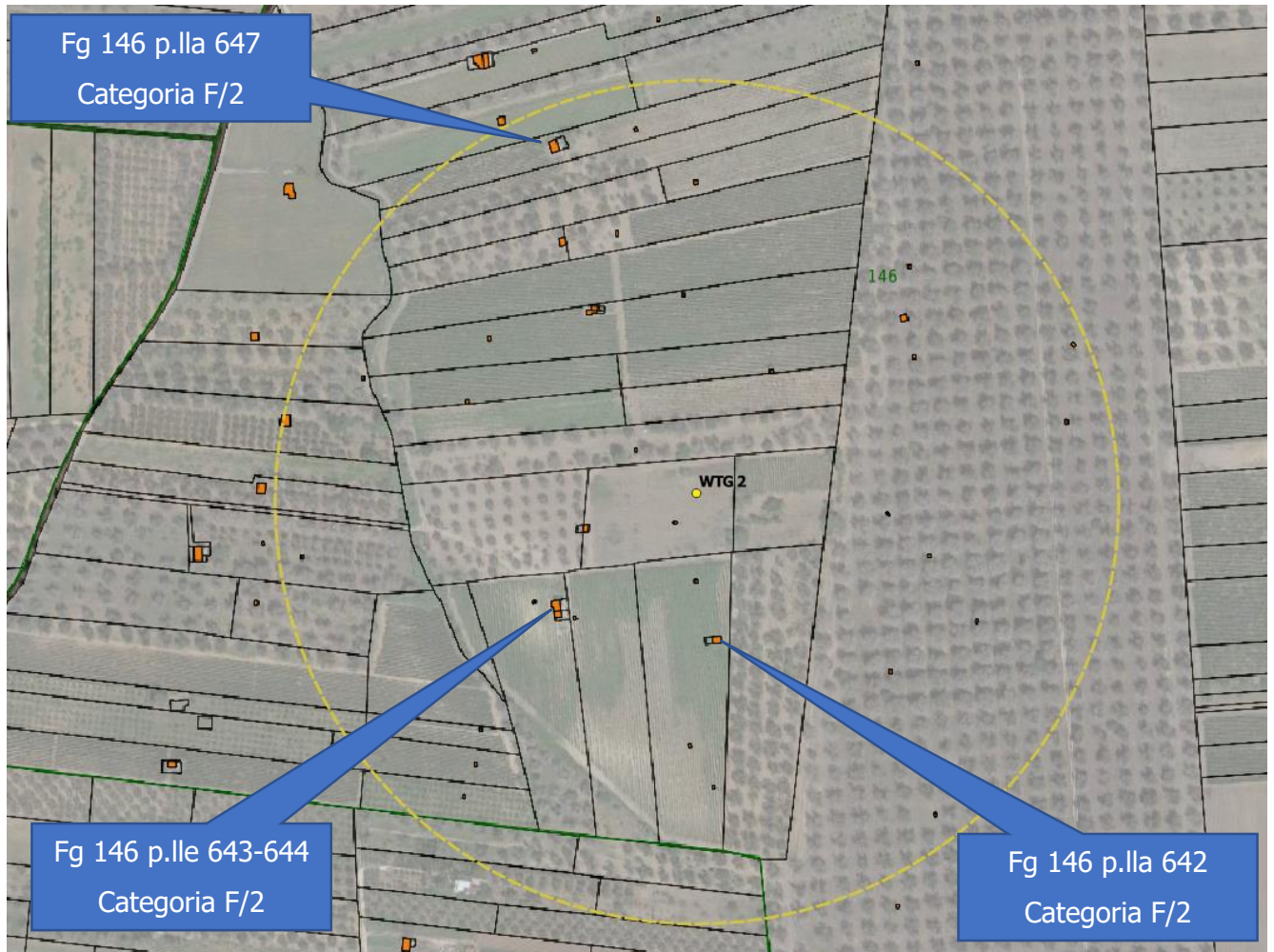
Figure 3 Particolare WTG02
