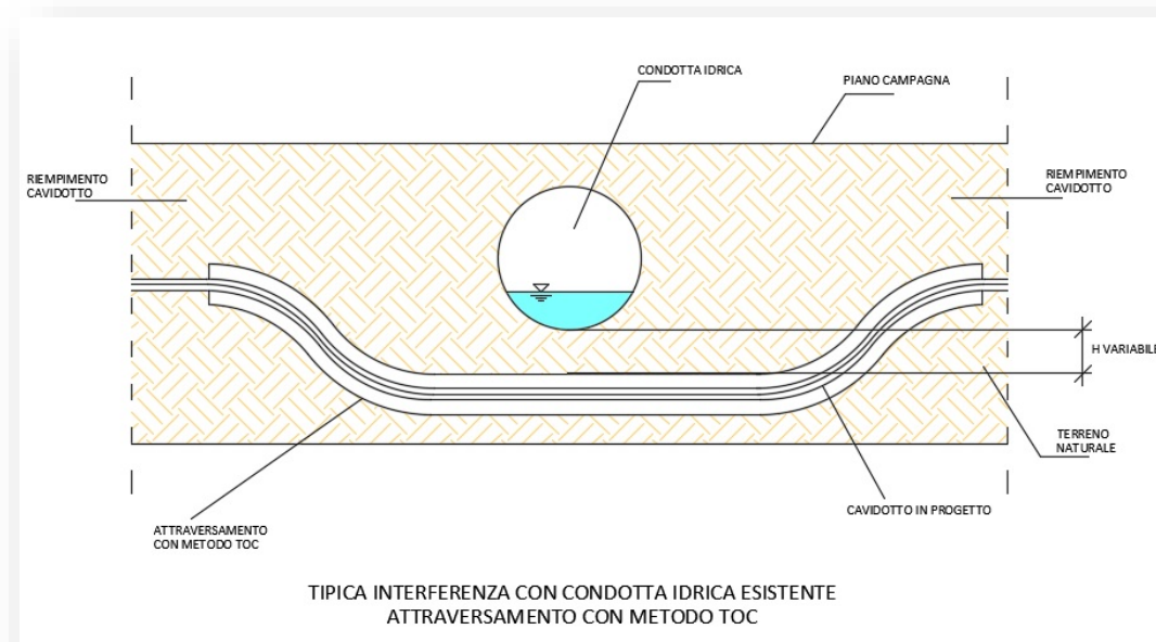
Figura 25- Schema tipico di risoluzione interferenza con condotte idriche esistenti mediante l'utilizzo di metodo TOC
