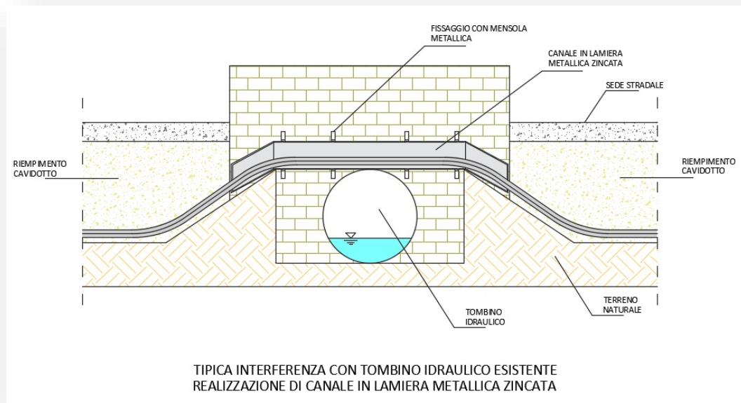
Figura 23- Schema tipico di risoluzione interferenza con tombino idraulico mediante realizzazione di canale in lamiera metallica zincata (staffaggio esterno)
