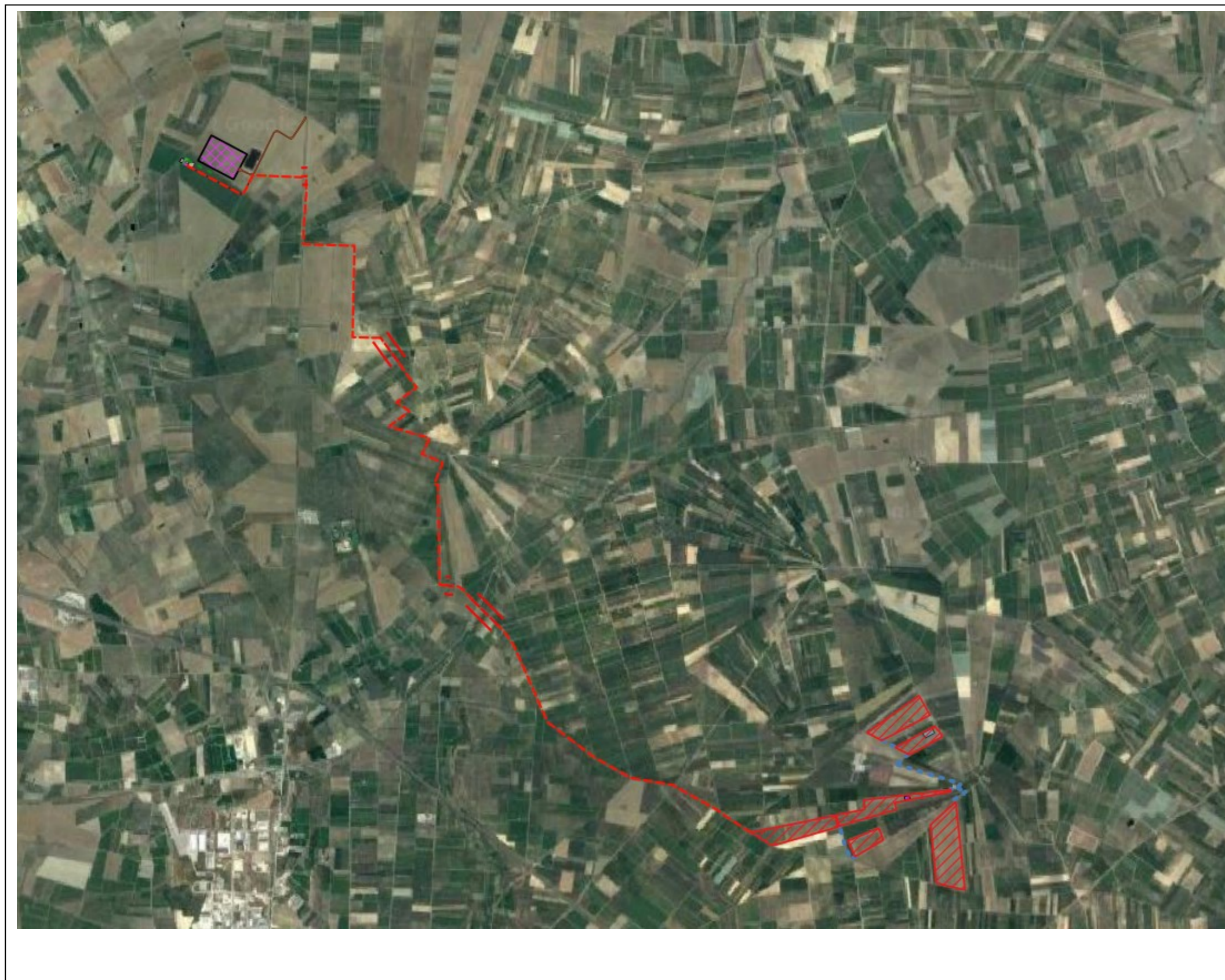
Figura 2 – Particolare Ortofoto con opere di progetto
