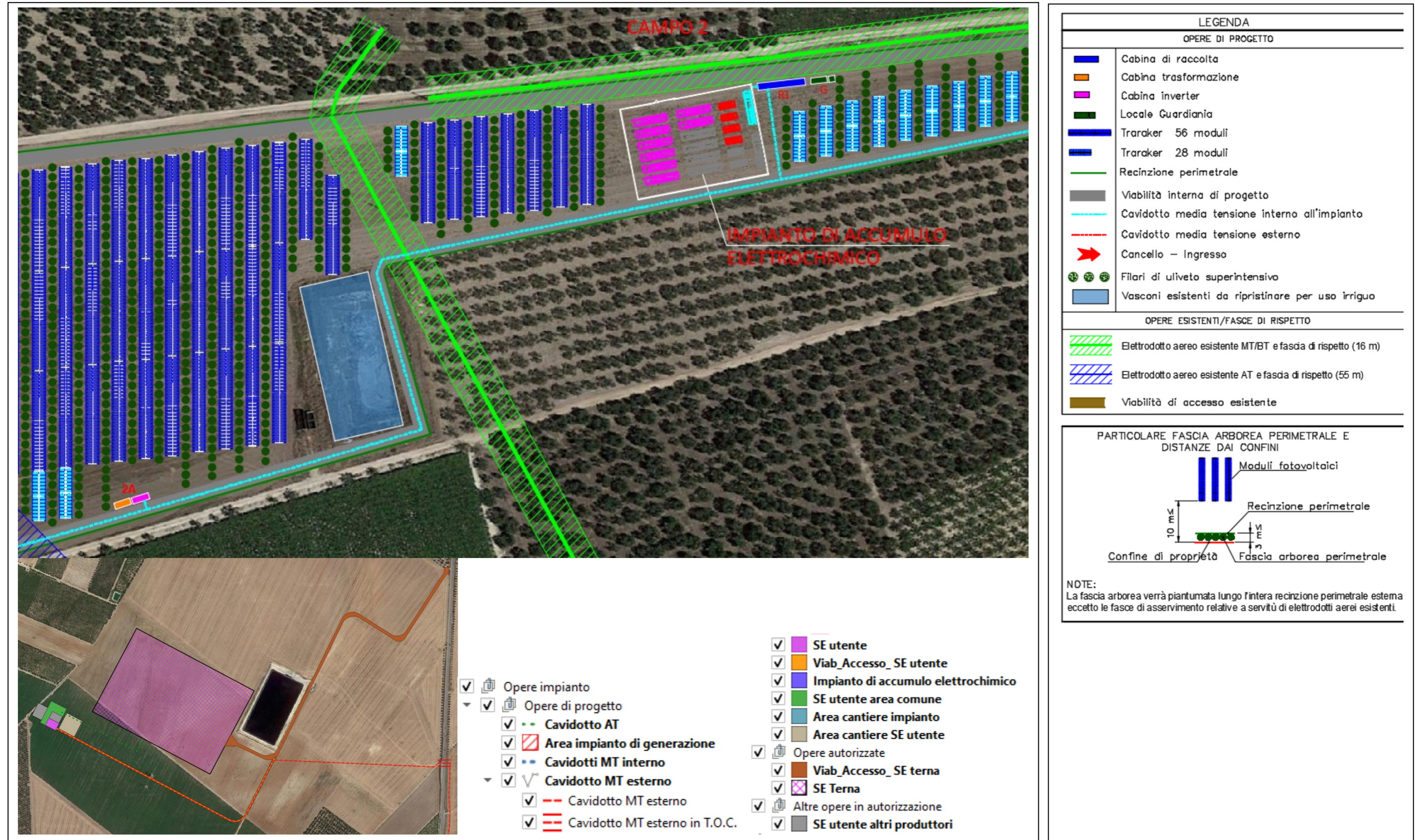
Figura 4 - Particolari stralci sottocampo fotovoltaico e opere di connessione alla RTN
