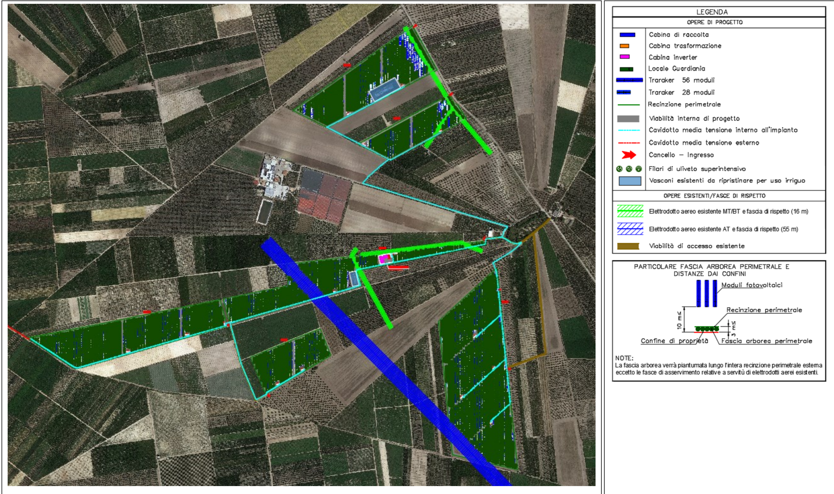
Figura 3 - Layout impianto con legenda
