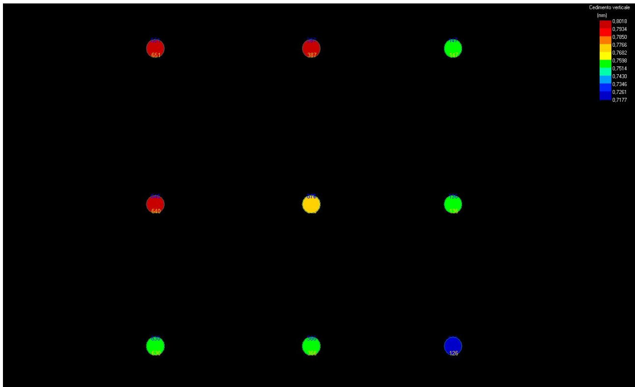
Figura 4 – Cedimenti massimi
