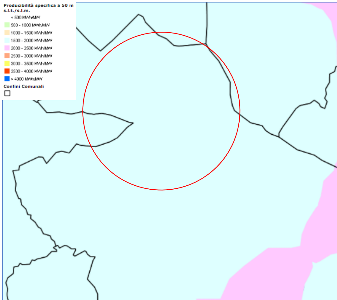
Figura 3 - Produttività specifica a 50 m s.l.t.
