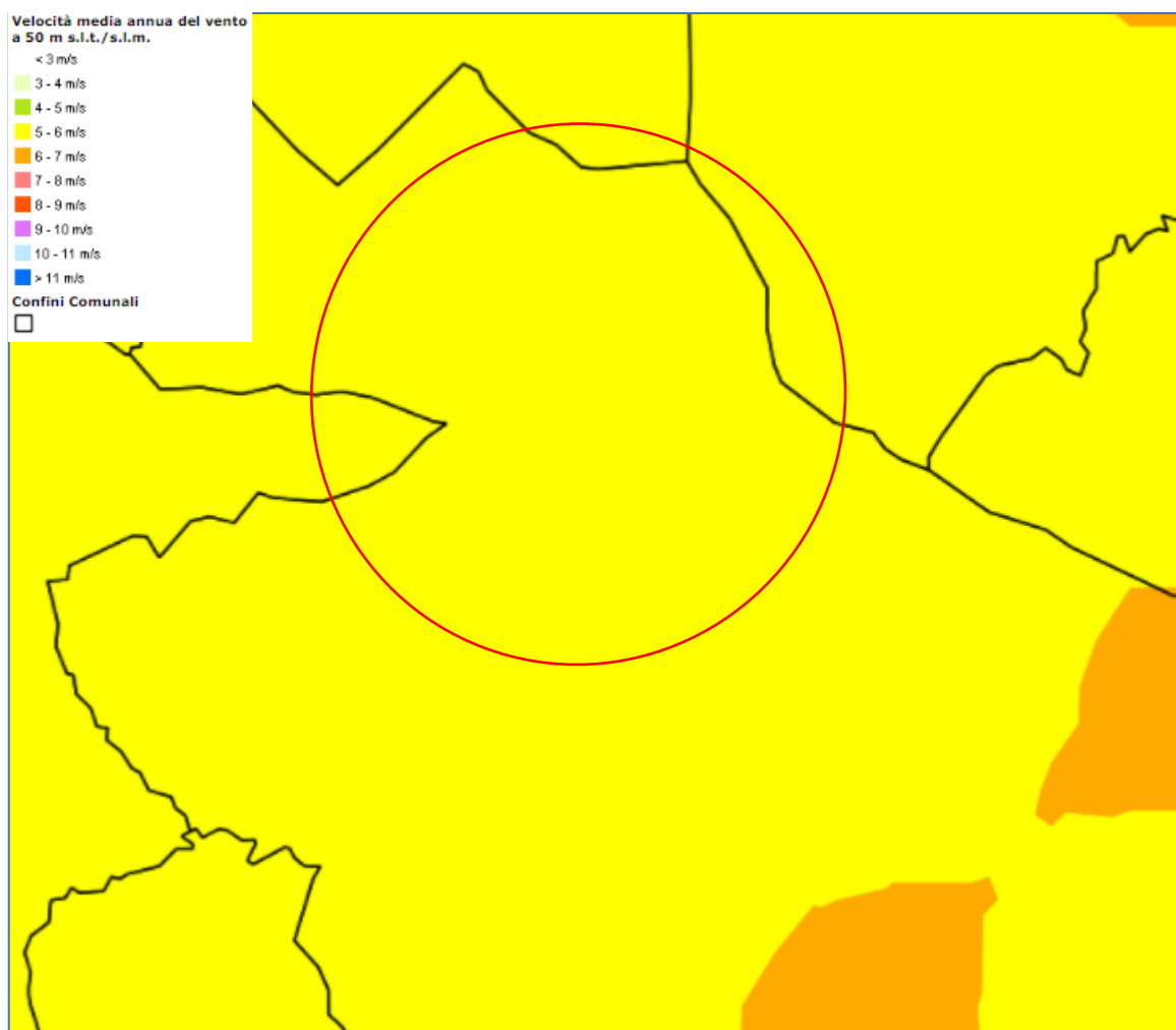
Figura 2 - Velocità media annua del vento a 50 m.s.l.t.
