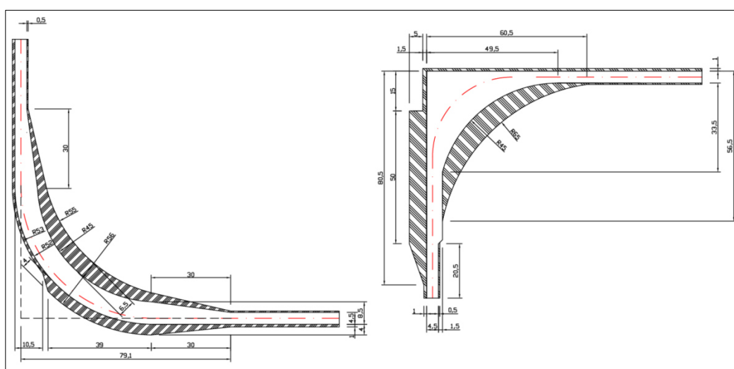
Figura 7 - Particolare realizzazione raccordo strade
