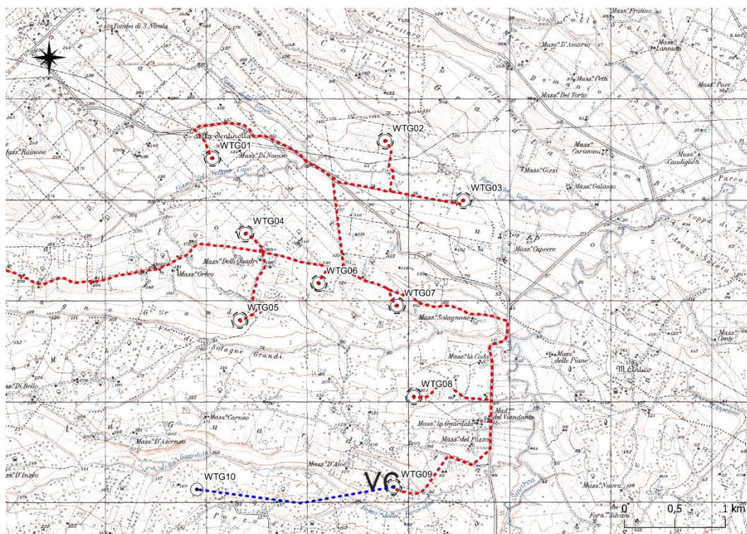
Figura 24 - Sovrapposizione schema layout di partenza a 10 WTG (in blu) e schema definitivo a 9 WTG (in rosso).
