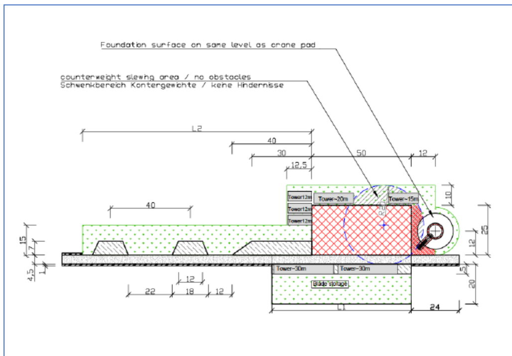
Figura 8 - Piazzola di montaggio
