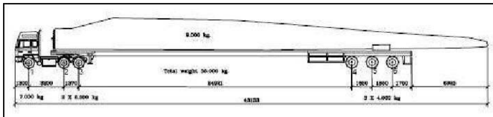
Dimensioni autoarticolato
