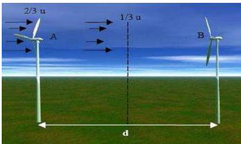
Figura 4 - Effetto di schiera
