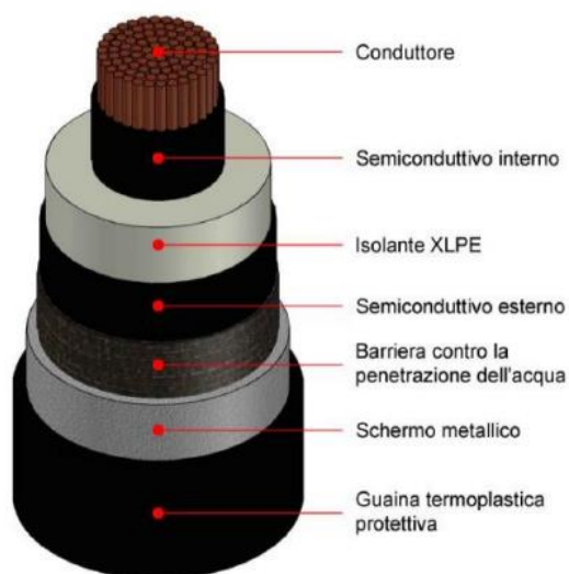
Figura 9 - Esempio di cavo
