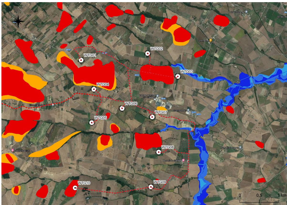
Figura 23 - Ipotesi di layout a 10 aerogeneratori - analisi vincolistica
