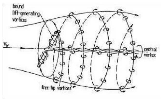
Figura 5 - Vortici e scia
