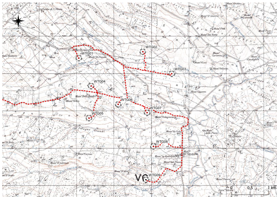
Figura 25 - layout impianto a n.9 aerogeneratori
