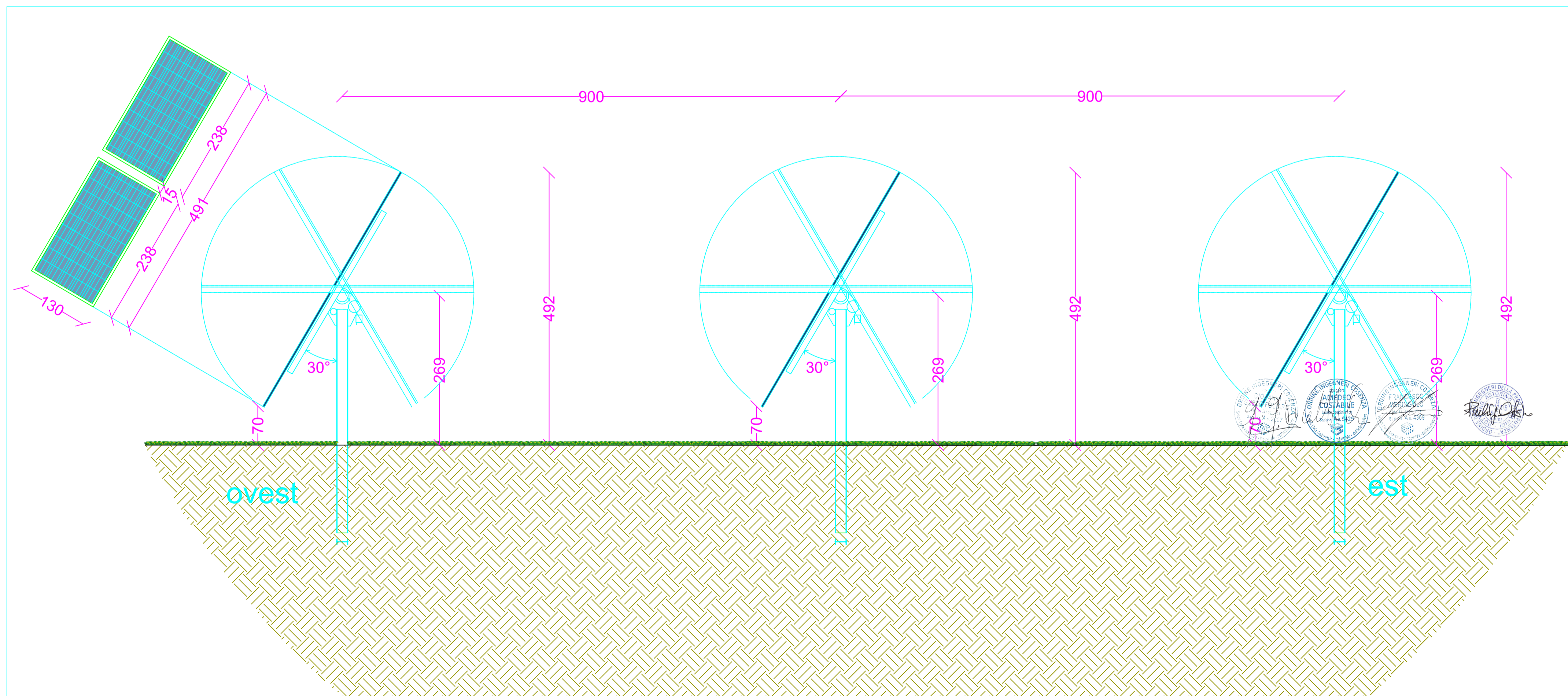
SCHEMA DI SEZIONE TIPO DISPOSIZIONE FILARI NELLA CONFIGURAZIONE TRACKERS - SCALA 1:50
