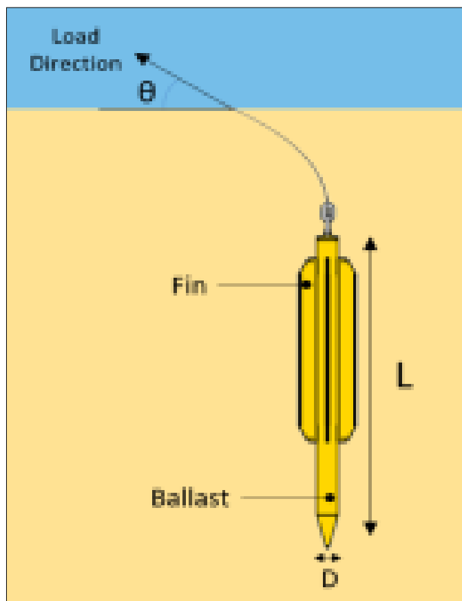
Figura 3.12: Ancoraggio della palo a siluro
