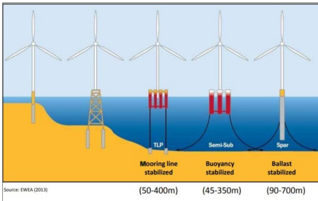
Figura 2.1: Tipi di fondazioni offshore
