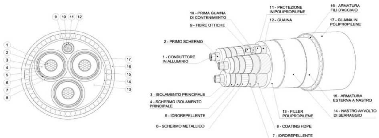
Figura 6 – Struttura cavo a 66 kV
