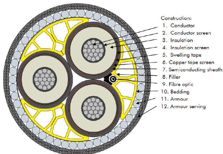
Figura 10 – Struttura cavo 66 kV
