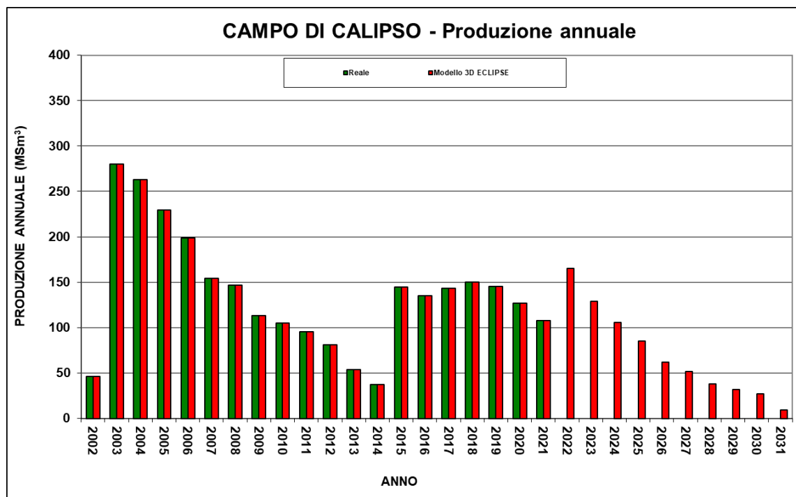
Figura 6 - Campo di Calipso: produzione (annuale) reale e da modello Eclipse 2021
