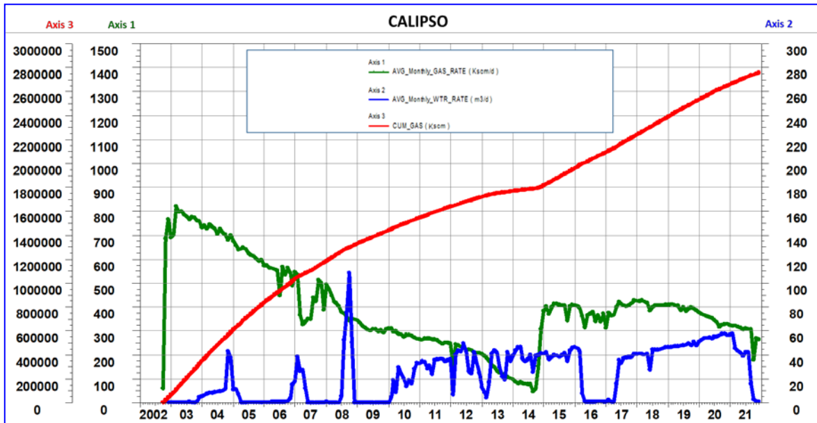
Figura 3 - Campo di Calipso: grafico di produzione storica
