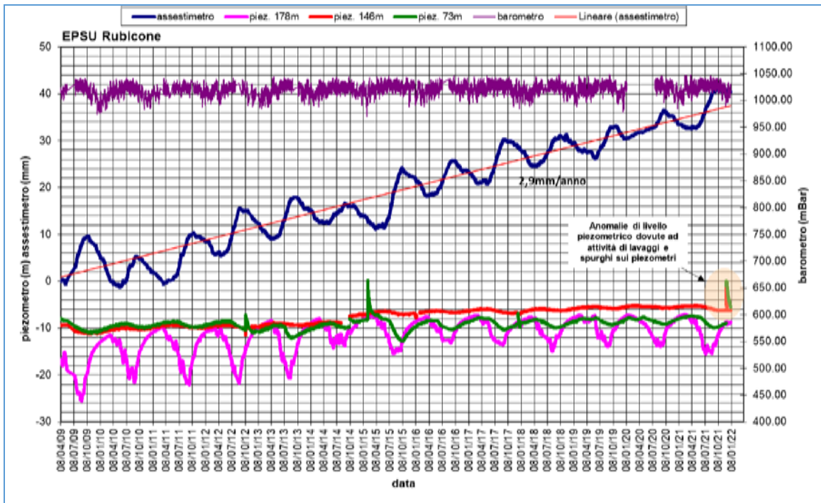
Figura 7B - Stazione EPSU di Rubicone: misure piezometriche, assestimmiche e barometriche
