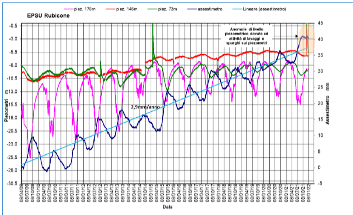
Figura 8B - Stazione EPSU di Rubicone: misure piezometriche e assestimmiche.
