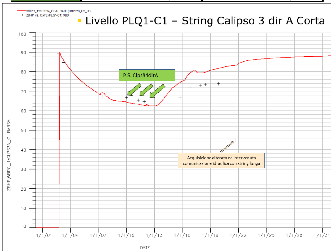
Figura 7 - Campo di Calipso: pressioni statiche misurate e modello Eclipse 2021 (livello PLQ1-C1)
