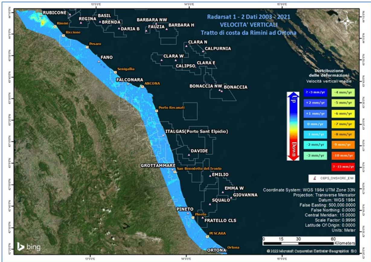
Figura 10 - Campo di Calipso: analisi dei dati SAR dal 2003 al 2021
