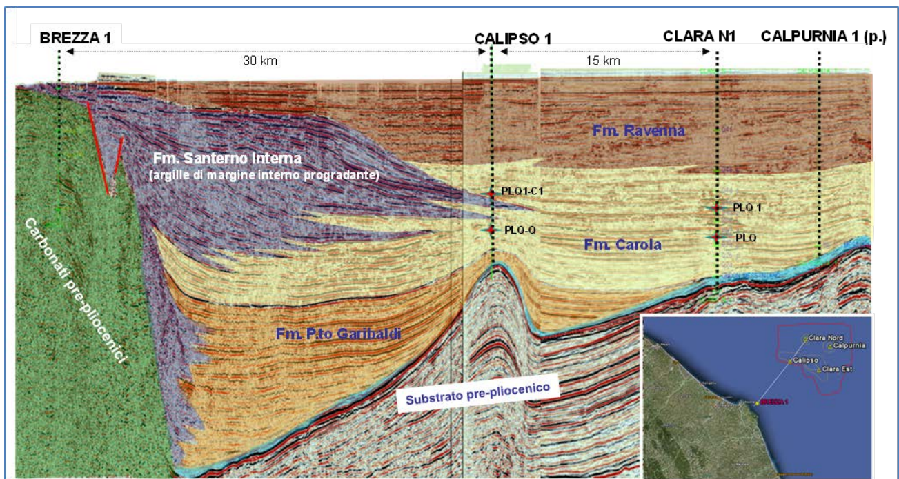
Figura 9 - Sezione sismica interpretata
