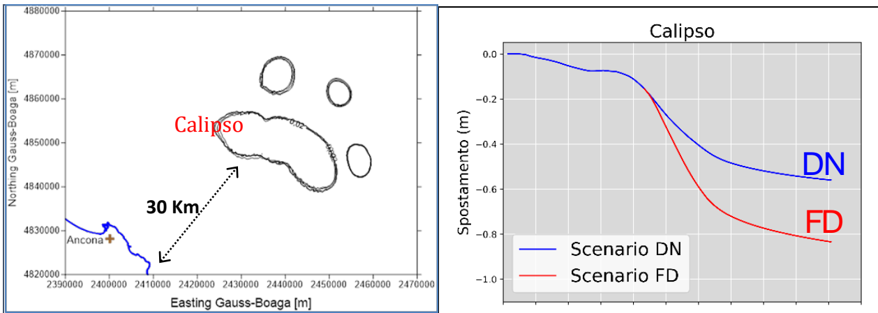
Figura 8 - Campo di Calipso: A sx: mappa con la posizione della linea di iso-subsidenza 2 cm nel periodo 2021-2050 per entrambi gli scenari considerati (DN e FD). La distanza minima resta pari o superiore ai 30km, e rimane pressochè invariata per l'intera durata del periodo. A dx : evoluzione della subsidenza in corrispondenza della p.ma Calipso nei due scenari considerati (DN e FD).
