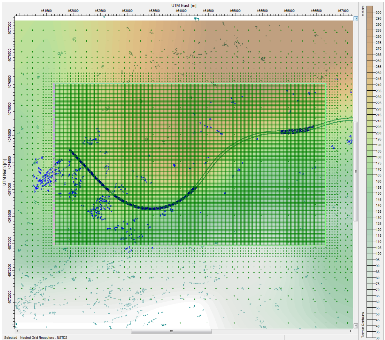
Fig. 7.7 - Vista planimetrica – Schematizzazione modello dispersivo Aermod-View
