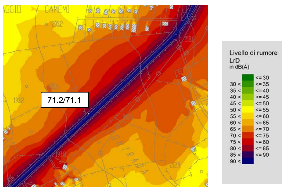
Fig. 6.1 - Distribuzione delle isofoniche per il punto di misura M10-L11
