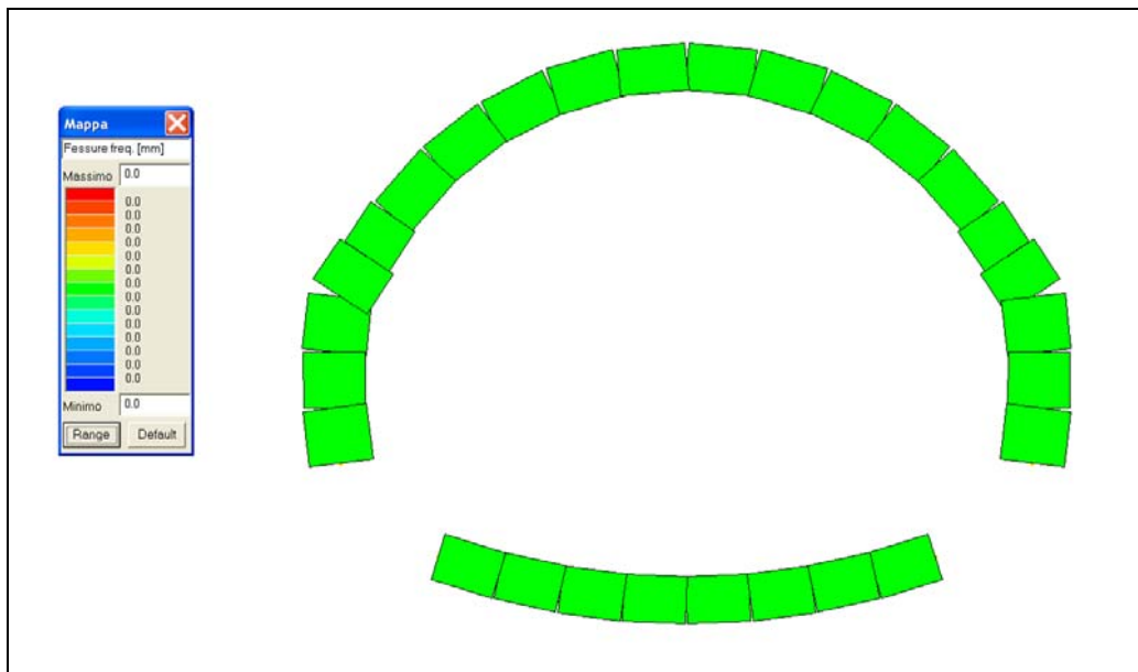
Fig. 8.16 - Op.24 "Galleria Occhipinti" Ampiezza fessure CMB7 SLE frequenti
