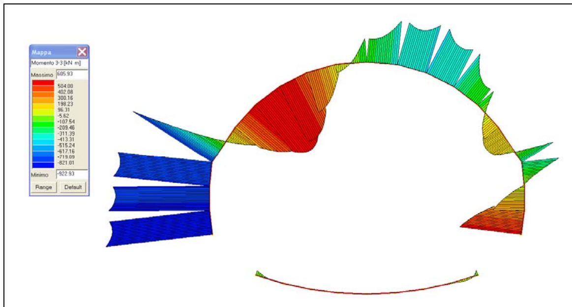
Fig. 8.12 - Op.24 "Galleria Occhipinti" Momento flettente max in CMB3 SLV
