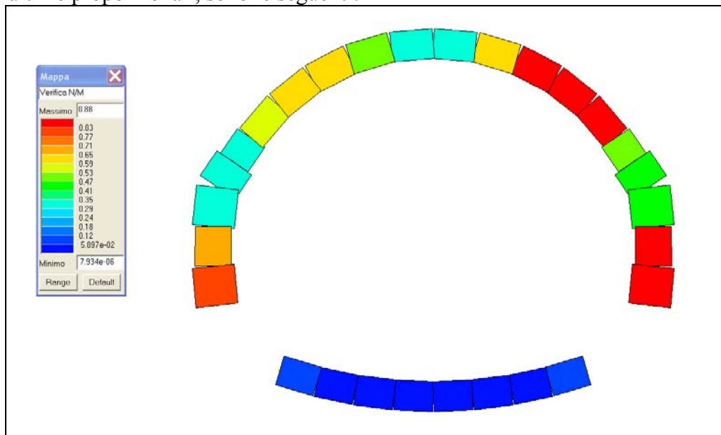
Fig. 8.4 - Op.8 "Galleria Caddame" Verifica N/M
