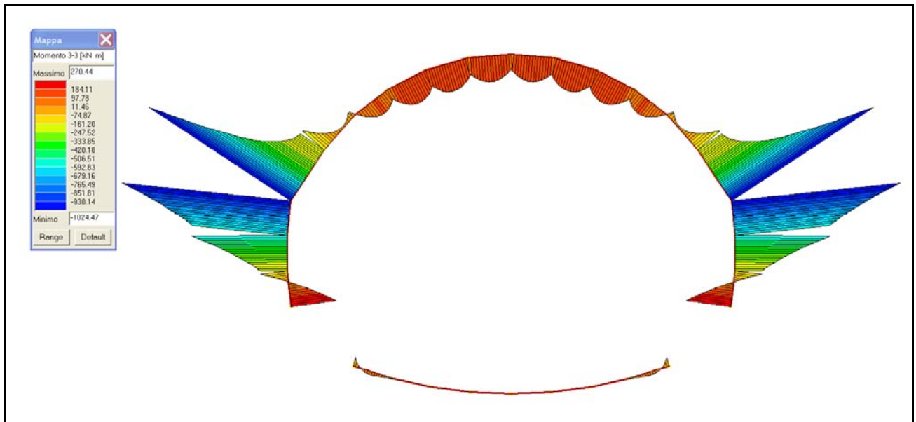
Fig. 8.13 - Op.24 "Galleria Occhipinti" Momento flettente max in CMB1
