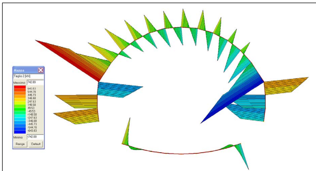
Fig. 8.15 - Op.24 "Galleria Occhipinti" Sforzo di taglio max in CMB1
