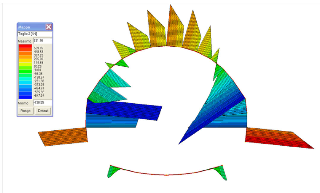
Fig. 8.5 - Op.8 "Galleria Caddame" Sforzo di taglio max in CMB3 SLV
