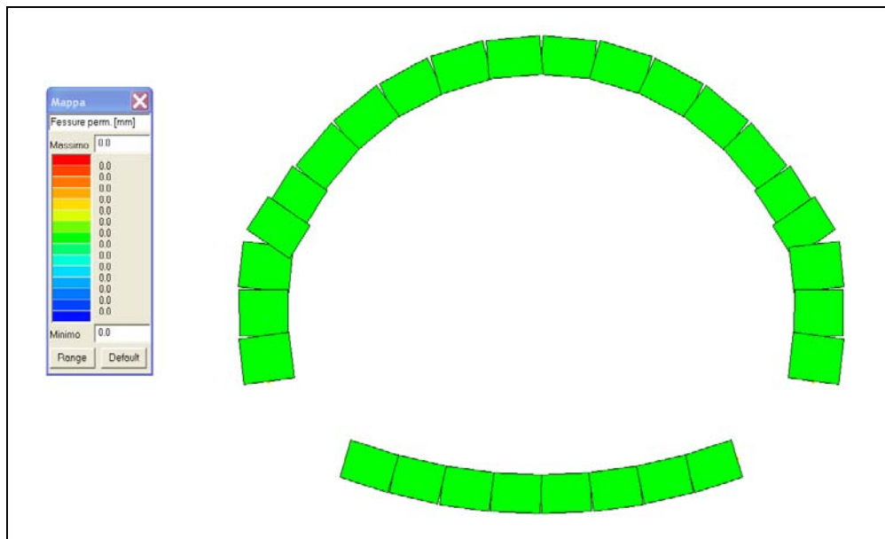
Fig. 8.17 - Op.24 "Galleria Occhipinti" Ampiezza fessure CMB8 SLE permanenti
