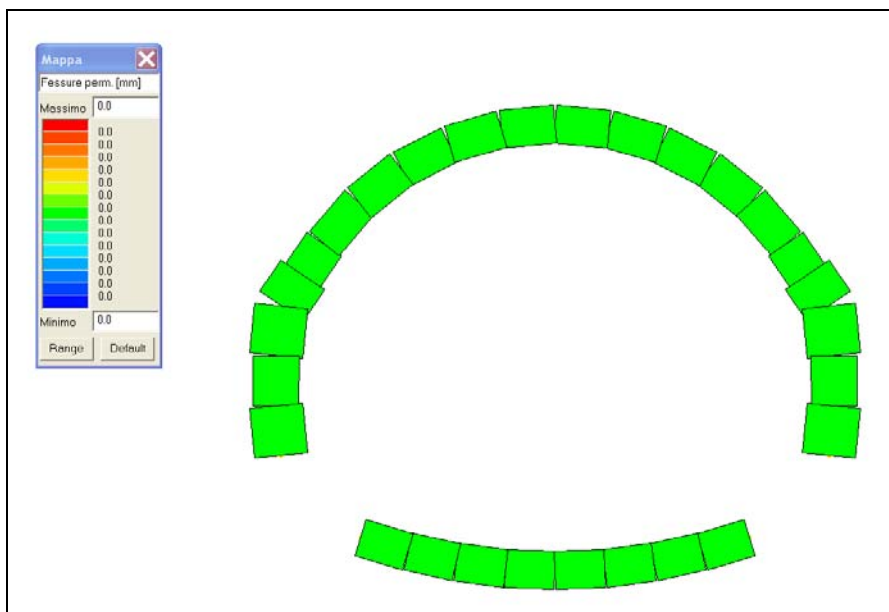
Fig. 8.7 - Op.8 "Galleria Caddame" Ampiezza fessure CMB8 SLE permanenti
