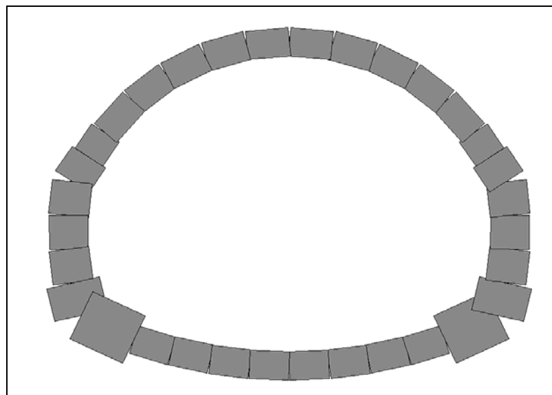
Fig. 6.3 - Op.24 "Galleria Occhipinti" Modello di calcolo
