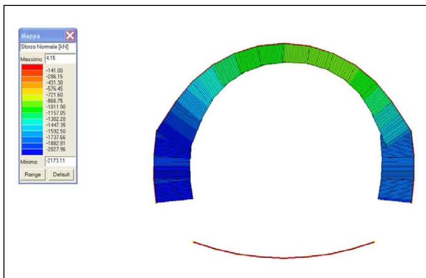
Fig. 8.1 - Op.8 "Galleria Caddame" Sforzo normale max in CMB1
