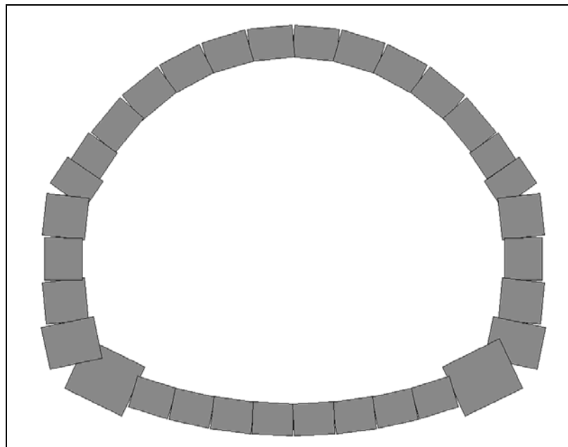
Fig. 6.1 - Op.8 “Galleria Caddame” Modello di calcolo
