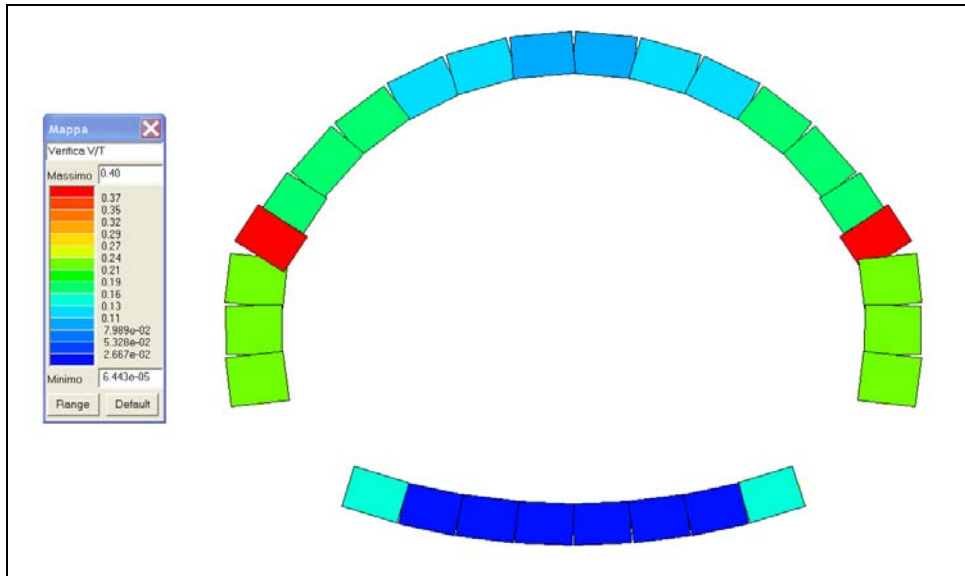
Fig. 8.20 - Op.24 "Galleria Occhipinti" Verifica al fuoco V/T
