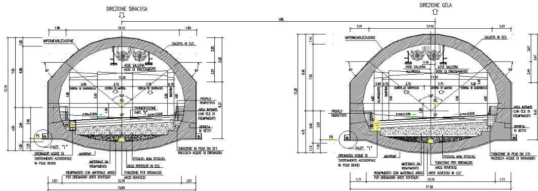
Fig. 1.1 - Sezioni fornici "Galleria Caddame"
