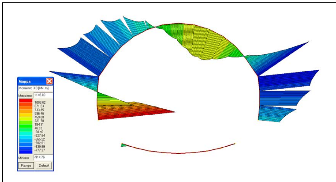
Fig. 8.3 - Op.8 "Galleria Caddame" Momento flettente max in CMB1
