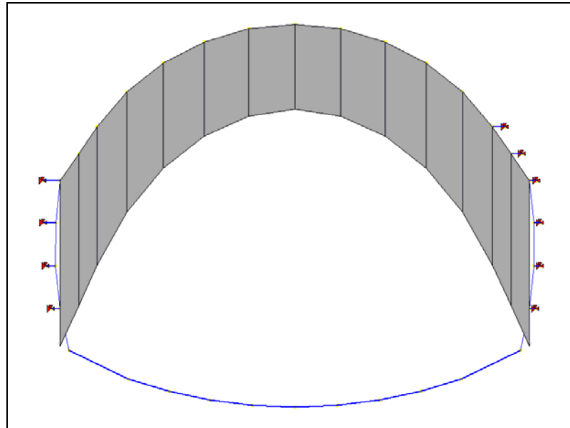
Carico verticale permanente da ricopertura.
