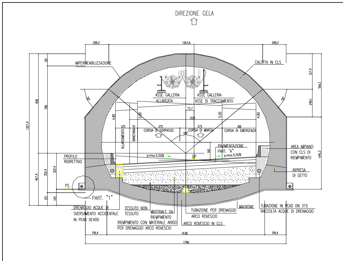
Fig. 1.10 - Op.24 "Galleria Occhipinti" sezione tipo artificiale
