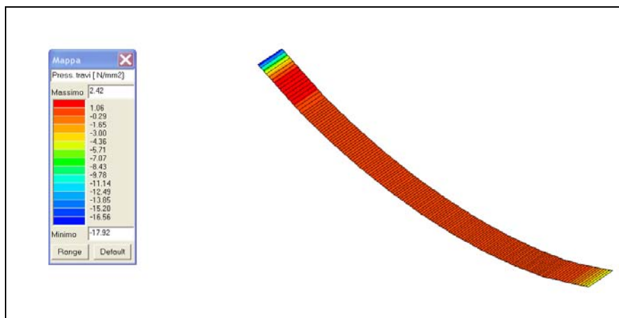
Fig. 8.8 - Op.8 "Galleria Caddame" Pressione di contatto in CMB1
