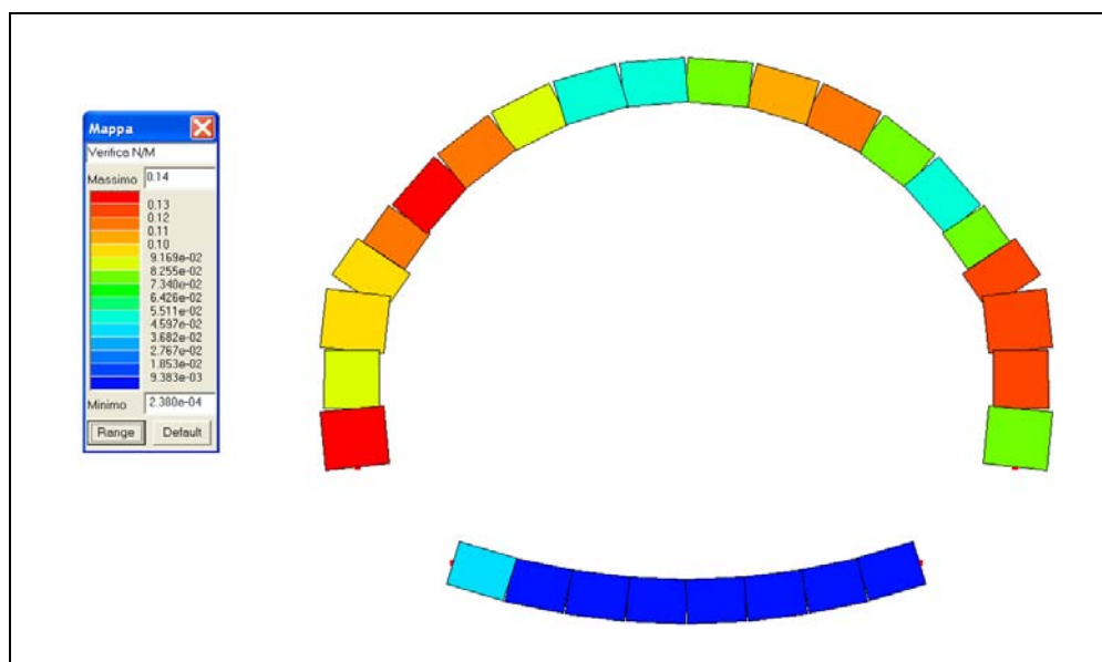
Fig. 8.9 - Op.8 "Galleria Caddame" Verifica al fuoco N/M
