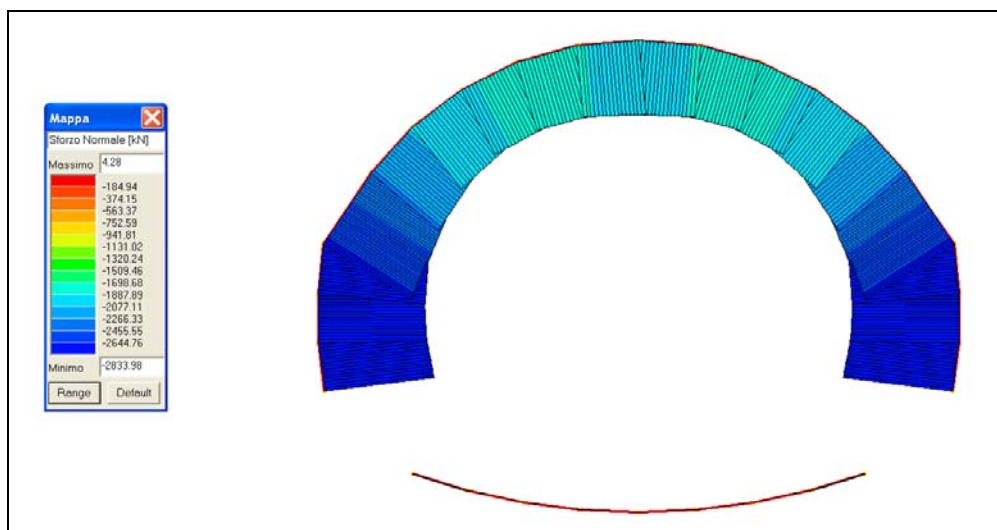
Fig. 8.11 - Op.24 "Galleria Occhipinti" Sforzo normale max in CMB1
