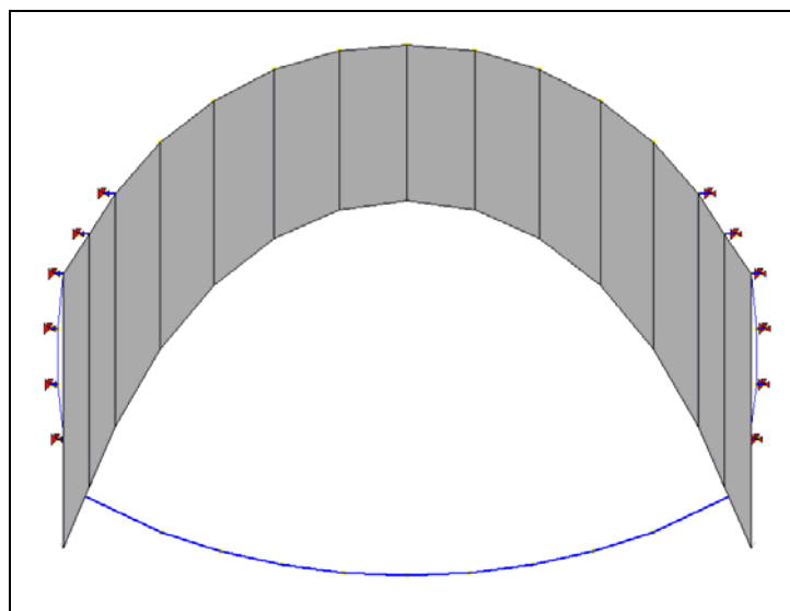
Carico verticale permanente da ricopertura.
