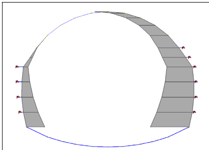
Carico orizzontale a riposo da ricopertura.
