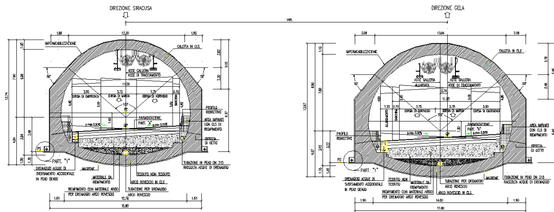
Fig. 1.4 - Sezioni fornici "Galleria Occhipinti"
