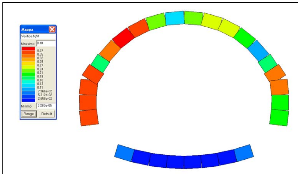
Fig. 8.14 - Op.24 "Galleria Occhipinti" Verifica N/M
