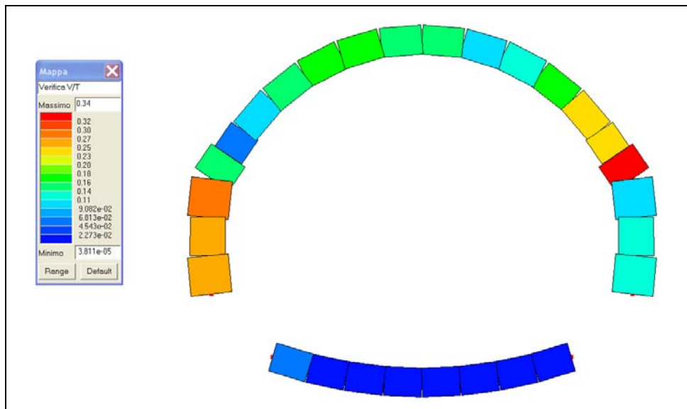
Fig. 8.10 - Op.8 "Galleria Caddame" Verifica al fuoco V/T
