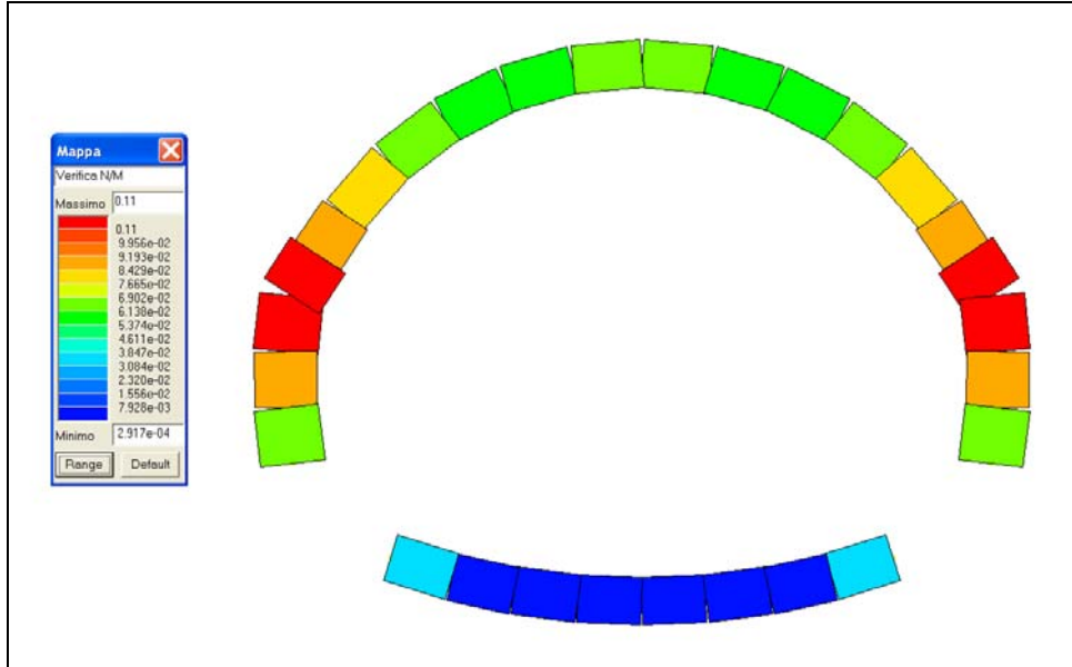
Fig. 8.19 - Op.24 "Galleria Occhipinti" Verifica al fuoco N/M
