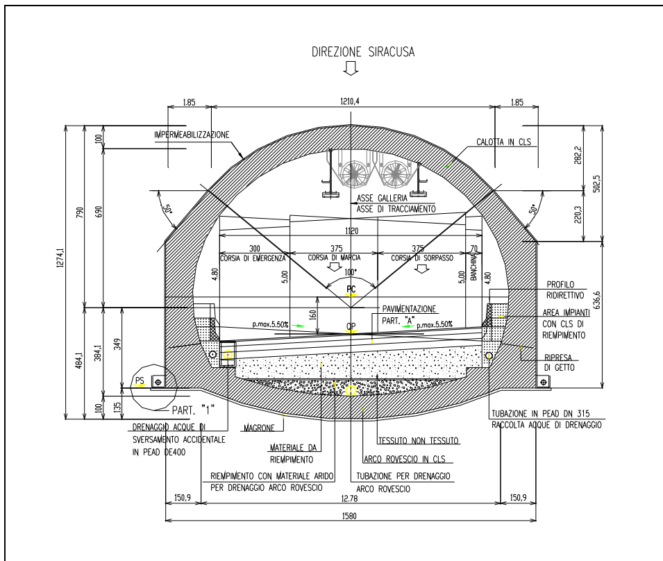
Fig. 1.8 - Op.8 “Galleria Caddame” sezione tipo artificiale
