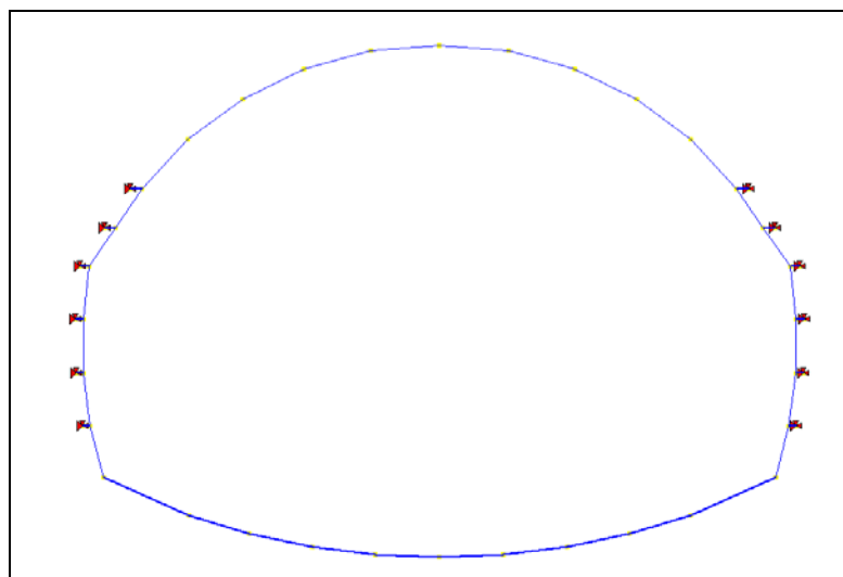
Fig. 6.4 - Op.24 "Galleria Occhipinti" Mesh di calcolo
