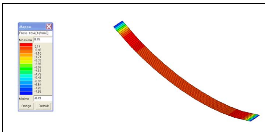
Fig. 8.18 - Op.24 "Galleria Occhipinti" Pressione di contatto in CMB1
