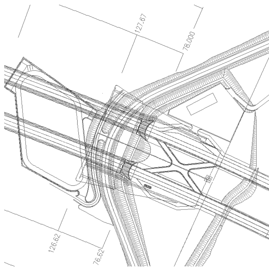
Fig. 1.2 - Imbocco lato Siracusa "Galleria Caddame"
