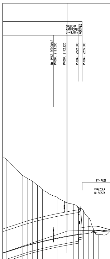
Fig. 1.7 - Op.8 "Galleria Caddame" sezione longitudinale imbocco Gela
