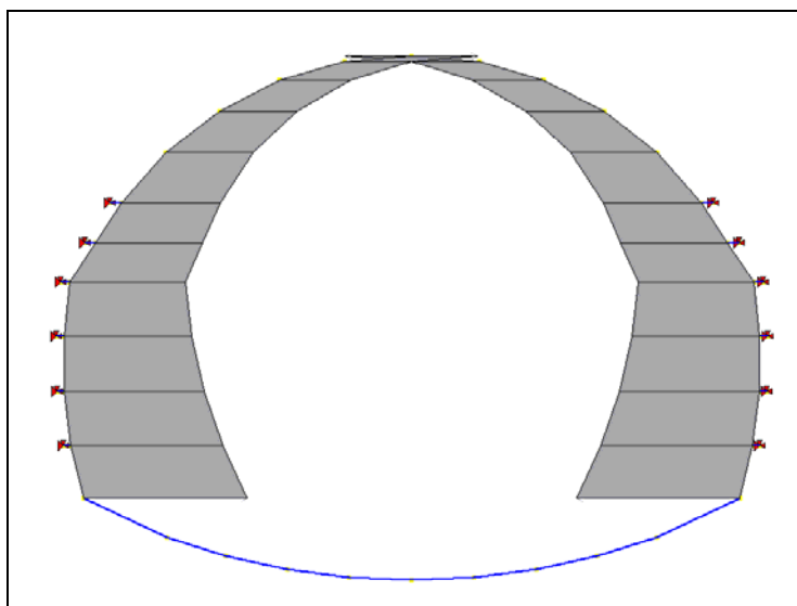
Carico orizzontale a riposo da ricopertura.
