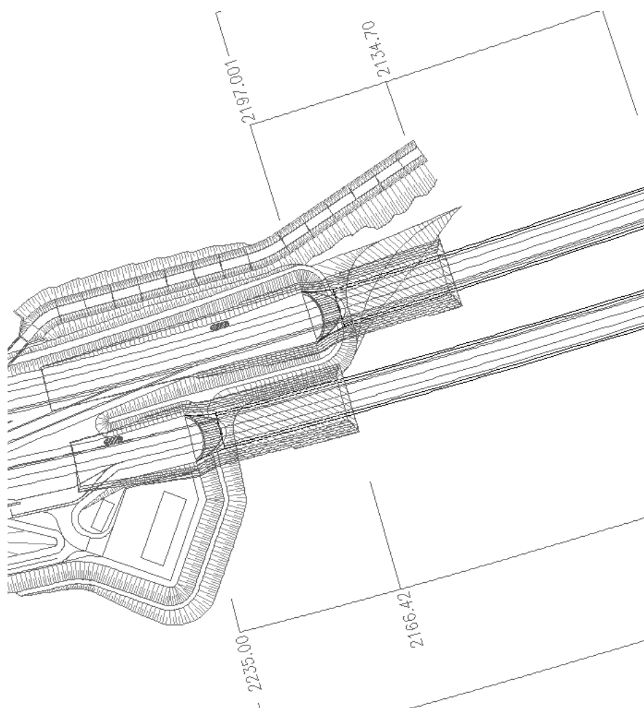
Fig. 1.3 - Imbocco lato Gela "Galleria Caddame"
