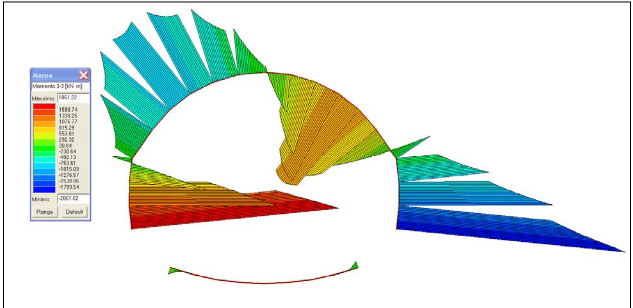
Fig. 8.2 - Op.8 "Galleria Caddame" Momento flettente max in CMB3 SLV
