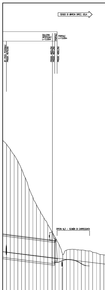
Fig. 1.9 - Op.24 "Galleria Occhipinti" sezione longitudinale imbocco Gela
