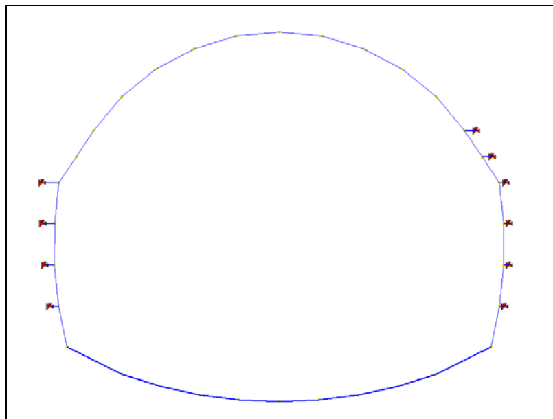
Fig. 6.2 - Op.8 "Galleria Caddame" Mesh di calcolo
