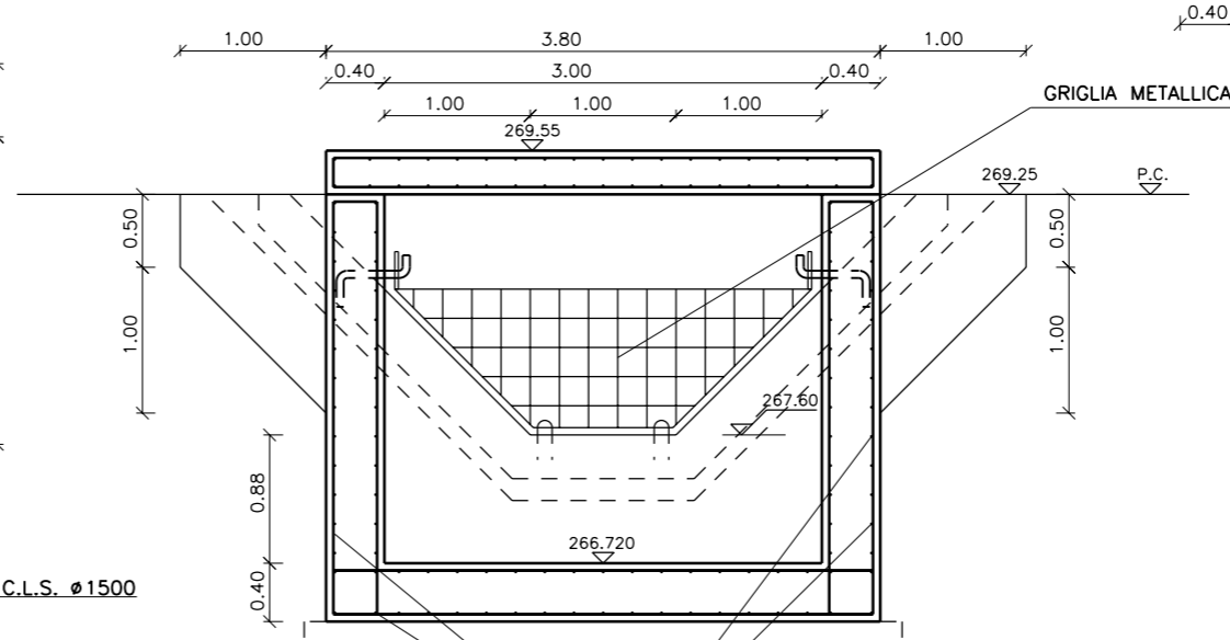
POZZETTO B SEZIONE 1-1
