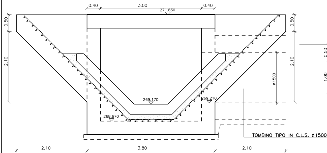
POZZETTO A SEZIONE 1-1
