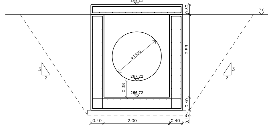
POZZETTO B SEZIONE 2-2
