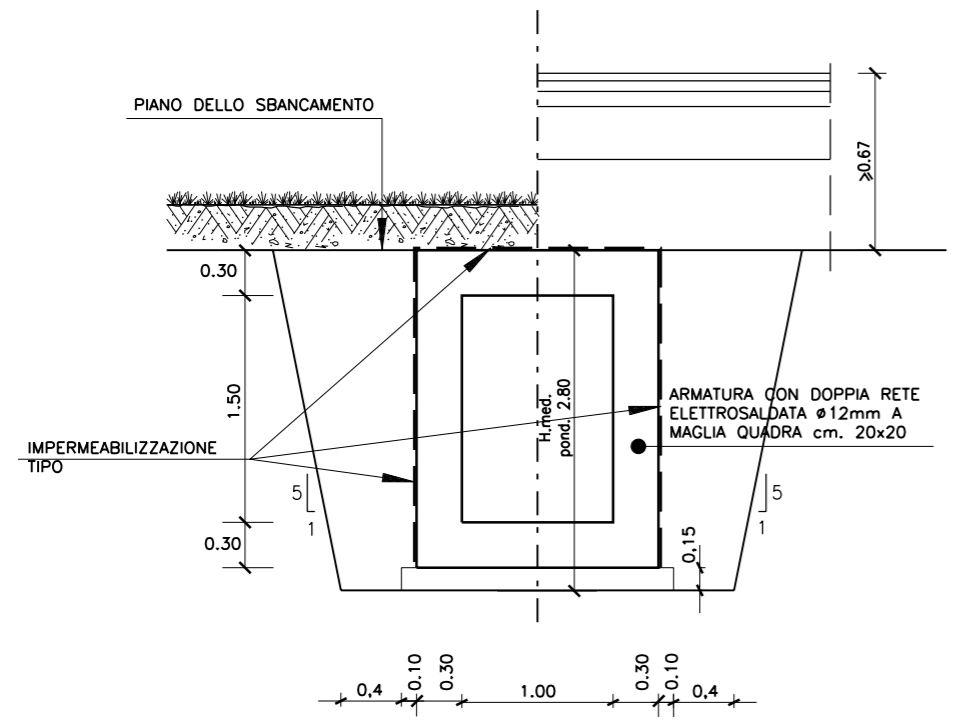
SEZIONE TIPO DELLA TOMBINATURA VALE 110.32m
