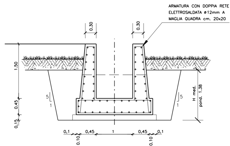
SEZIONE TIPO DELLA CANALETTA
