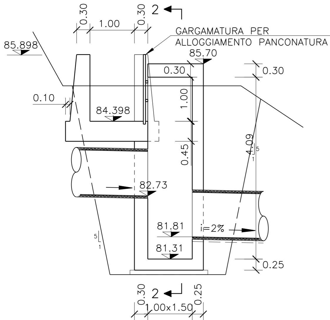
SEZIONE 1-1
