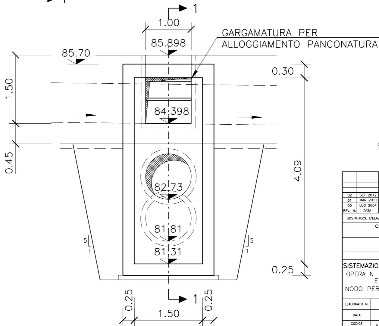
SEZIONE 2-2
