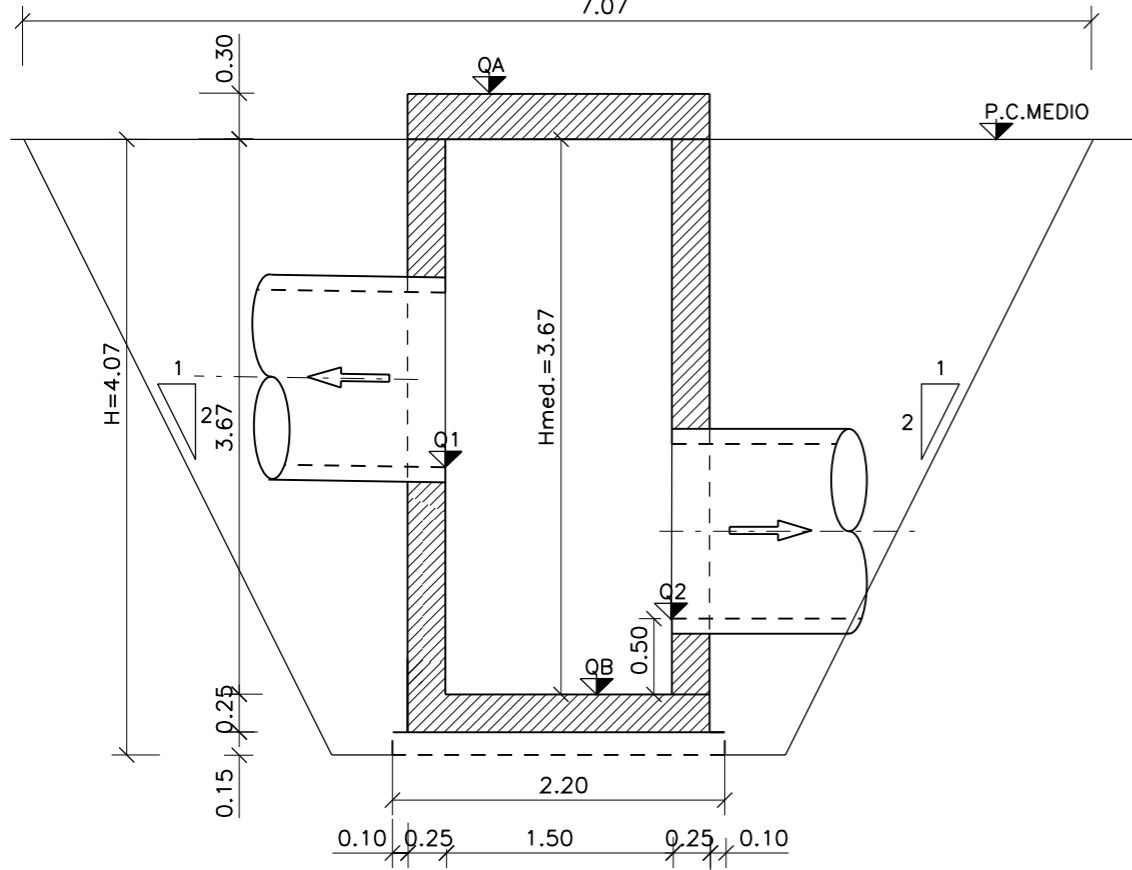
SEZIONE 1-1 7.07
