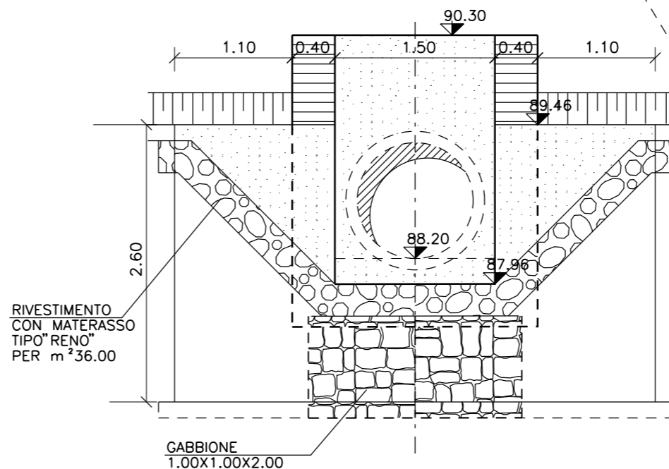
SEZIONE 2-2
