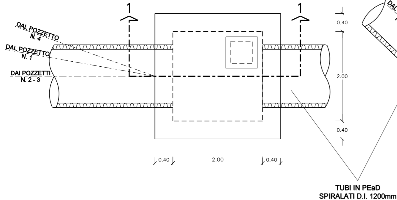
PIANTA POZZETTI N. 2 - 3 - 4 - 5
