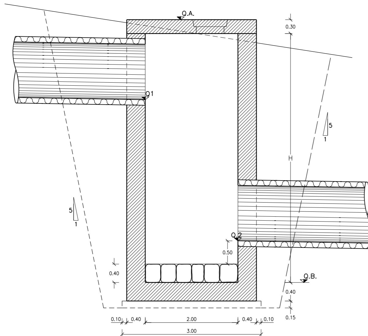
SEZIONE 1 - 1
