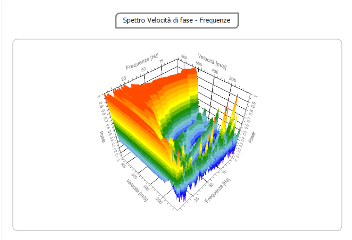
Fig. 33: spettro di velocità – frequenze 3D acquisito M2
