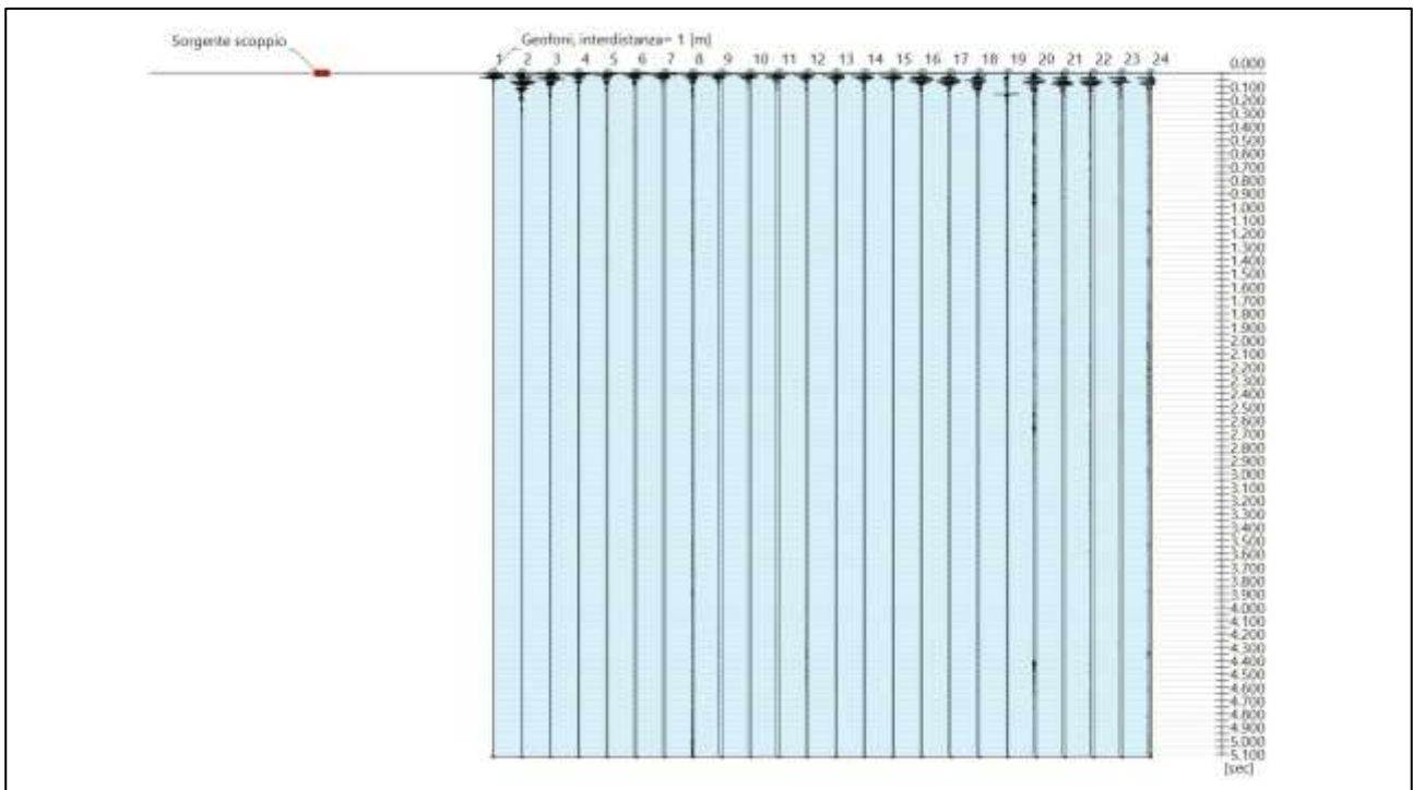
Fig.39: sismogrammi acquisiti durante l'esecuzione della MASW- M3
