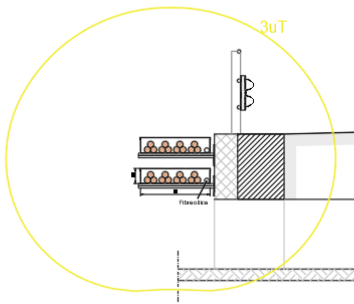
Figura 9. Sovrapposizione della curva di isolivello di B=3\mu\text{T} con tipologico sezione cavidotto MT su passerella ancorata al ponte
