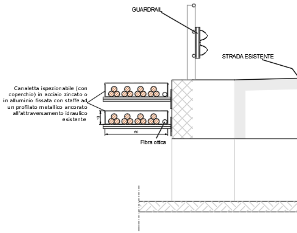
Figura 6. Tipologico sezione cavidotto MT in fiancheggiamento al ponte/cavalcavia
