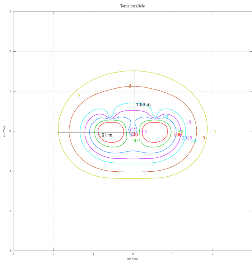
Figura 12. Curve isolivello andamento induzione magnetica B dei cavi MT posati nel pozzetto di giunzione
