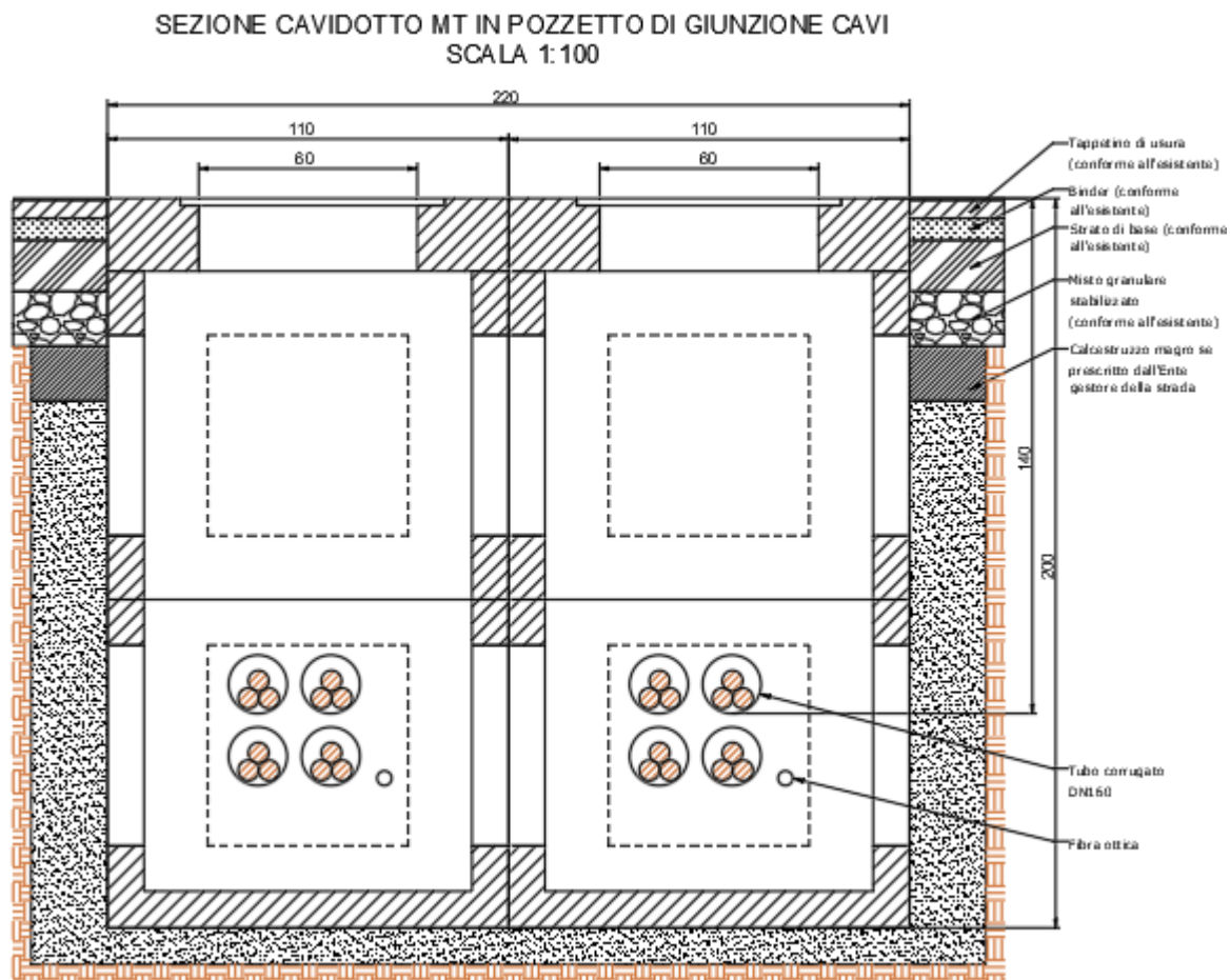
Figura 11. Tipologico sezione cavidotto MT in pozzetto di giunzione cavi
