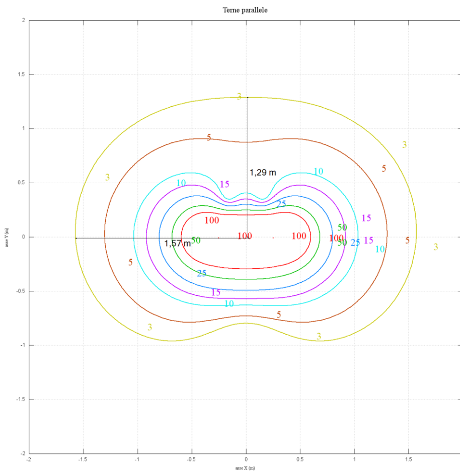
Figura 5. Curve isolivello andamento induzione magnetica B
