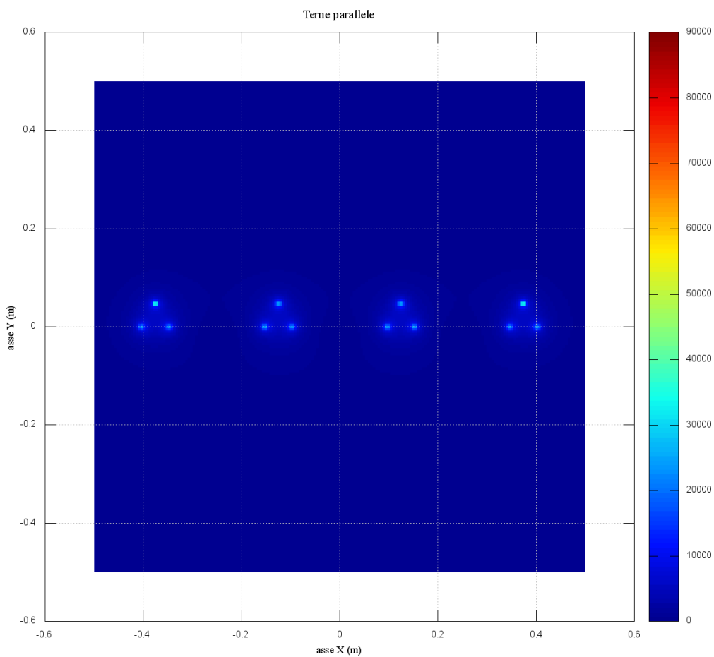
Figura 4. Andamento induzione magnetica B bidimensionale
