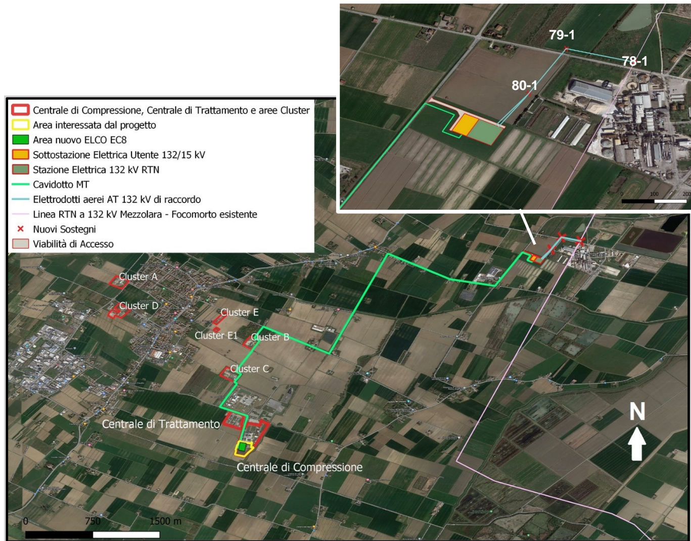
Figura 4.1-2 Area delle Opere in centrale ed Opere accessorie in progetto
