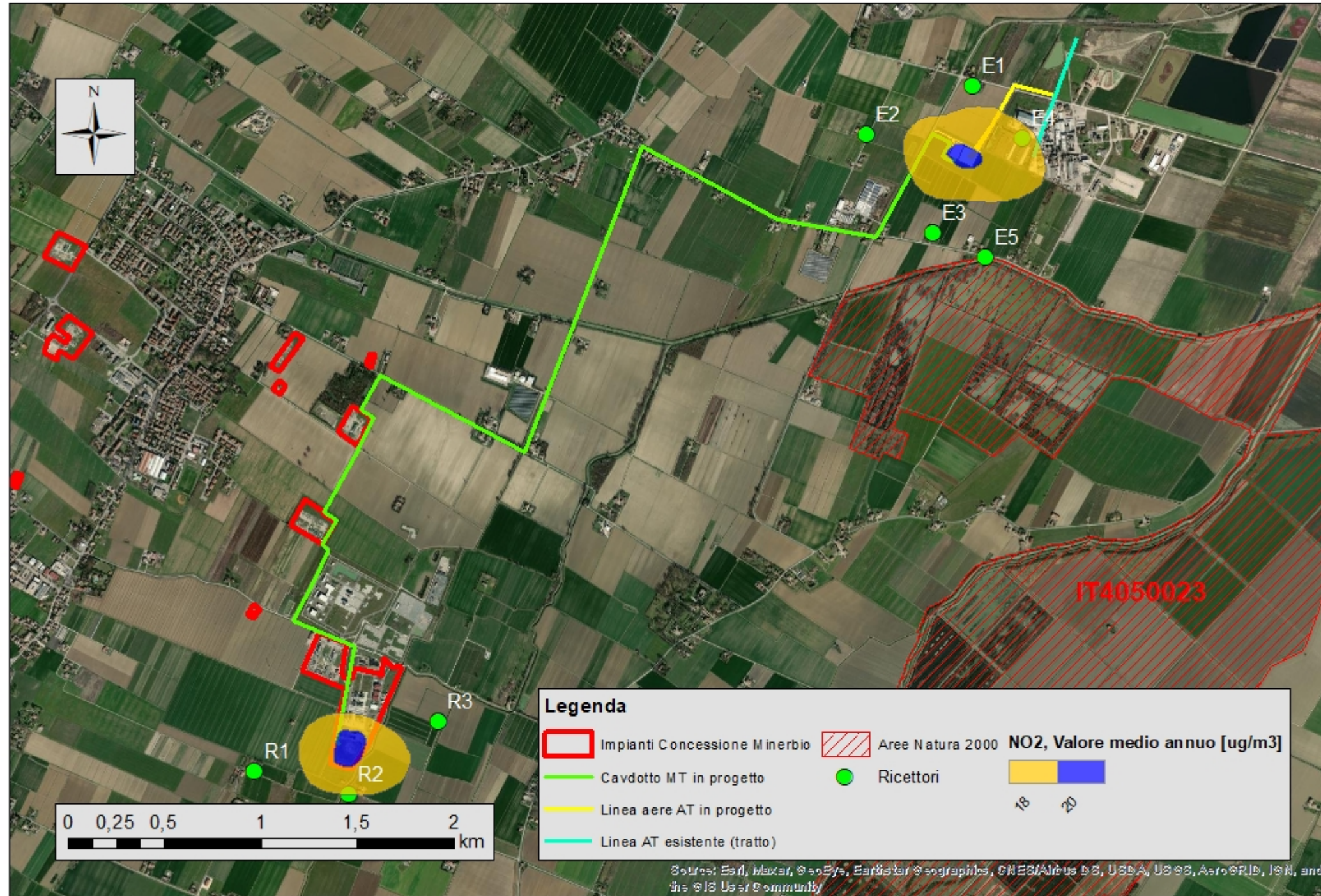
Figura 6.2-1 Biossido di Azoto. Valore medio annuo (V.L. 40 \mu\text{g}/\text{m}^3 , D.Lgs. 155/10 e ss.mm.ii.). Rappresentazione delle isolinee di concentrazione delle ricadute al suolo totali (concentrazione di fondo pari a 17,7 \mu\text{g}/\text{m}^3 e contributo del cantiere)
