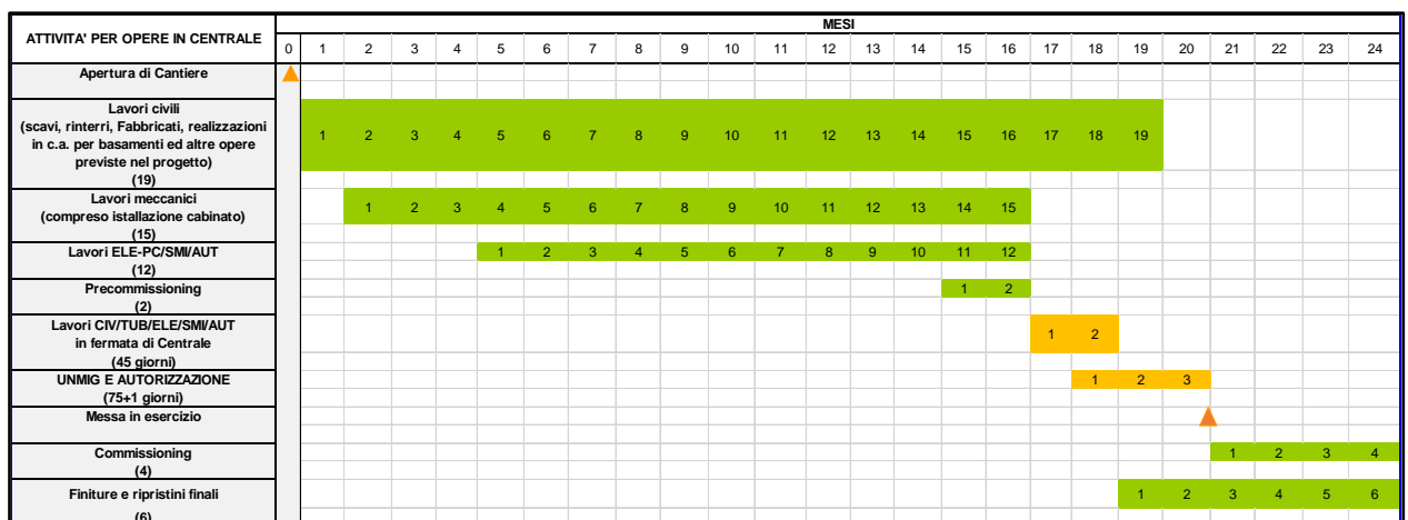
Figura 4.1-1 Cantiere Opere in centrale. Cronoprogramma delle attività previste (in arancione è indicata la Fase 2)
