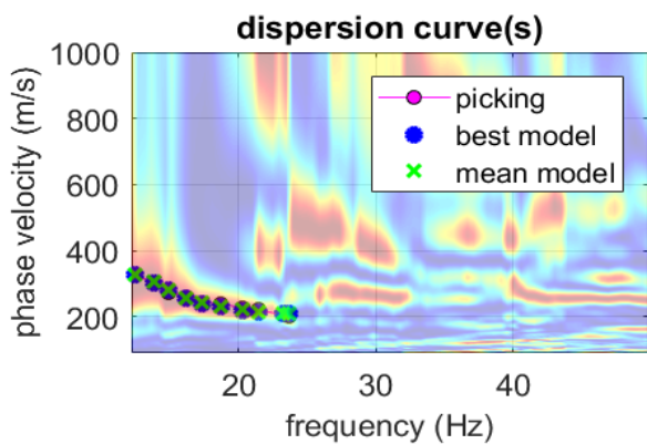
Fig. a - Spettro di velocità base sismica con picking.
