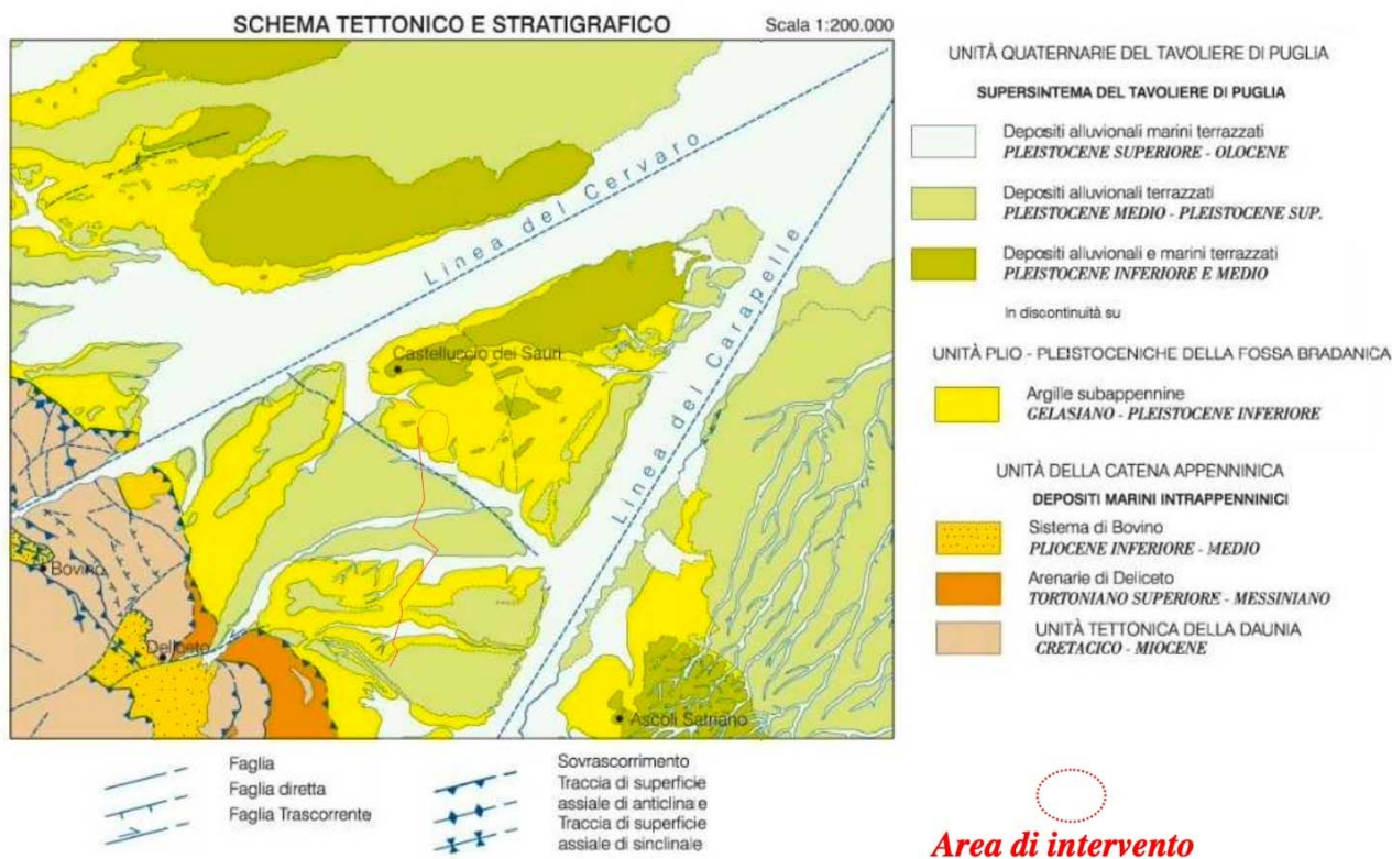
Figura 4 Shema tettonico stratigrafico Progetto CARG. Stralcio della Carta Geologica Foglio 421 Ascoli Satriano - scala 1:50.000
