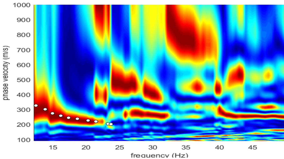
Fig. a - Spettro di velocità base sismica con picking.
