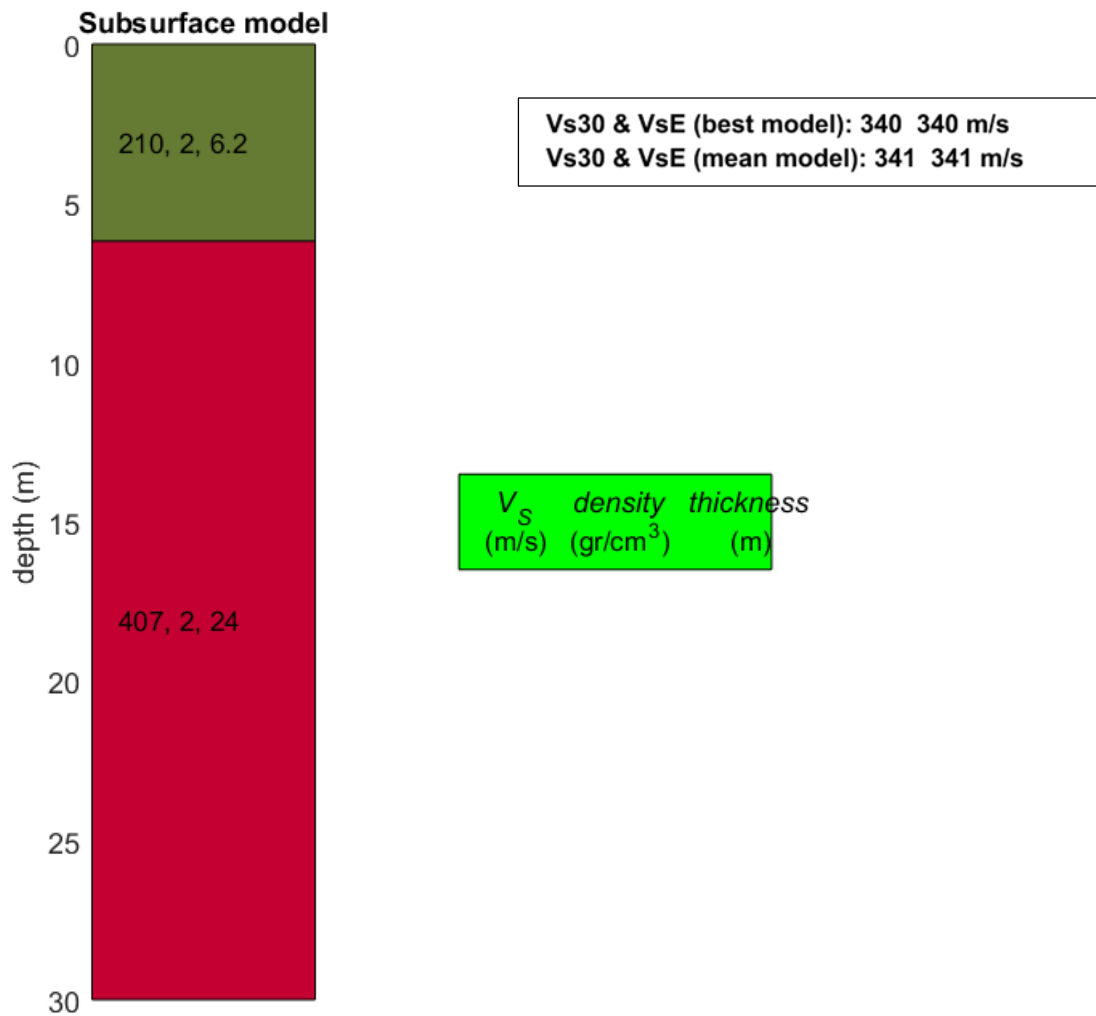
Modello stratigrafico su base sismica
