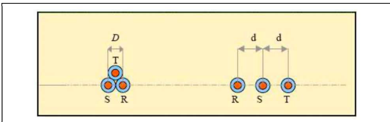
Figura 9-2 Modalità di posa cavo AT
