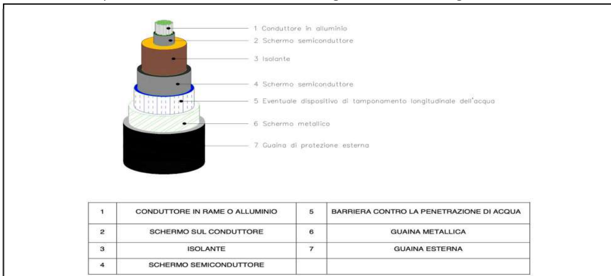
Figura 9-1 Caratteristiche tecniche Cavo AT per trasporto energia
