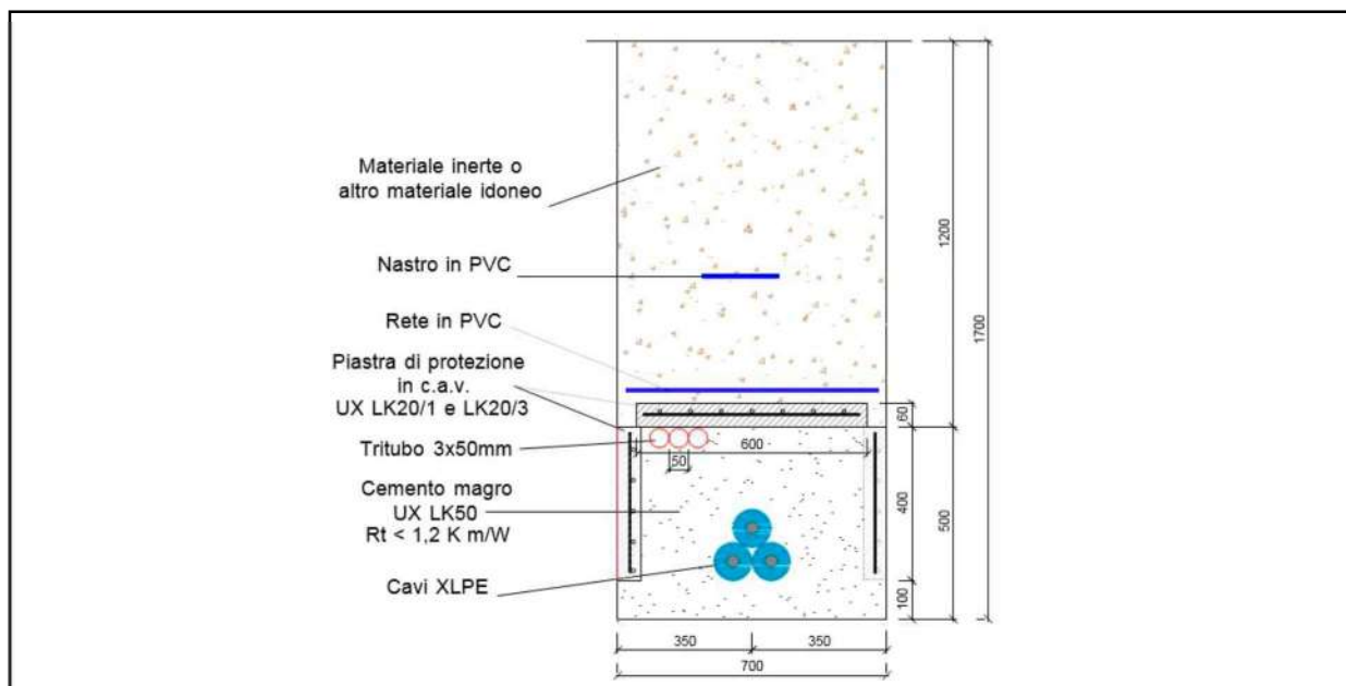
Figura 9-3 Particolare/Posa Cavidotto AT
