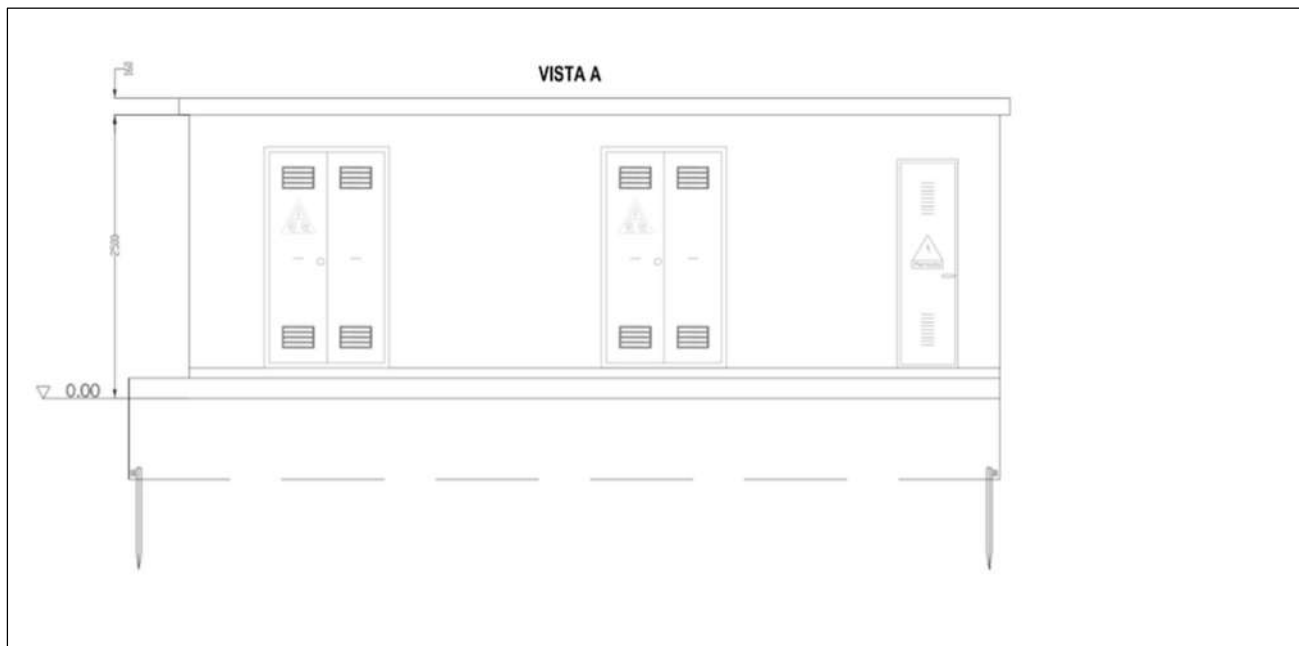
Figura 4-3 Locale cabina di Parallelo MT-Prospecto
