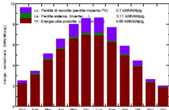
Produzione normalizzata (per kWp installato): Potenza nominale 3088 kWp
