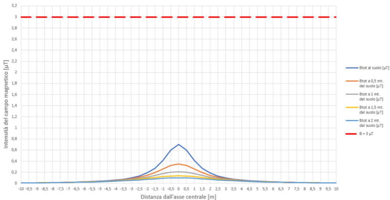
INTESITA' DEL CAMPO MAGNETICO AL VARIARE DELL'ALTEZZA h
