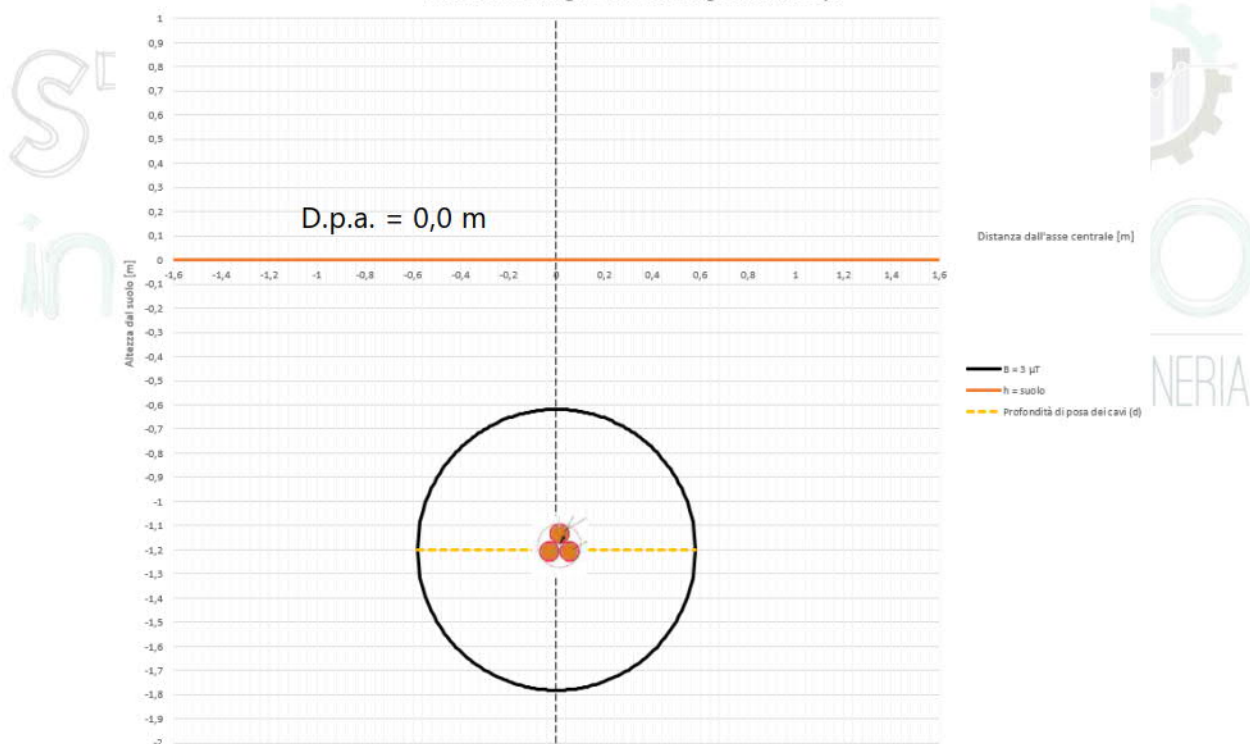
Cavi interrati a trifoglio - Induzione magnetica limite 3 µT
