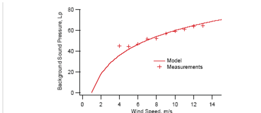
Figura : Confronto tra l'andamento reale del rumore residuo in funzione della velocità del vento e la curva logaritmica che teoricamente descrive meglio tale dipendenza.
