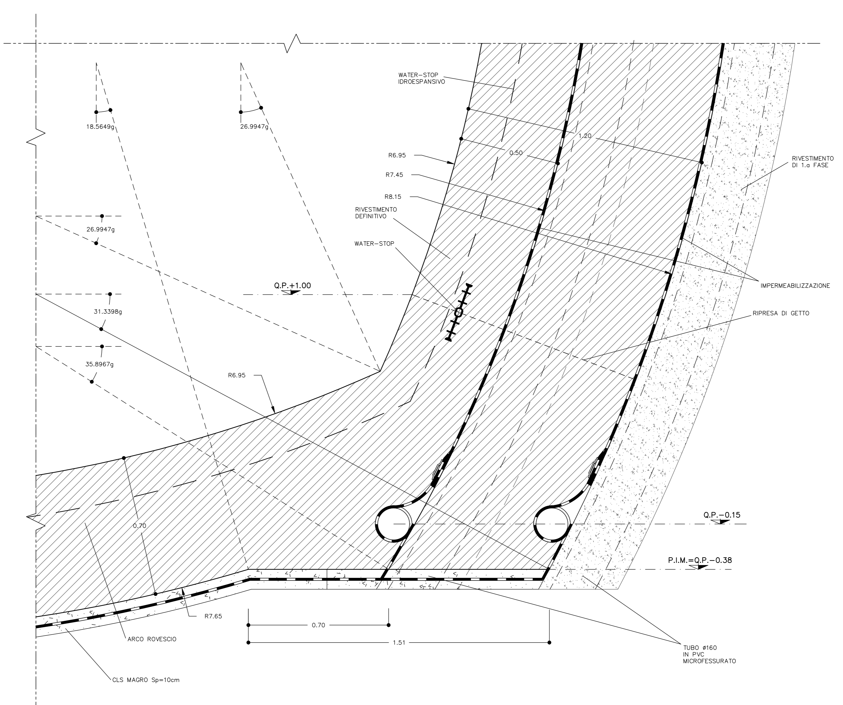
PARTICOLARE MURETTA SCALA 1:10
