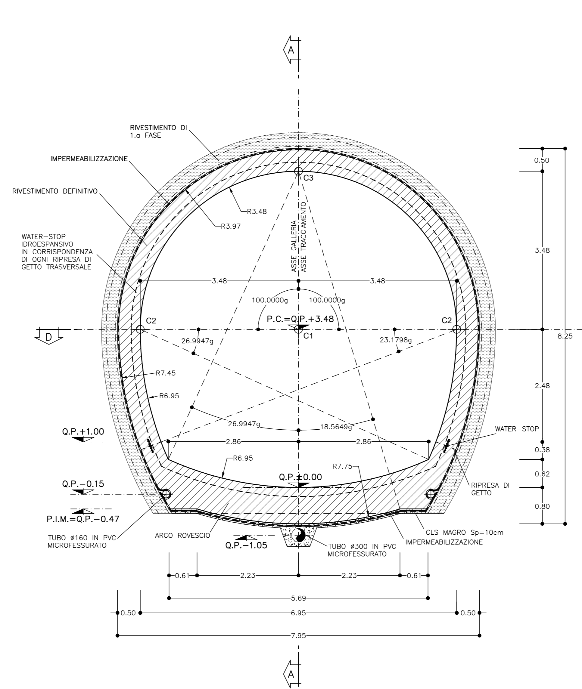
SEZIONE B-B SCALA 1:50 SEZIONE MINIMA
