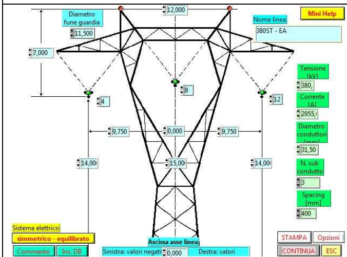
Configurazione 380 ST – Tipo EA
