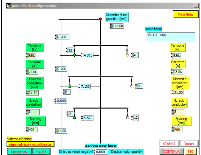
Configurazione 380 DT – Tipo M e Tipo N
