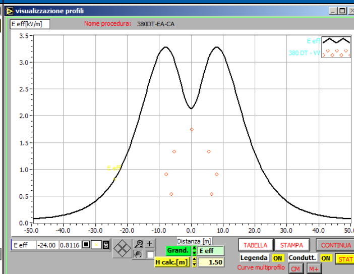
Campo elettrico inferiore a 3.4kV/m
