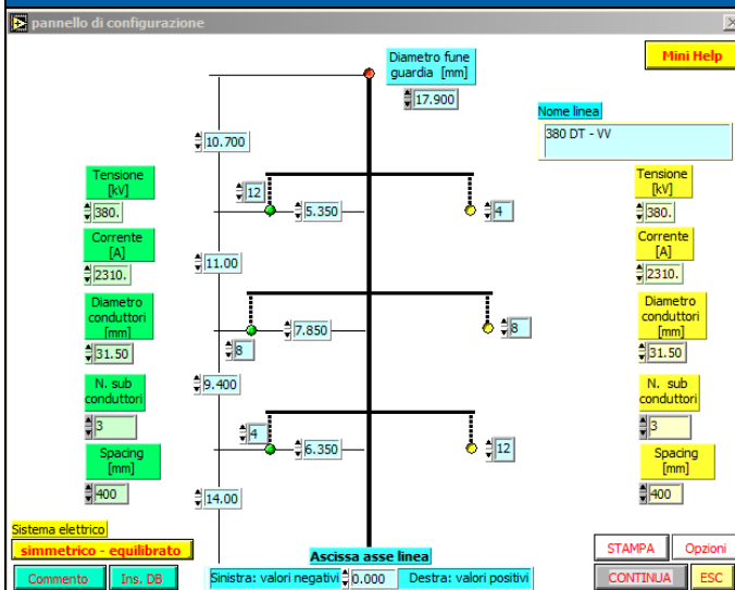
Configurazione 380 DT – Tipo VV
