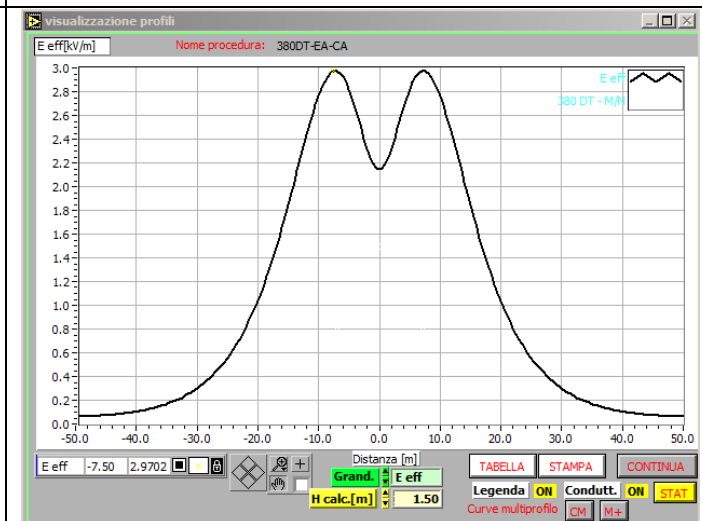
Campo elettrico inferiore a 3kV/m
