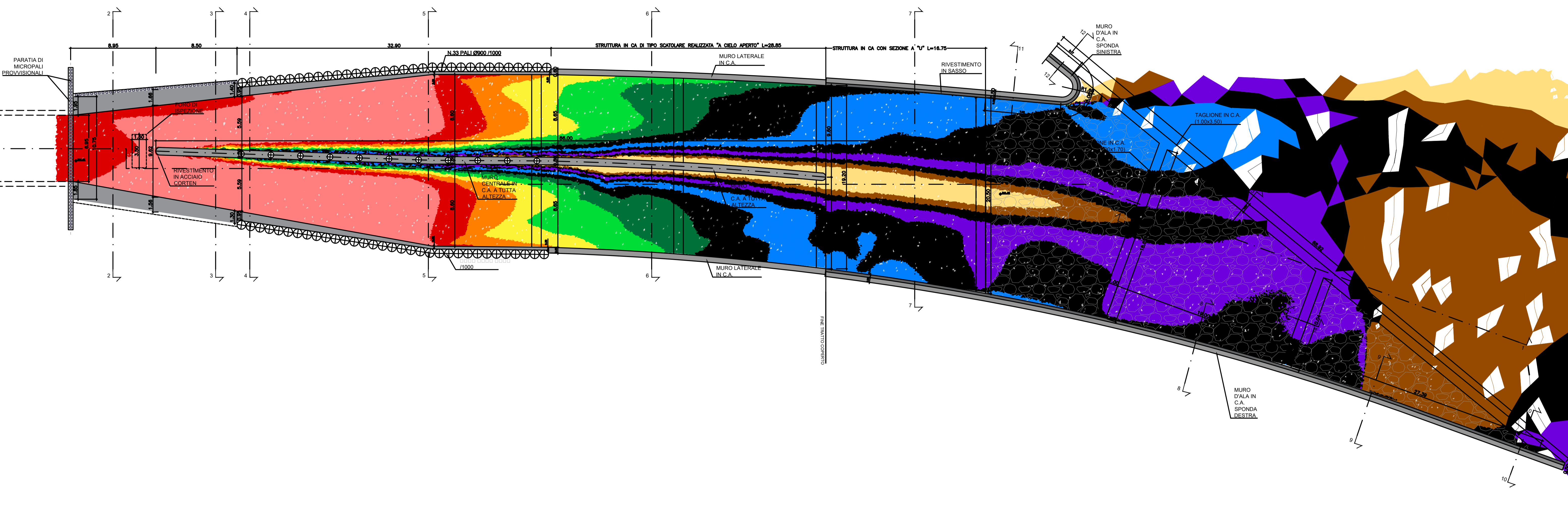
PIANTA SBOCCO - VELOCITA' Qgalleria=330 mc/s - Scala 1:200
