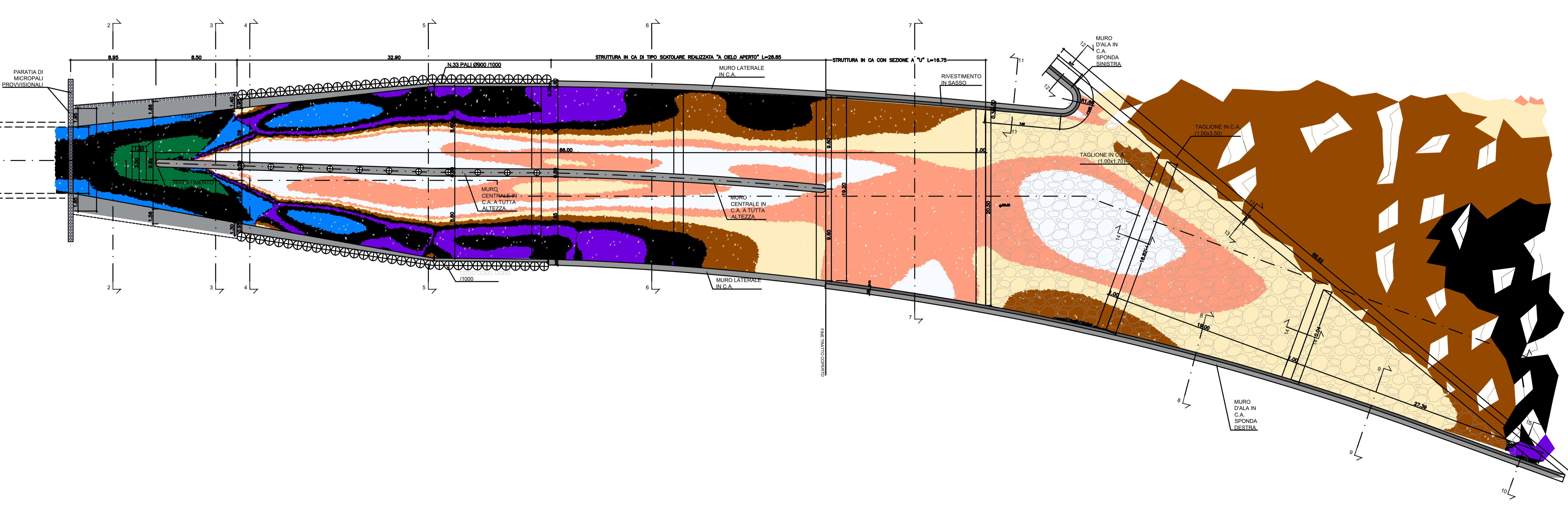
PIANTA SBOCCO - VELOCITA' Qchiese=220mc/s e Qgalleria 110mc/s - Scala 1:200
