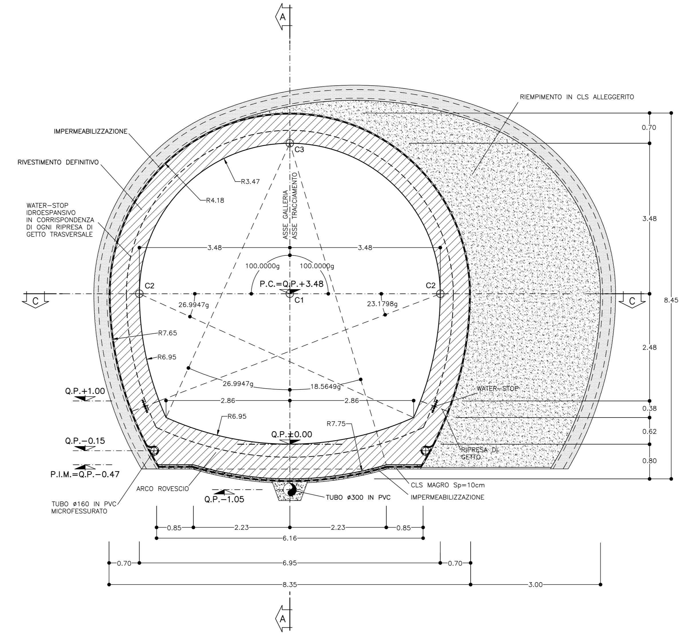
SEZIONE B-B SCALA 1:50 SEZIONE TRASVERSALE
