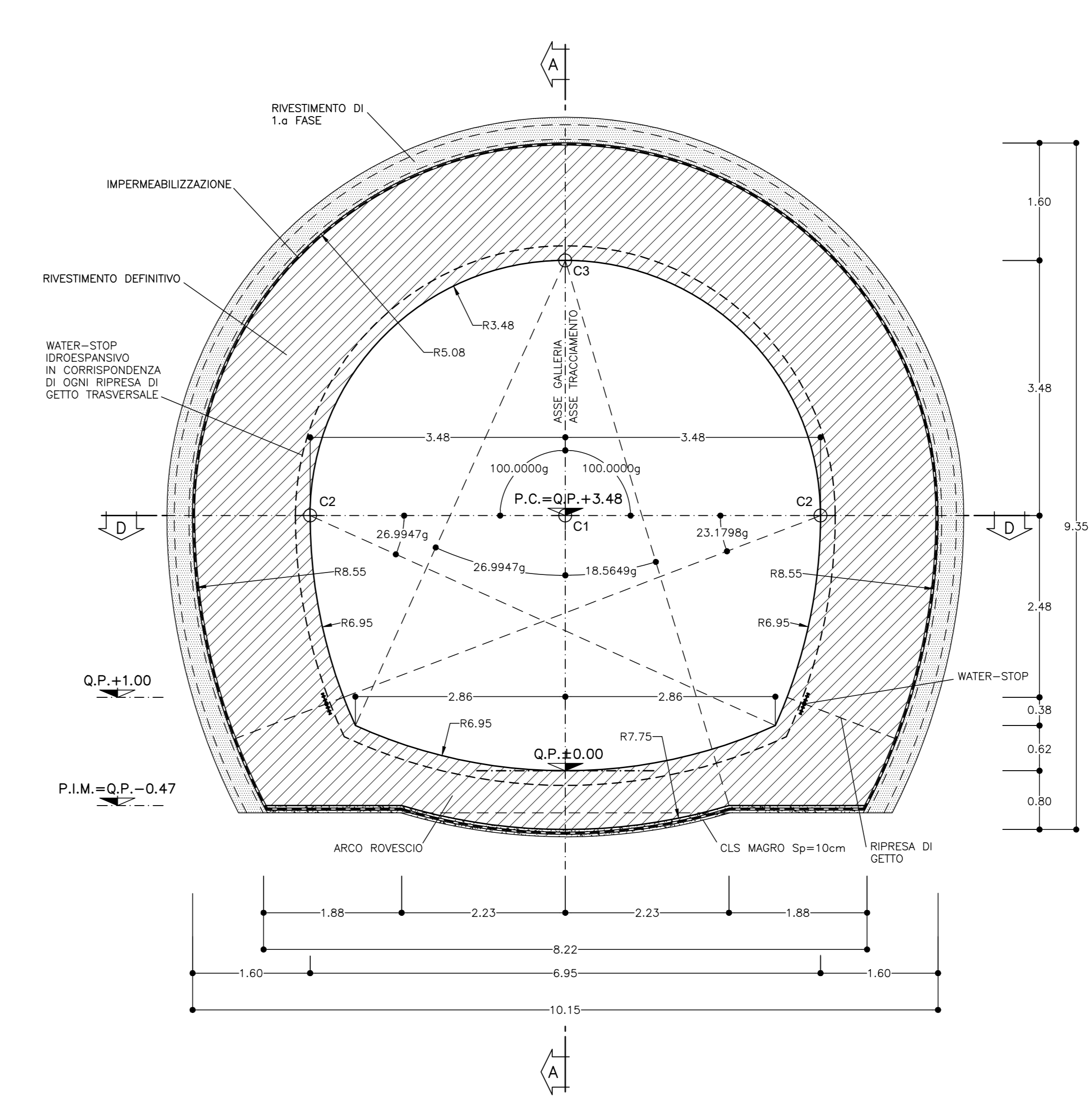
SEZIONE C-C SCALA 1:50 SEZIONE MASSIMA
