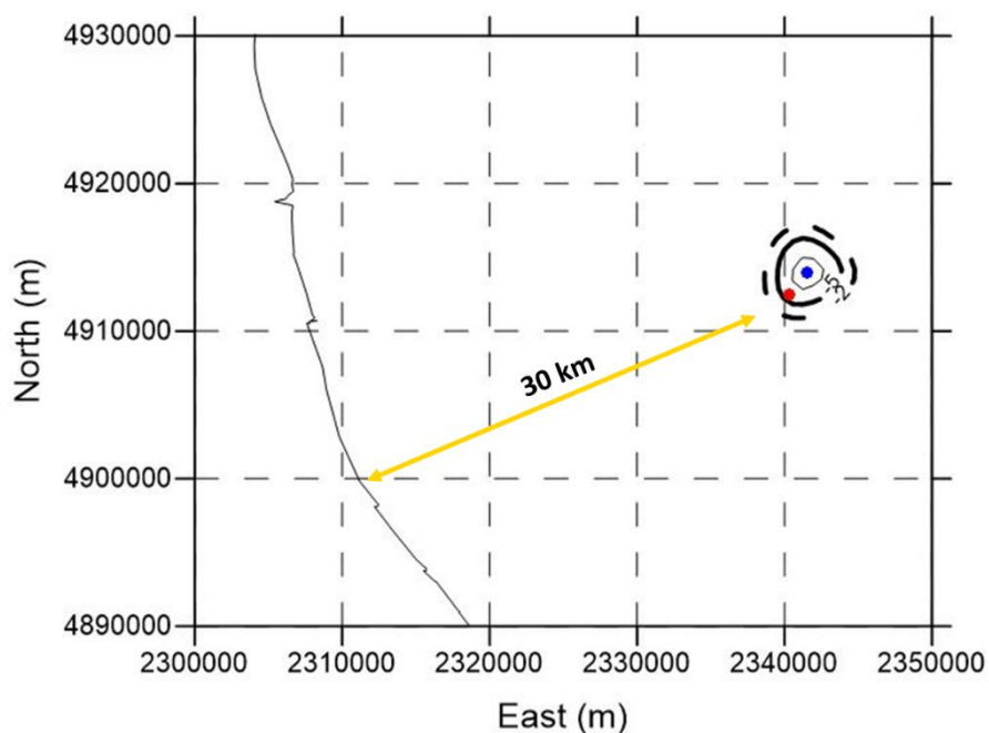
Figura 8 – Curve di iso-subsidenza per lo scenario “Do Nothing - caso base” a fine produzione. In blu è riportata la posizione del punto di massimo, in rosso la posizione della piattaforma.
