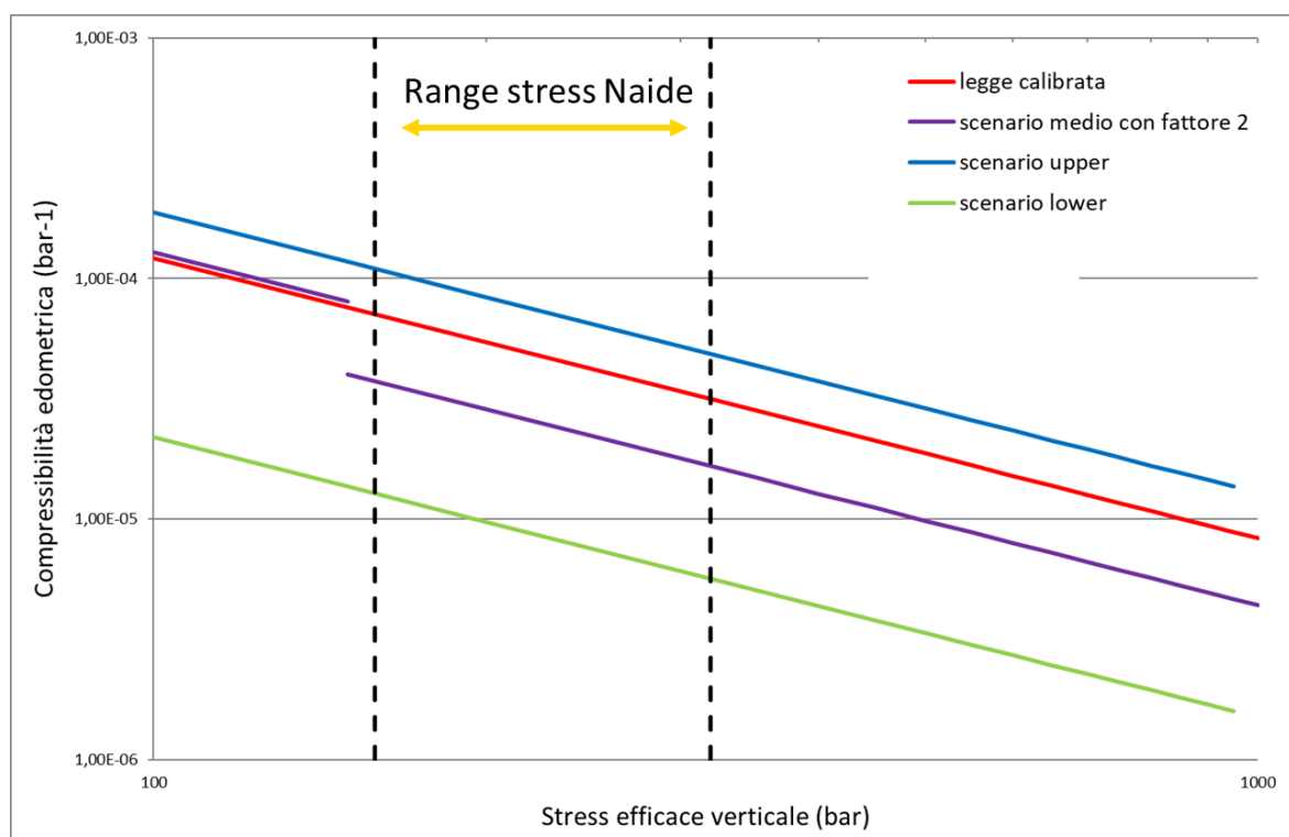
Figura 5 – Legge di variazione della compressibilità edometrica calibrata per il campo di Naide.
