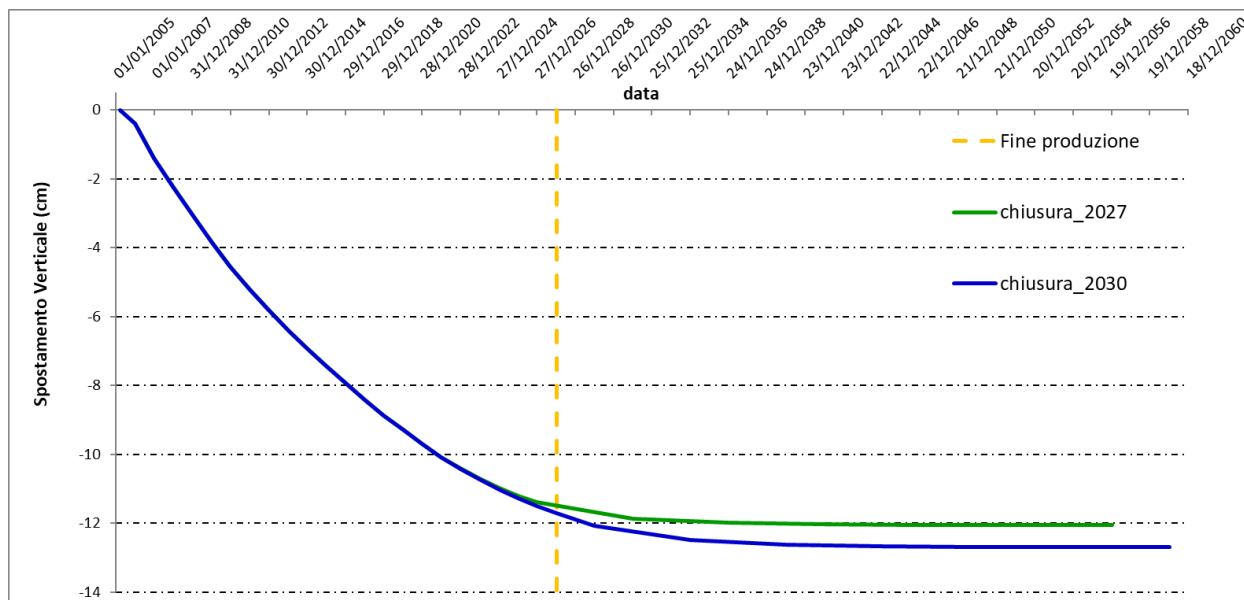
Figura 7 – Evoluzione nel tempo del valore di subsidenza nel punto di massimo.
