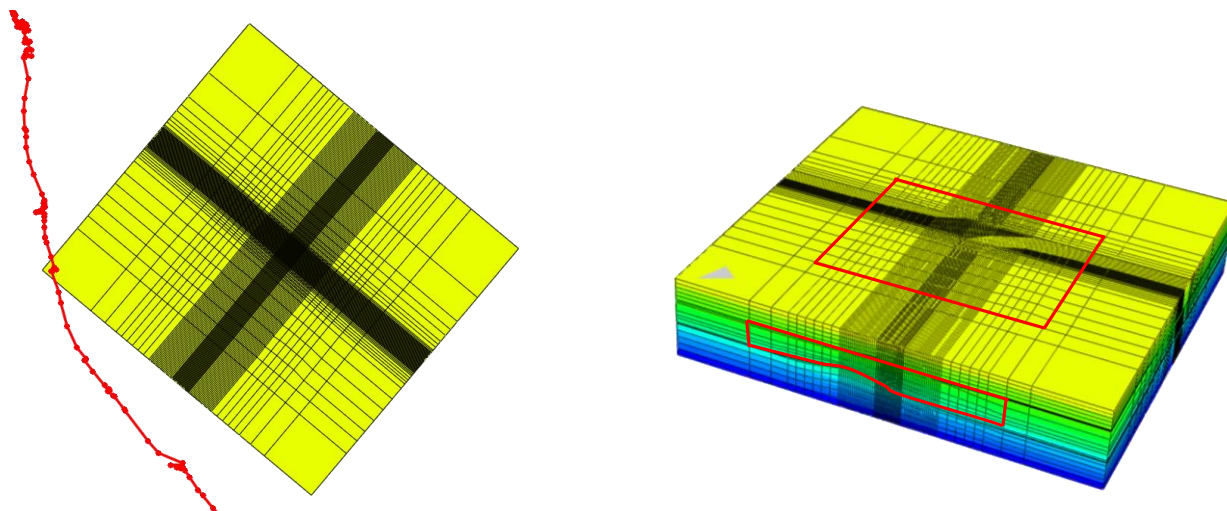
Figura 3 – Confronto tra l'estensione del modello geomeccanico e del modello dinamico (rosso). A sinistra è evidenziata la linea di costa.
