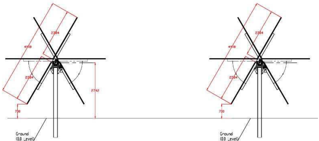
Figura 4.2: Sezione trasversale tracker
