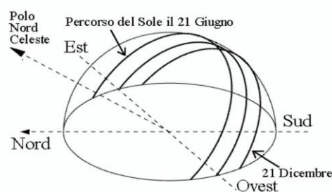
Fig. 1 - Movimento apparente del disco solare per un osservatore situato ad una latitudine nord attorno ai 45°. Per tutte le località situate tra il Tropico del Cancro e il Polo Nord Geografico il disco solare non raggiunge mai lo zenit.
