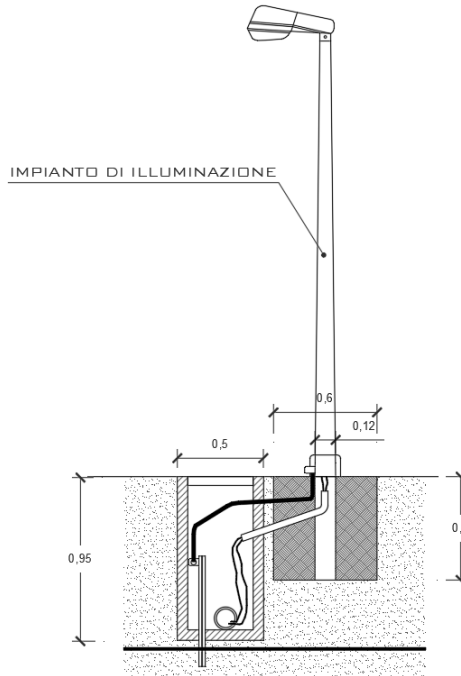
Fig. 3 - Tipologia di corpi illuminanti - perimetro impianto
