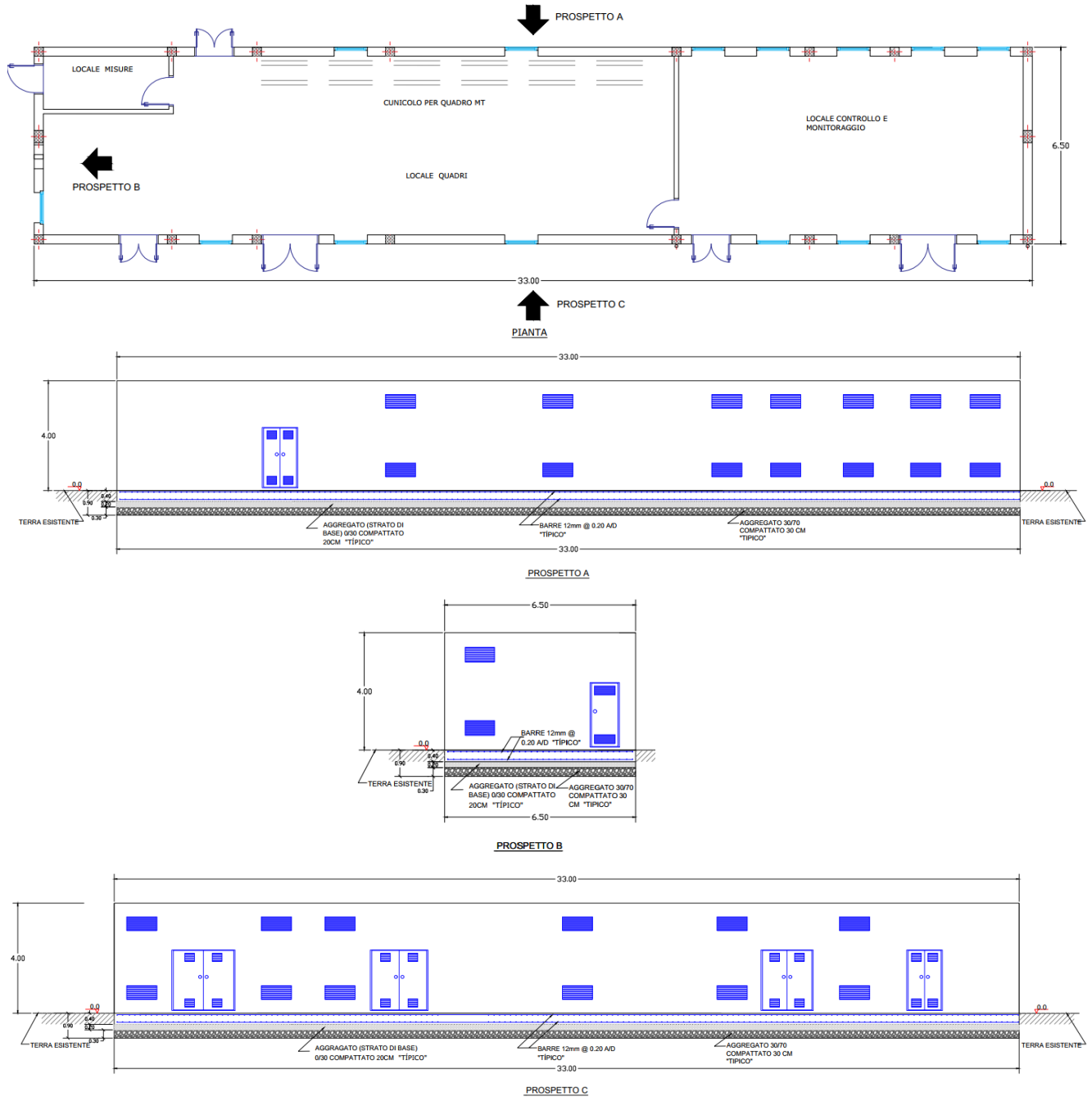
Fig. 15 - Cabina di ricezione
