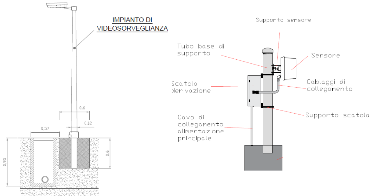
Fig. 19 – Sistema antintrusione
