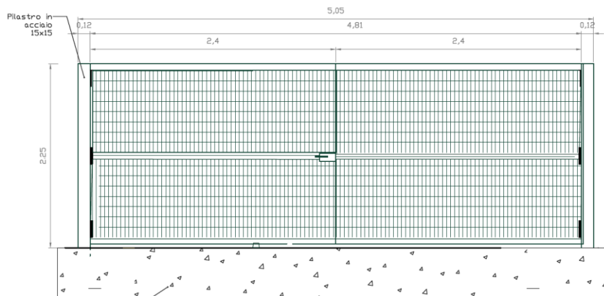
Fig. 17 – Cannello carrabile
