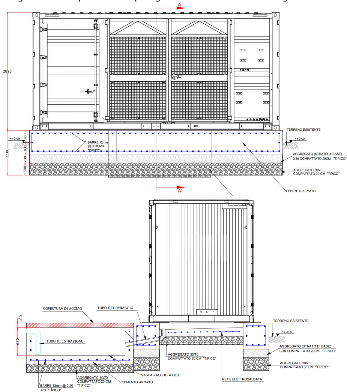
Fig.14 – Cabina di trasformazione BT/MT
