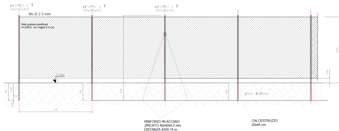
Fig. 16 – Particolare della recinzione
