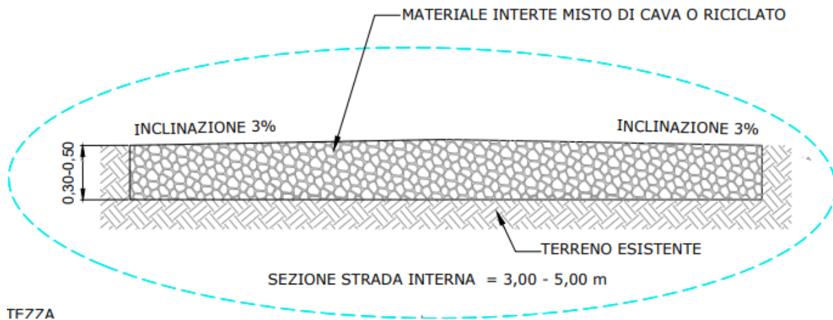
Fig. 18 – Sezione strada perimetrale
