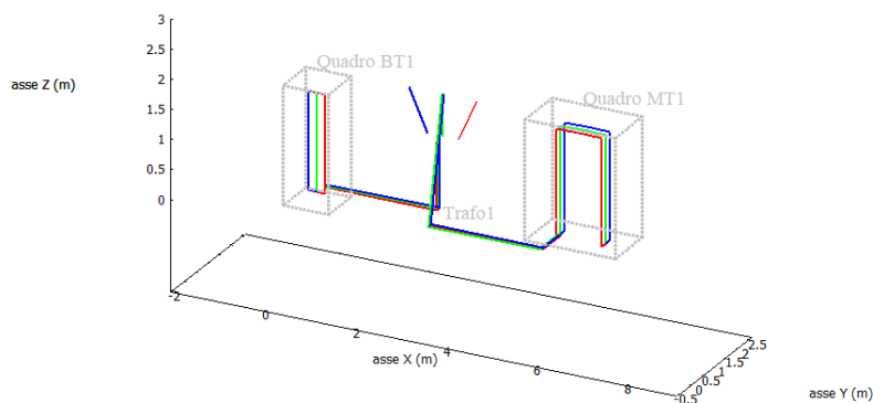
Fig.6 - Modello spaziale cablaggi nelle cabine di trasformazione MT/BT
