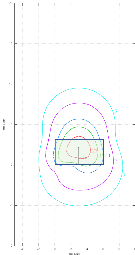
Cabina - calcolo su piano xz - quote Y=-1 m
