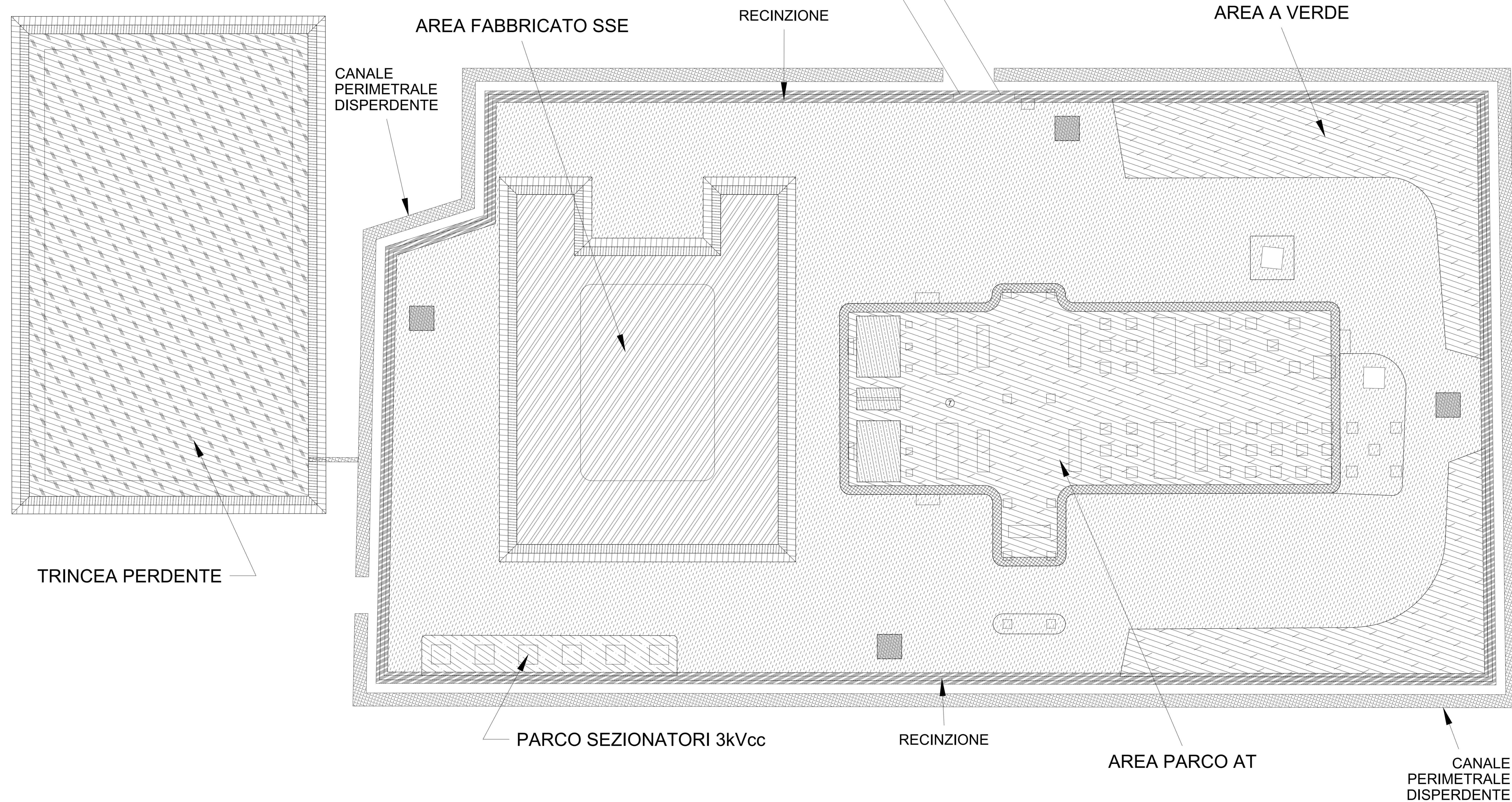
1 Piazzale di SSE - Pianta scavi 1 : 200
