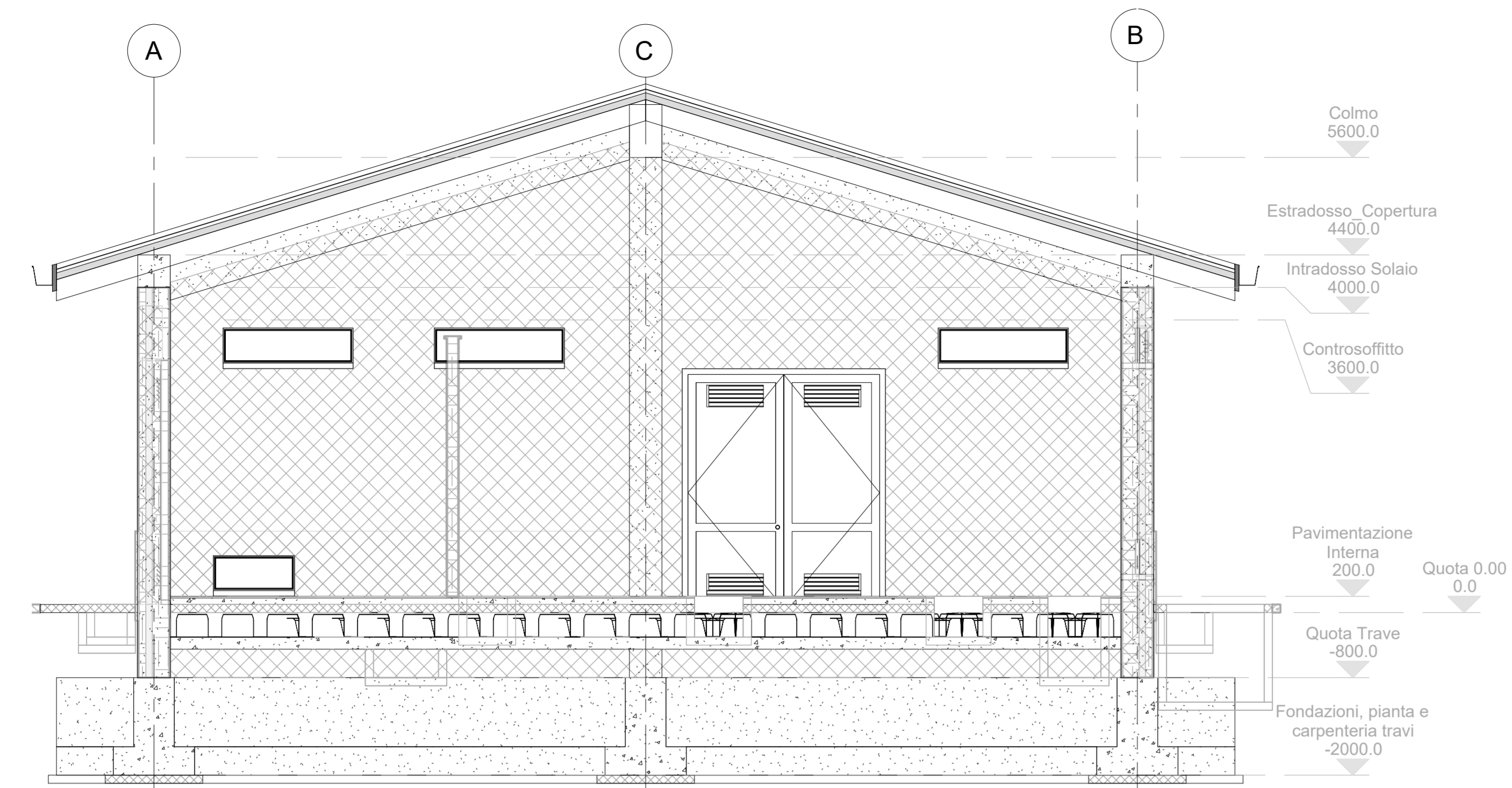
5 Arc.3 1:50
