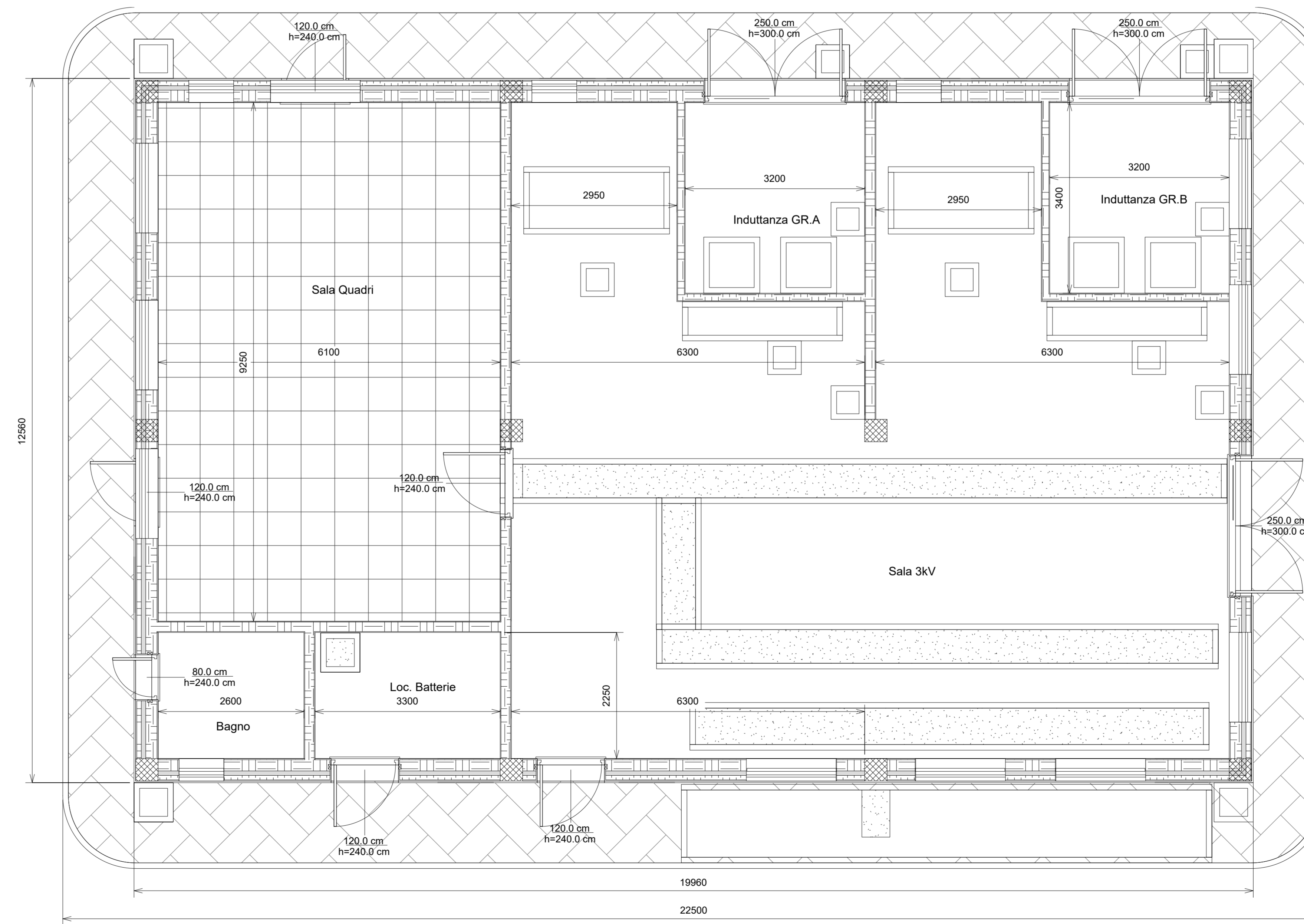
1 Pianta piano Terra 1:50
