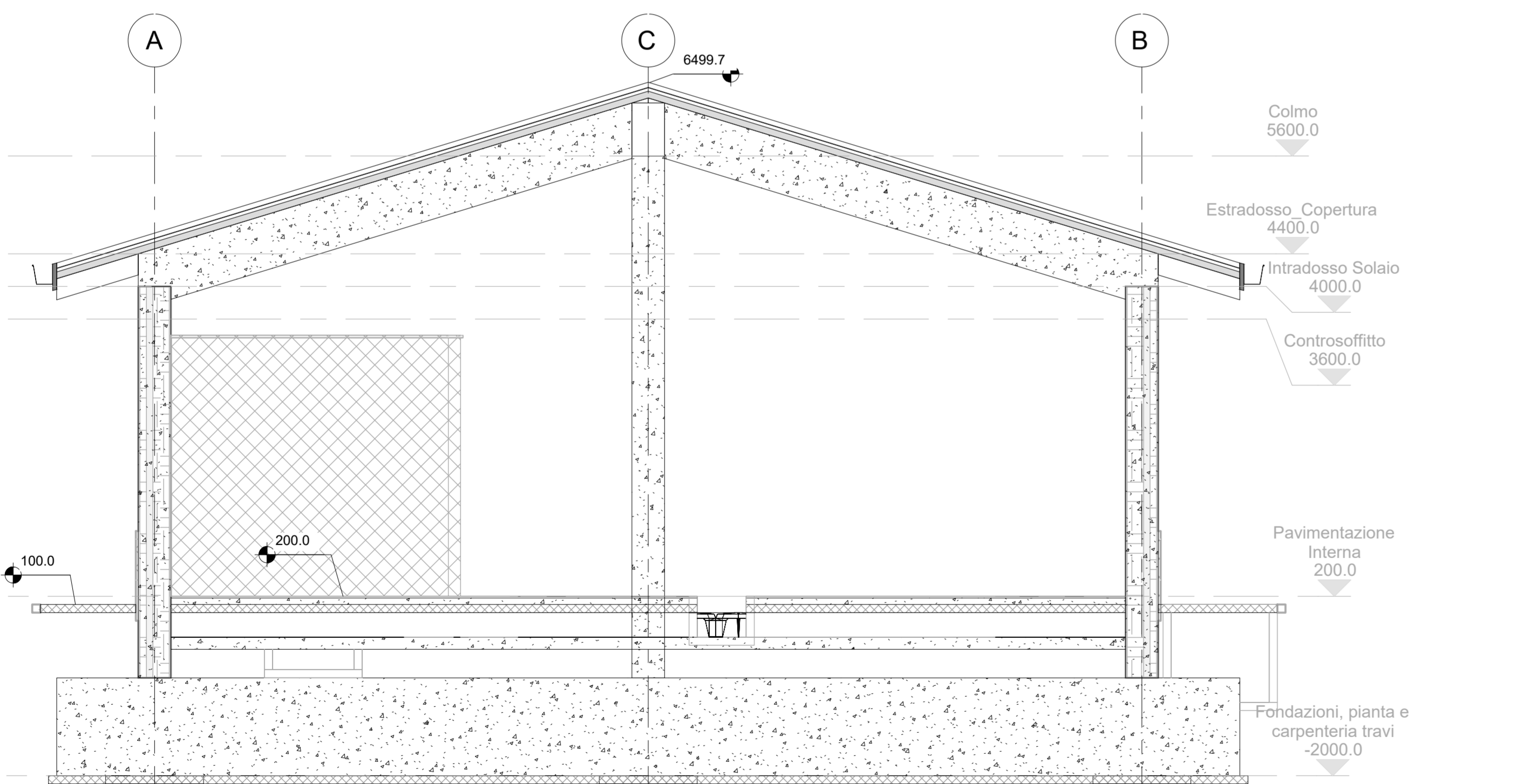
4 Arc.2 1:50
